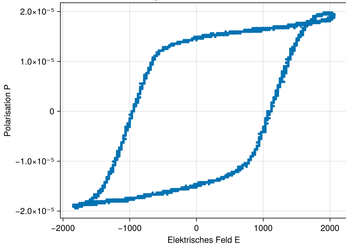
Hysterese bei 4V und 30 Hz
