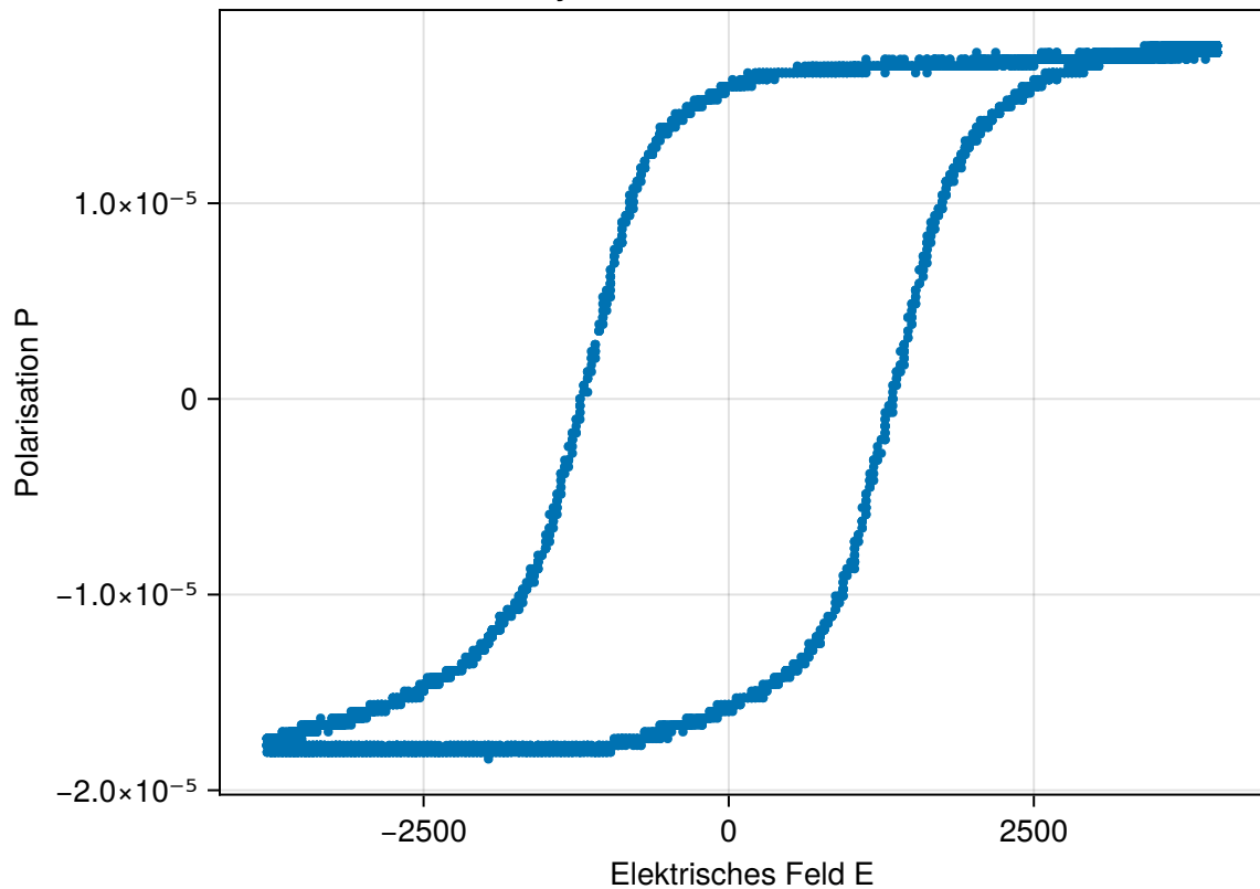
Hysteresese bei 8V und 110 Hz
