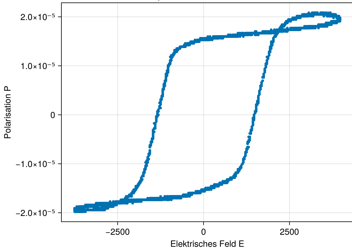
Hysteresese bei 8V und 30 Hz
