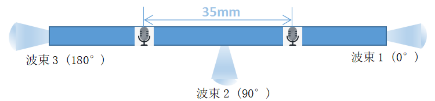
图 1 2mic线型三波束阵列示意图
