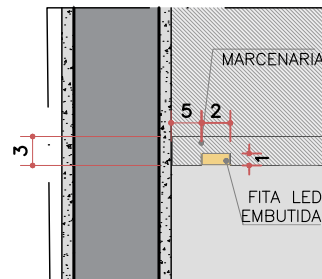
DET.2 FITA LED (SEM ESCALA)
