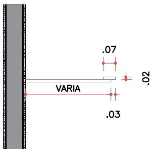
SEÇÃO ÁREA MOLHADA ESC. 1:25
