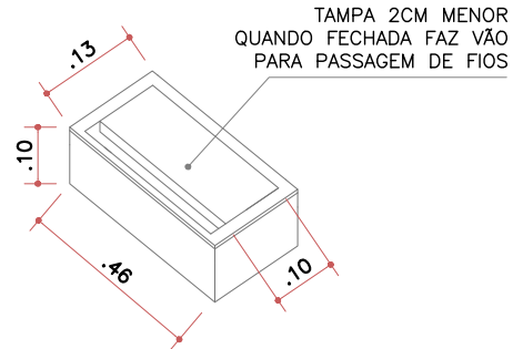
DET.9. CAIXA TOMADAS S/ ESCALA
