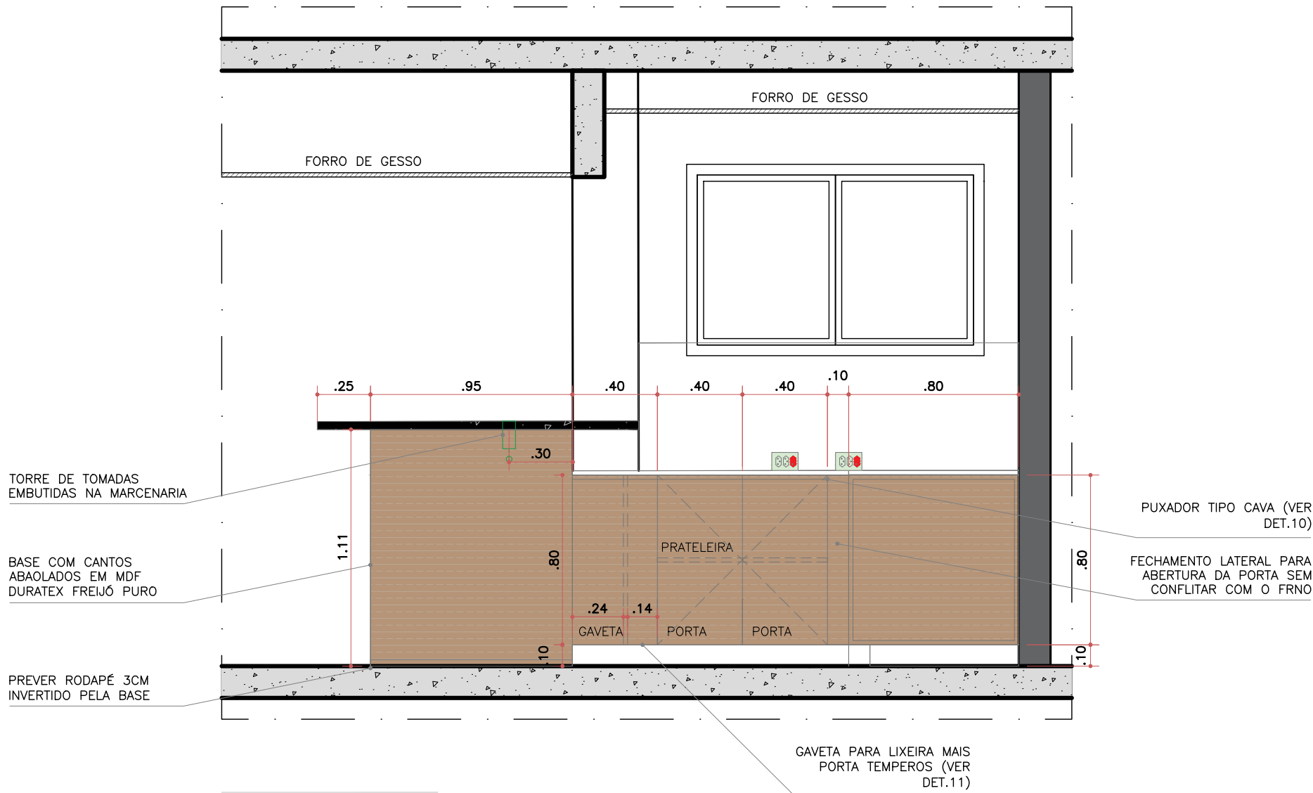
VISTA 02 COZINHA ESC. 1:25
