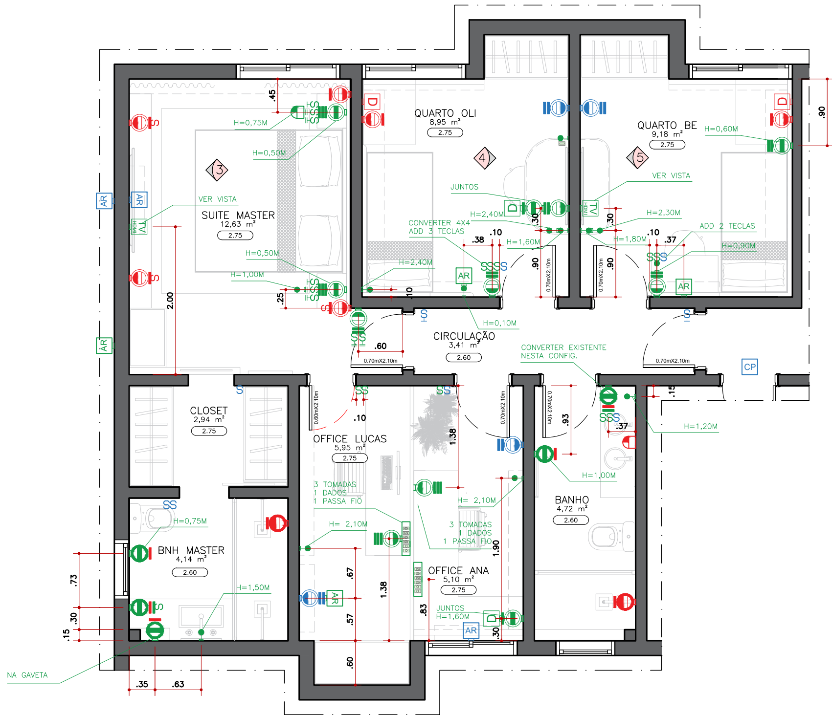
PLANTA BAIXA SECÇÃO 01 ESC. 1:50
