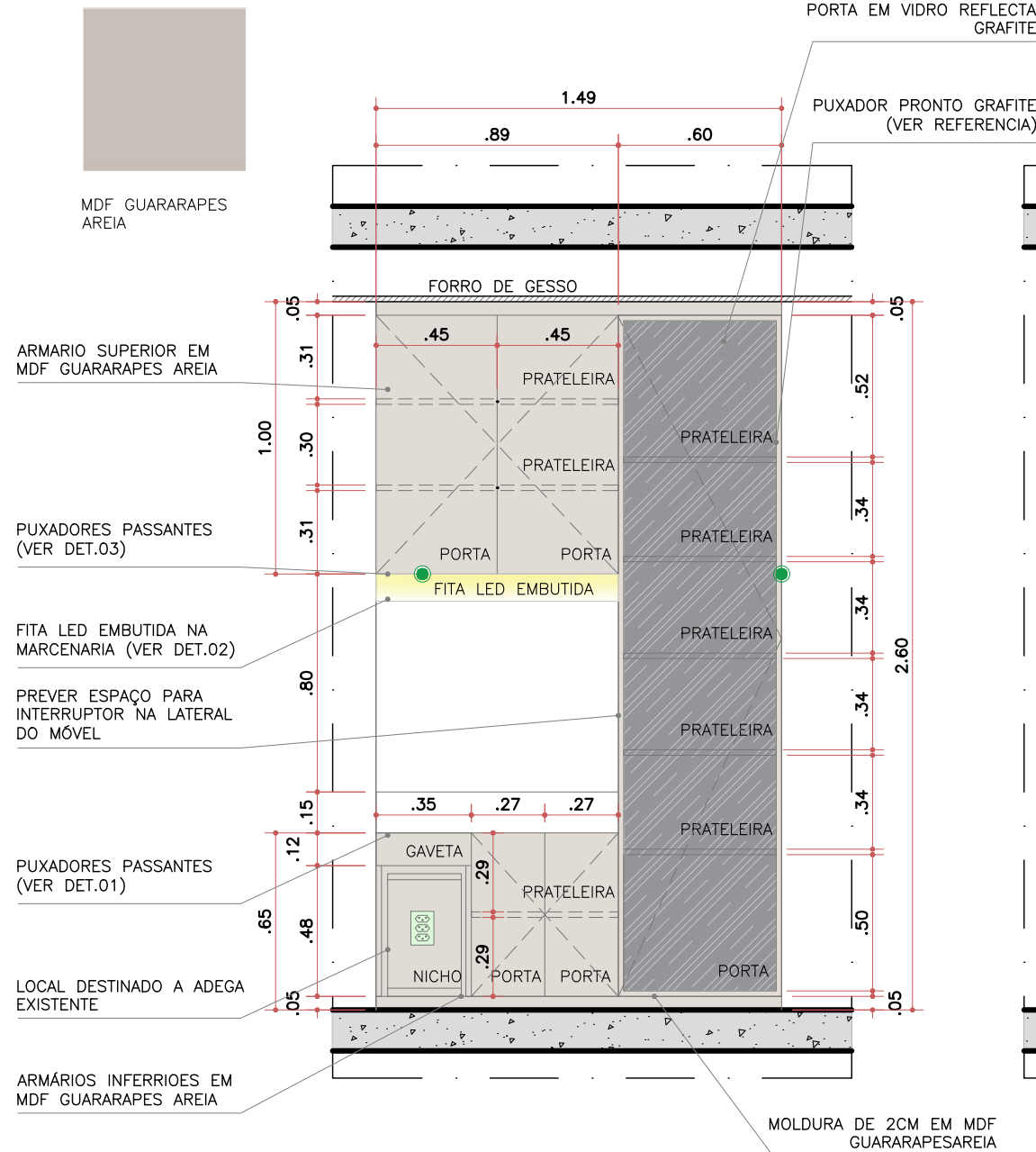
VISTA 01 LIVING – JANTAR ESC. 1:25
