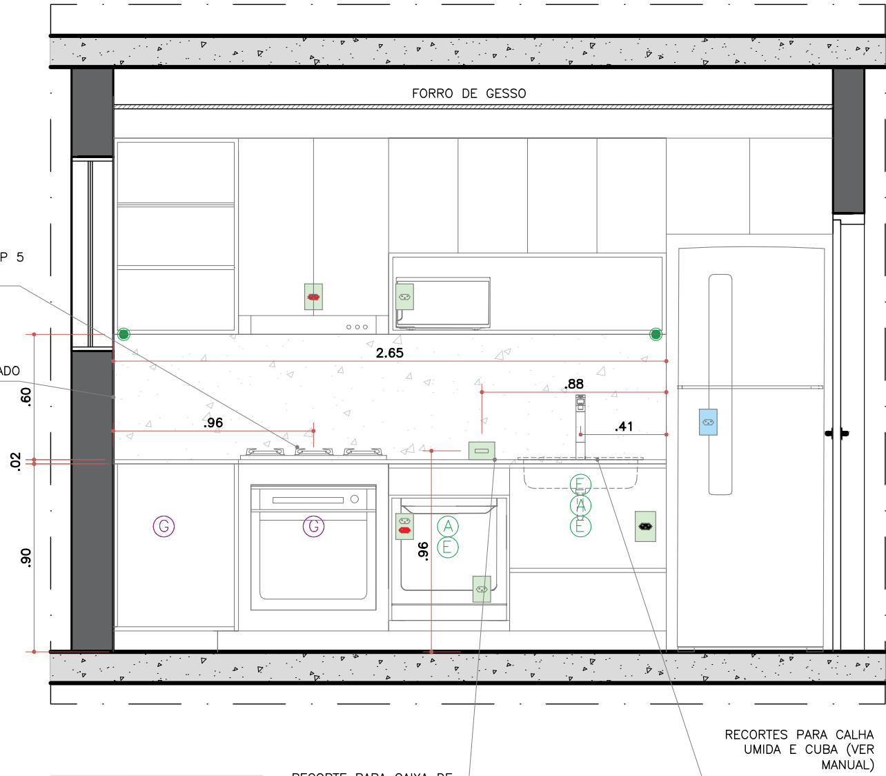
VISTA 01 COZINHA ESC. 1:25
