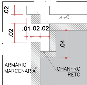
DET.10 CAVA RETA (SEM ESCALA)
