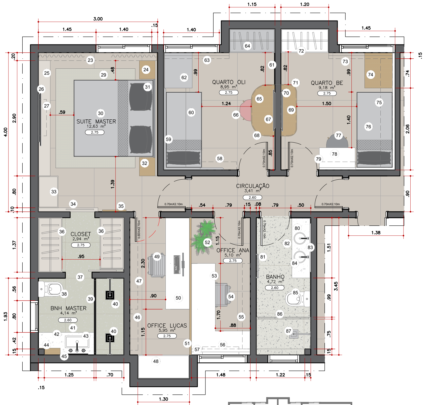
PLANTA BAIXA SECÇÃO 02 ESC. 1:50
