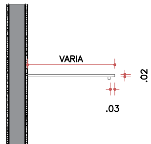
SEÇÃO ÁREA SECA ESC. 1:25
