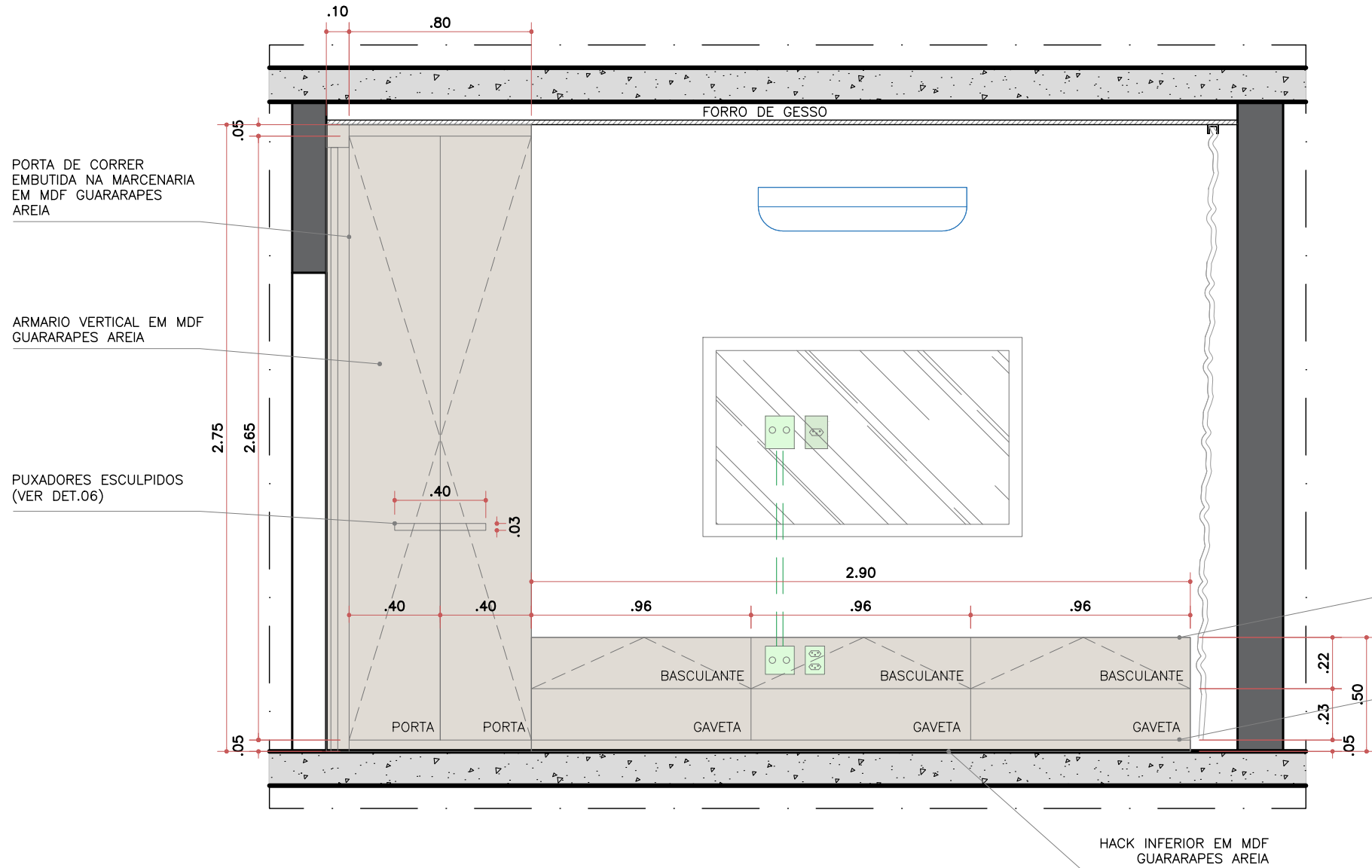
VISTA 01 SUITE MASTER ESC. 1:25
