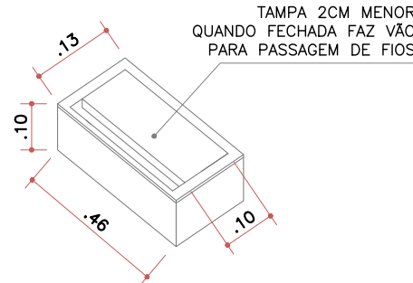
DET9. CAIXA TOMADAS S/ ESCALA
