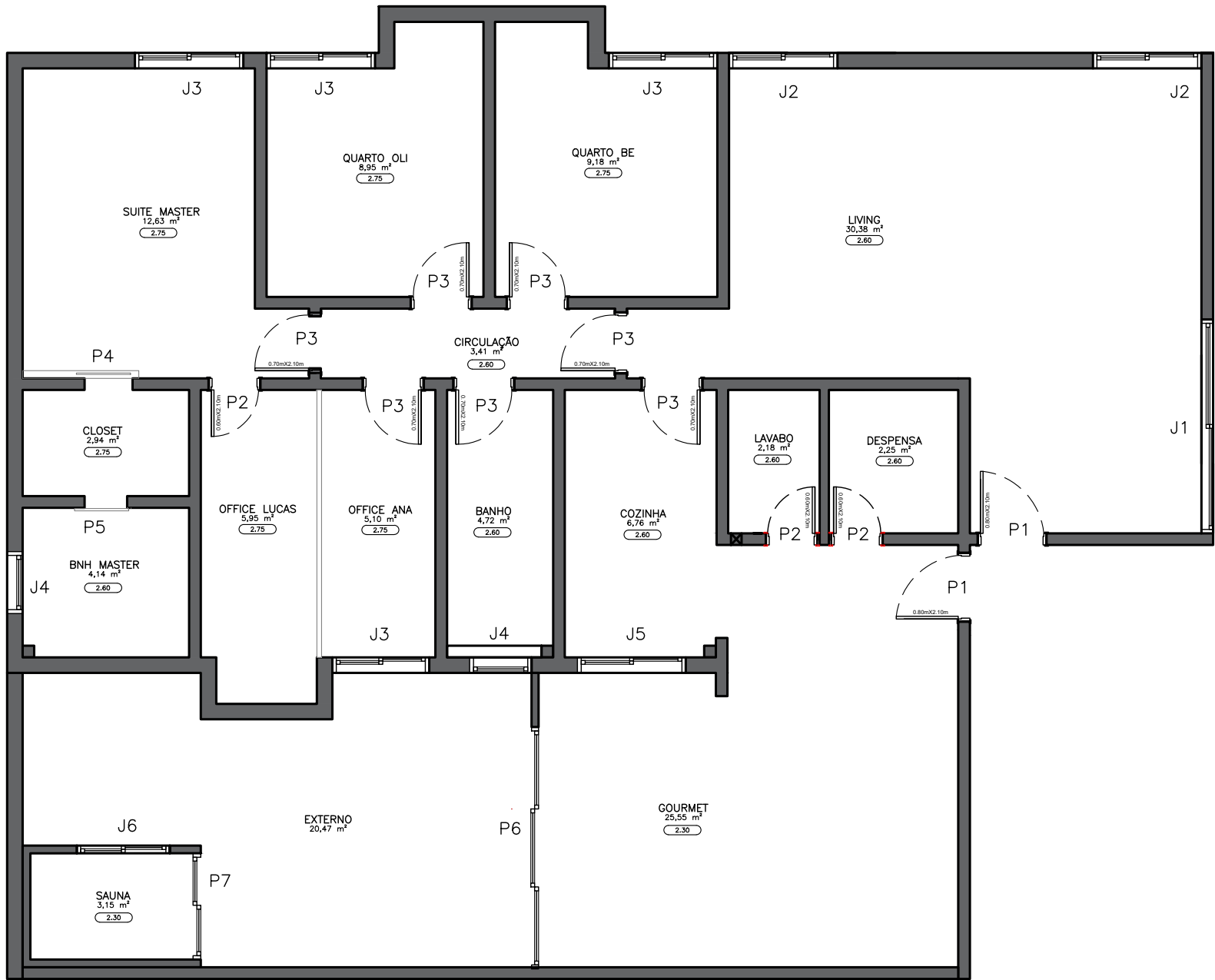
PLANTA BAIXA APTO 101 ESC. 1:75
