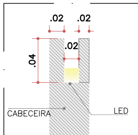
DET. 05 PUXADOR (SEM ESCALA)
