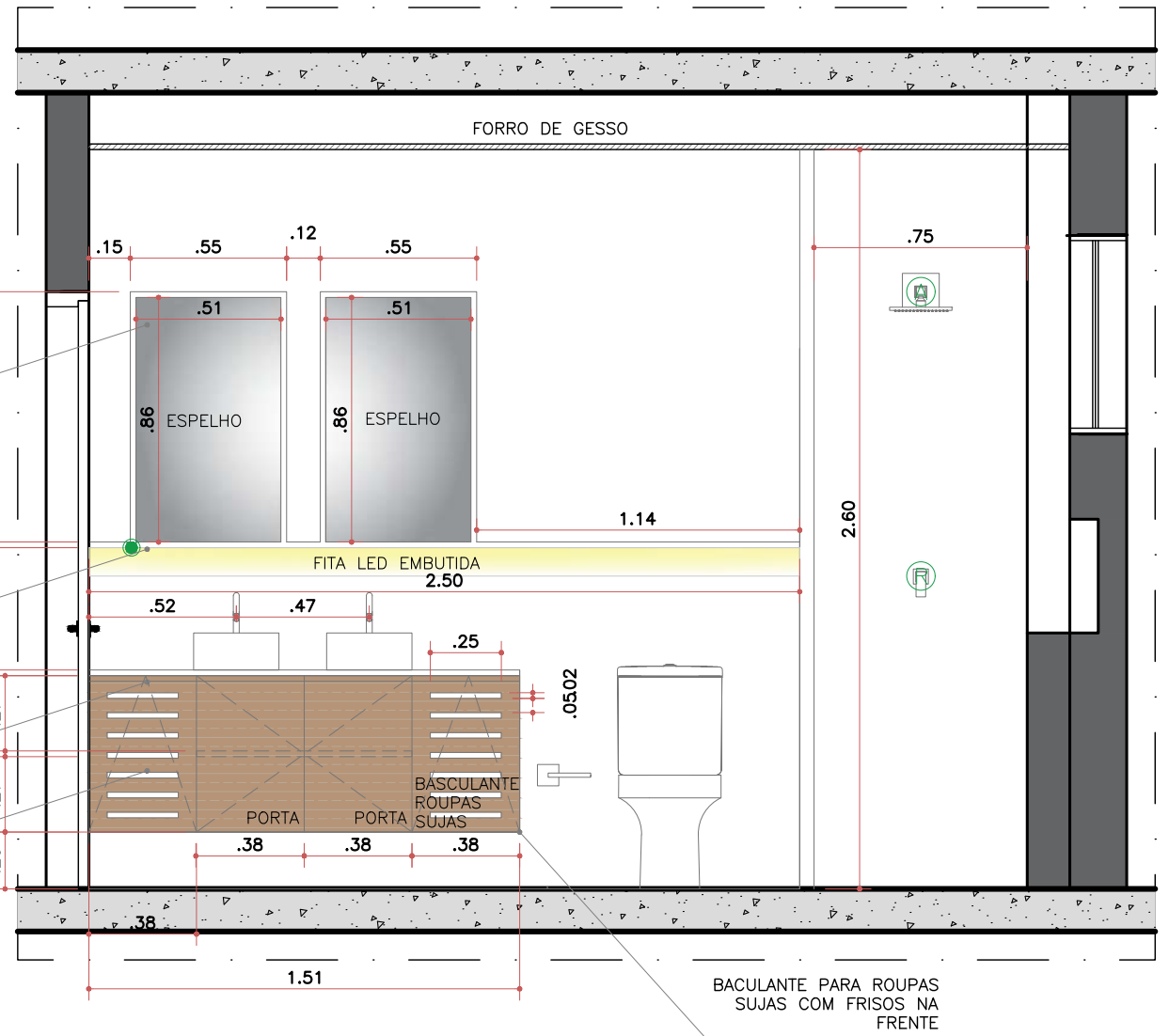
VISTA 01 BANHO ESC. 1:25
