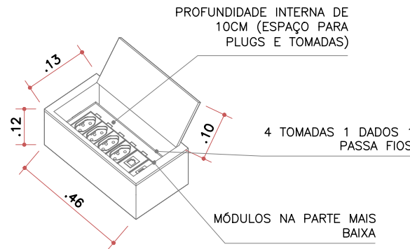
DET.9 CAIXA TOMADAS S/ ESCALA
