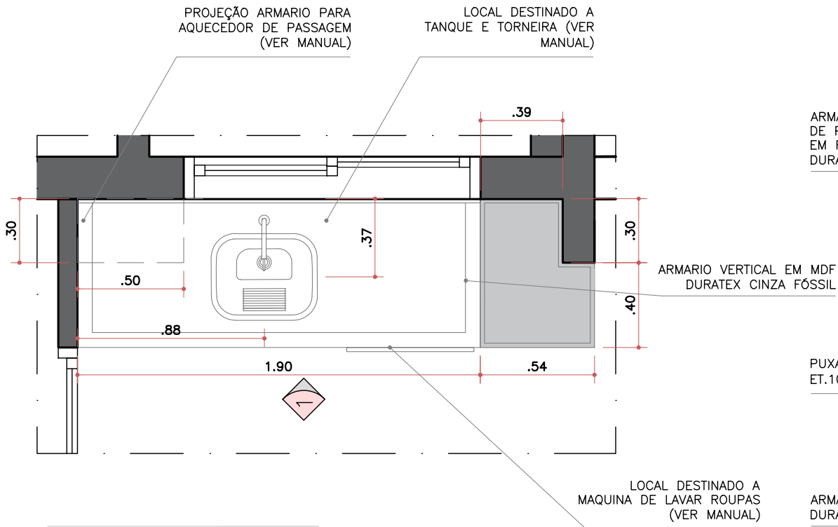
PLANTA AREA DE SERVIÇO ESC. 1:25
