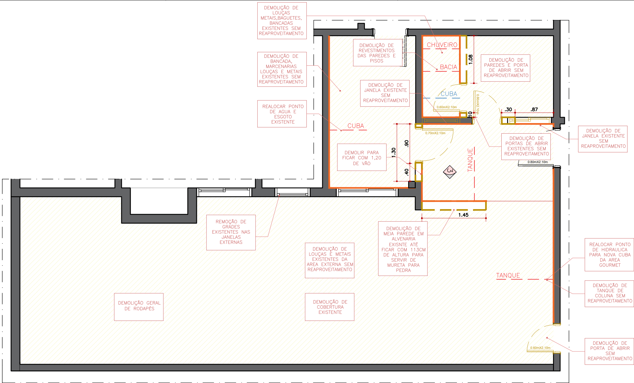
PLANTA BAIXA SECÇÃO 02 ESC. 1:50
