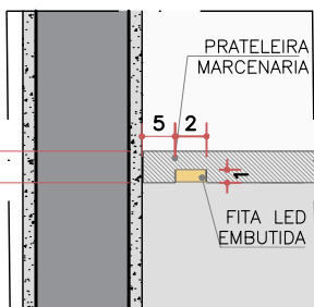
DET.6 FITA LED (SEM ESCALA)
