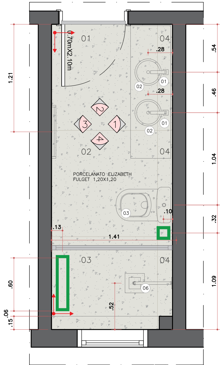
PLANTA BANHO ESC. 1:25
