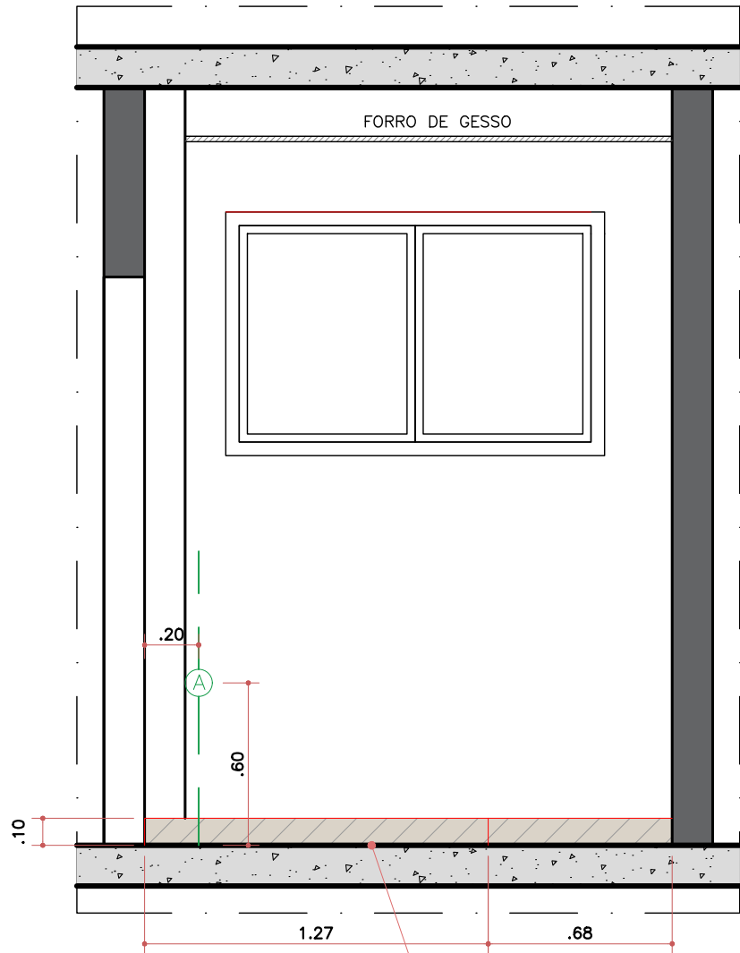
VISTA 03 COZINHA ESC. 1:25
