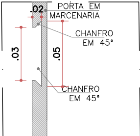
DET.06 PUXADOR CAVA (SEM ESCALA) EM PLANTA
