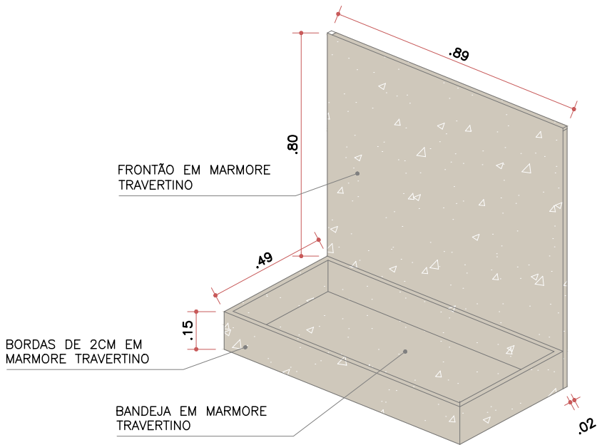
ISOMETRICA PEDRA S/ESCALA
