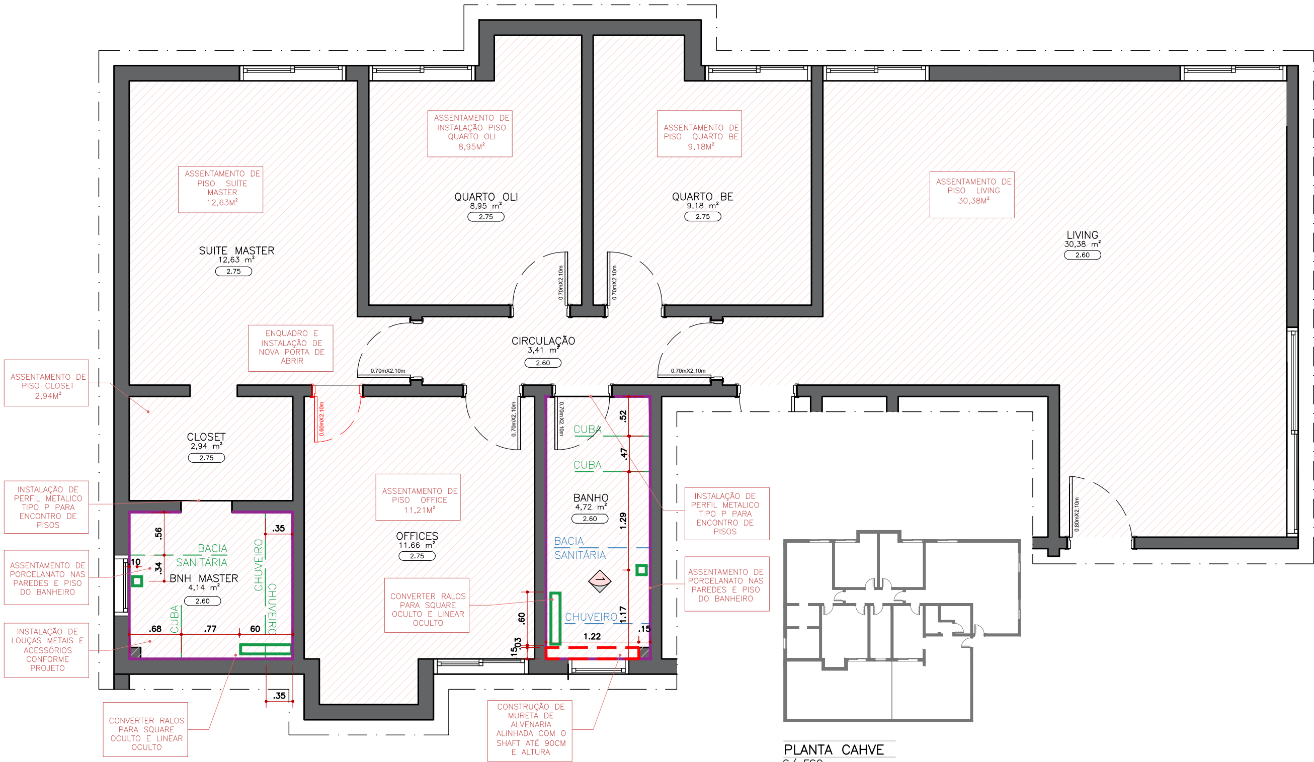
PLANTA BAIXA SECÇÃO 01 ESC. 1:50
