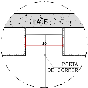
DET. 01 PORTA DE CORRER S/E. VER MEDIDAS NA PLANTA
