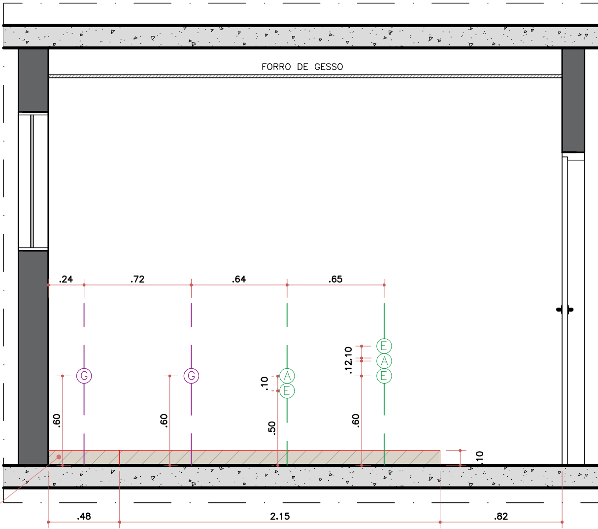
VISTA 02 COZINHA ESC. 1:25
