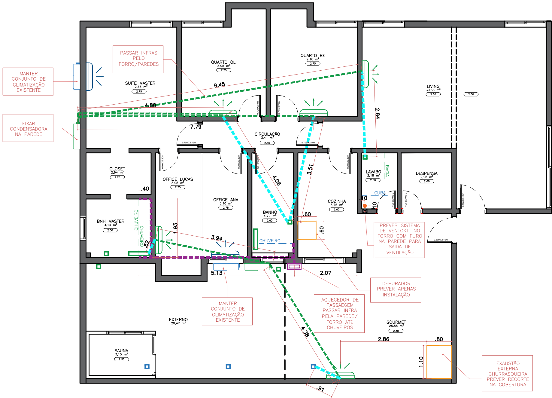
PLANTA BAIXA APTO 101 ESC. 1:75
