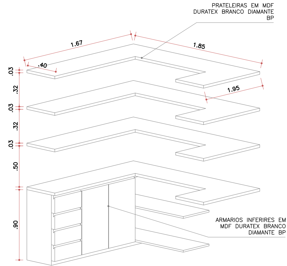
ISOMETRICA DESPENSA S/ESCALA
