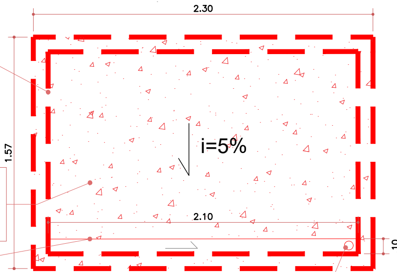
PLANTA COBERTURA HIDRO/SAUNA ESC. 1:25
