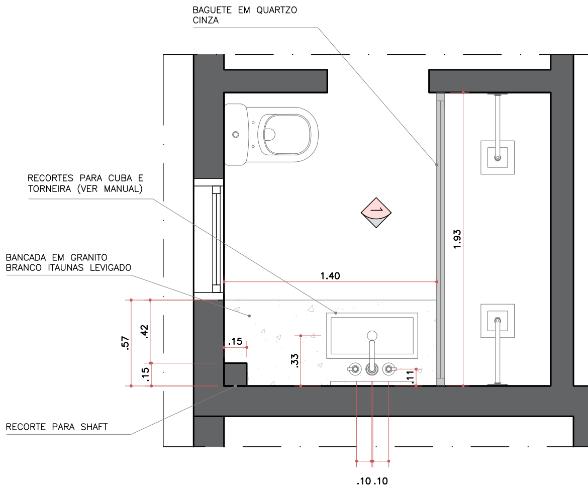
PLANTA BANHO MASTER ESC. 1:25
