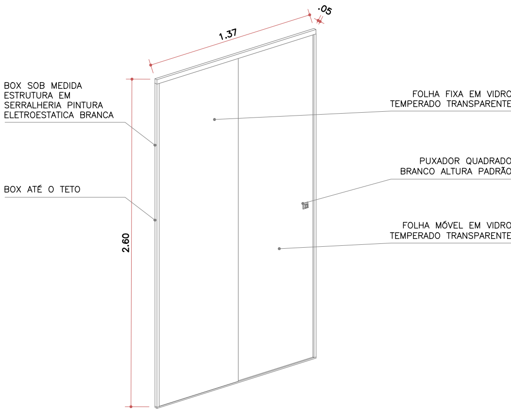
ISOMETRICA BOX S/ESCALA
