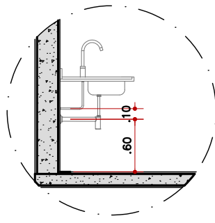
DET. 02 CUBA SEM ESCALA
