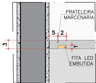
DET.6 FITA LED (SEM ESCALA)
