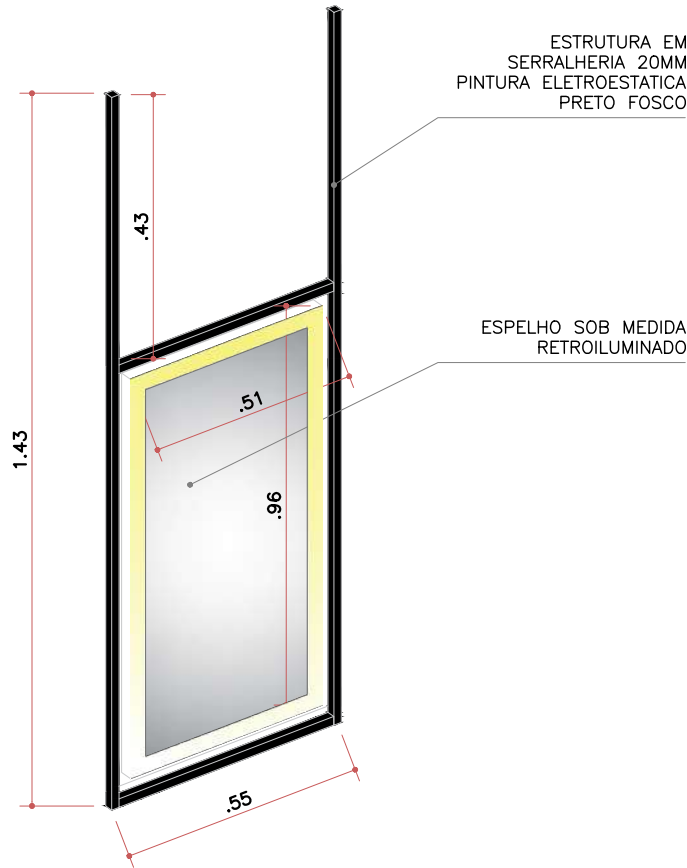
ISOMETRICA ESPELHO S/ESCALA
