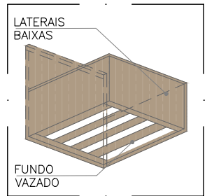
DET.08 GAVETA CESTO (SEM ESCALA)
