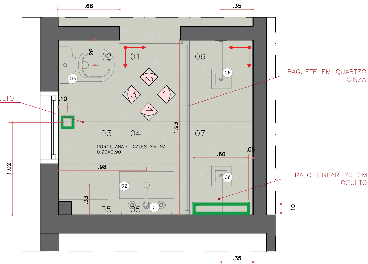
PLANTA BANHO MASTER ESC. 1:25
