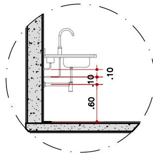
DET. 01 CUBA SEM ESCALA
