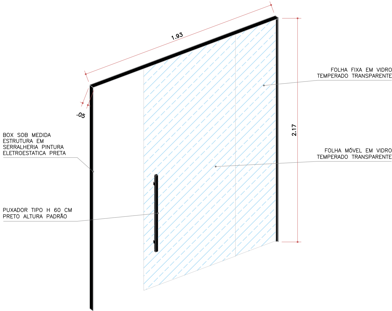
ISOMETRICA BOX S/ESCALA
