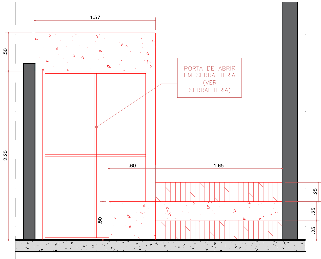
VISTA 01 HIDRO/SAUNA ESC. 1:25
