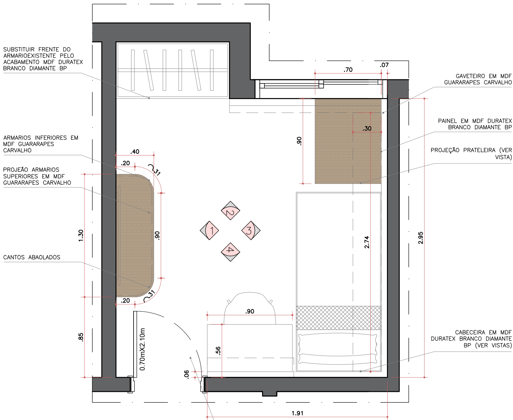
PLANTA QUARTO BE ESC. 1:25
