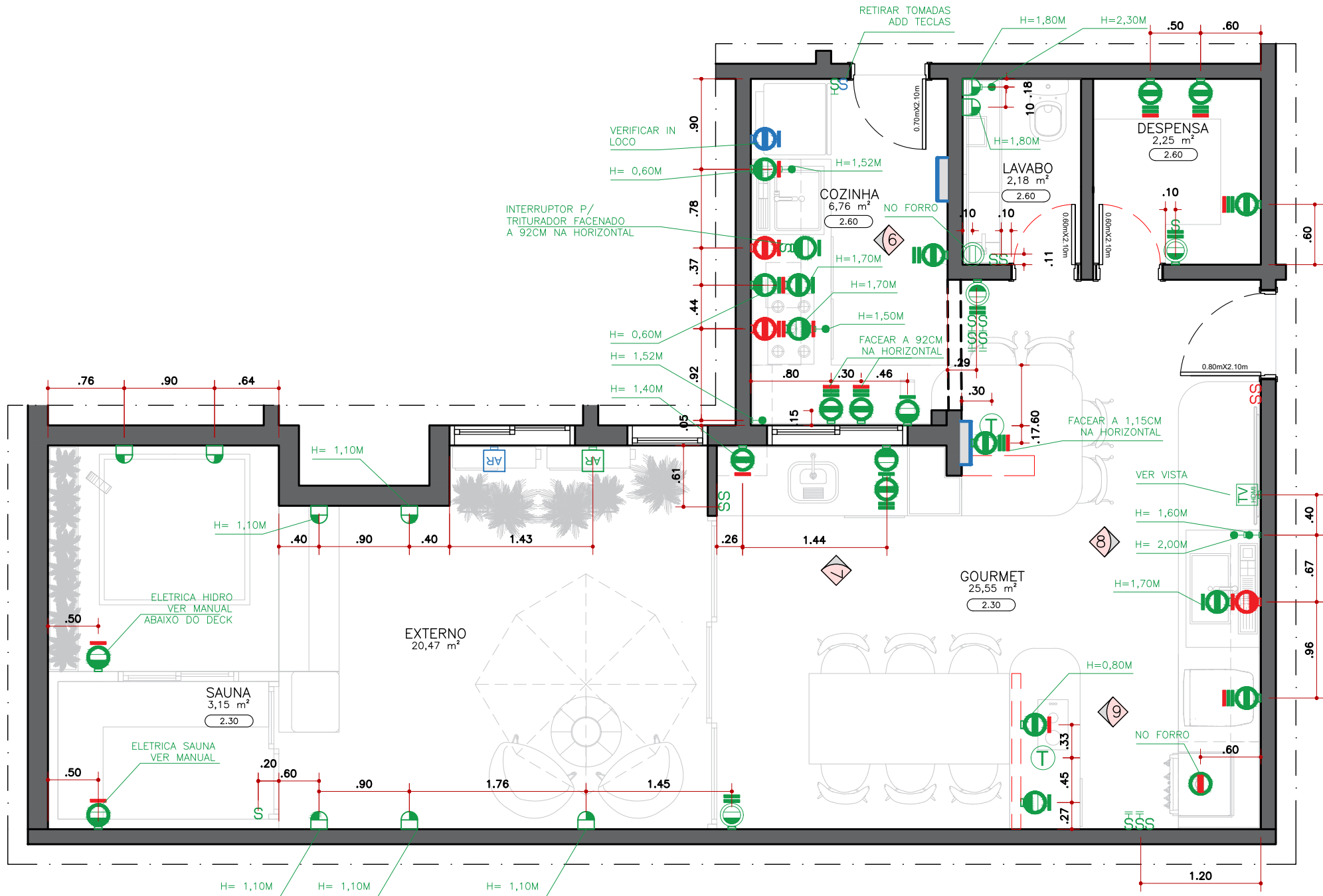
PLANTA BAIXA SECÇÃO 02 ESC. 1:50
