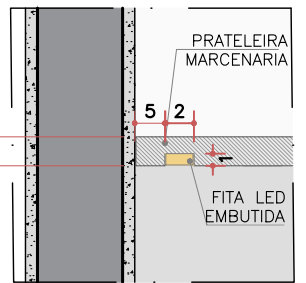
DET.6 FITA LED (SEM ESCALA)
