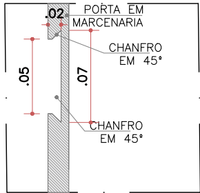
DET.12 PUXADOR CAVA (SEM ESCALA) EM PLANTA
