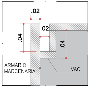
DET. 01 PUXADOR (SEM ESCALA)
