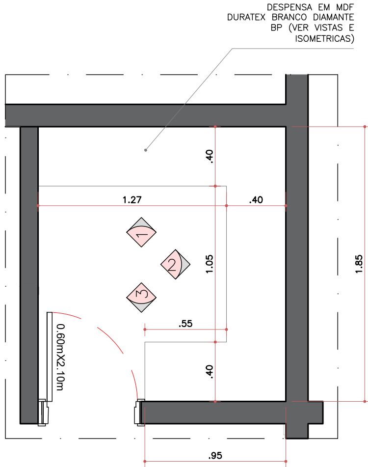
PLANTA DESPENSA ESC. 1:25
