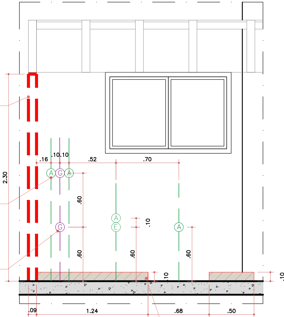
VISTA 04 ÁREA DE SERVIÇO ESC. 1:25
