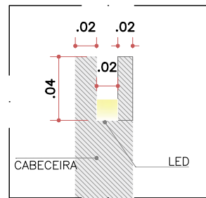
DET. 05 PUXADOR (SEM ESCALA)
