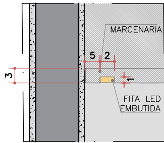
DET.2 FITA LED (SEM ESCALA)
