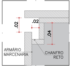
DET.10 CAVA RETA (SEM ESCALA)
