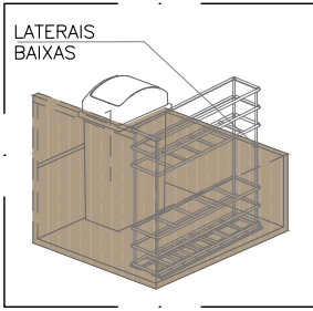
DET.21 GAVETA LIXEIRA (SEM ESCALA)
