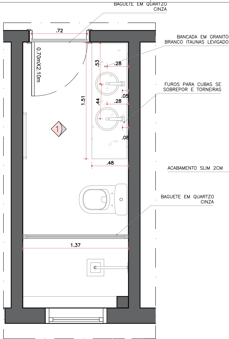
VISTA 01 BANHO ESC. 1:25
