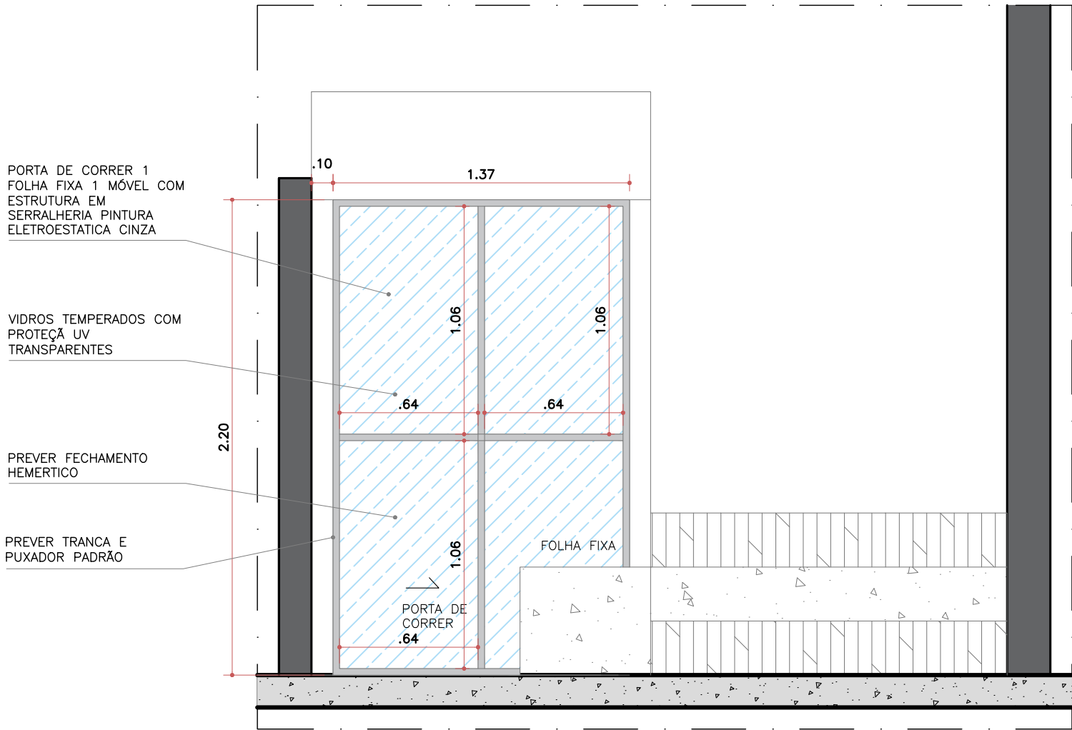
VISTA 01 HIDRO/SAUNA ESC. 1:25
