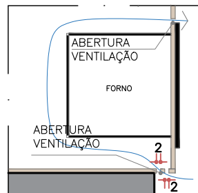
DET.11 FÓRNO (SEM ESCALA)
