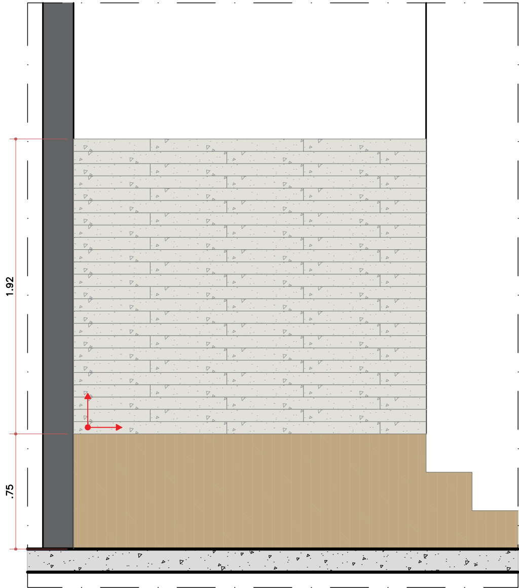
VISTA 02 HIDRO/SAUNA ESC. 1:25
