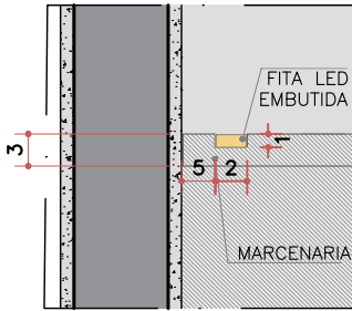
DET.4 FITA LED (SEM ESCALA)
