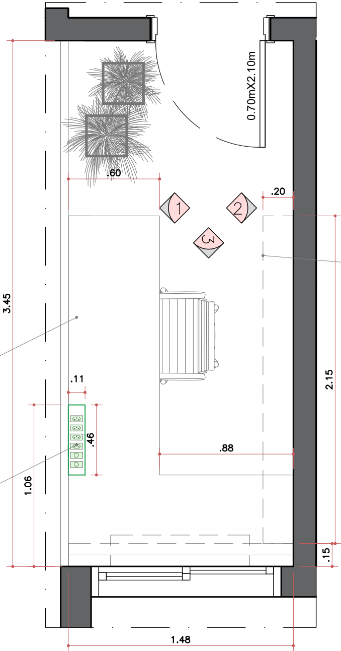
PLANTA OFFICE ANA ESC. 1:25
