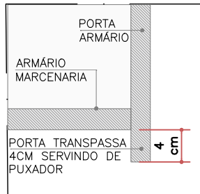
DET.3 PUXADOR PORTA (SEM ESCALA)
