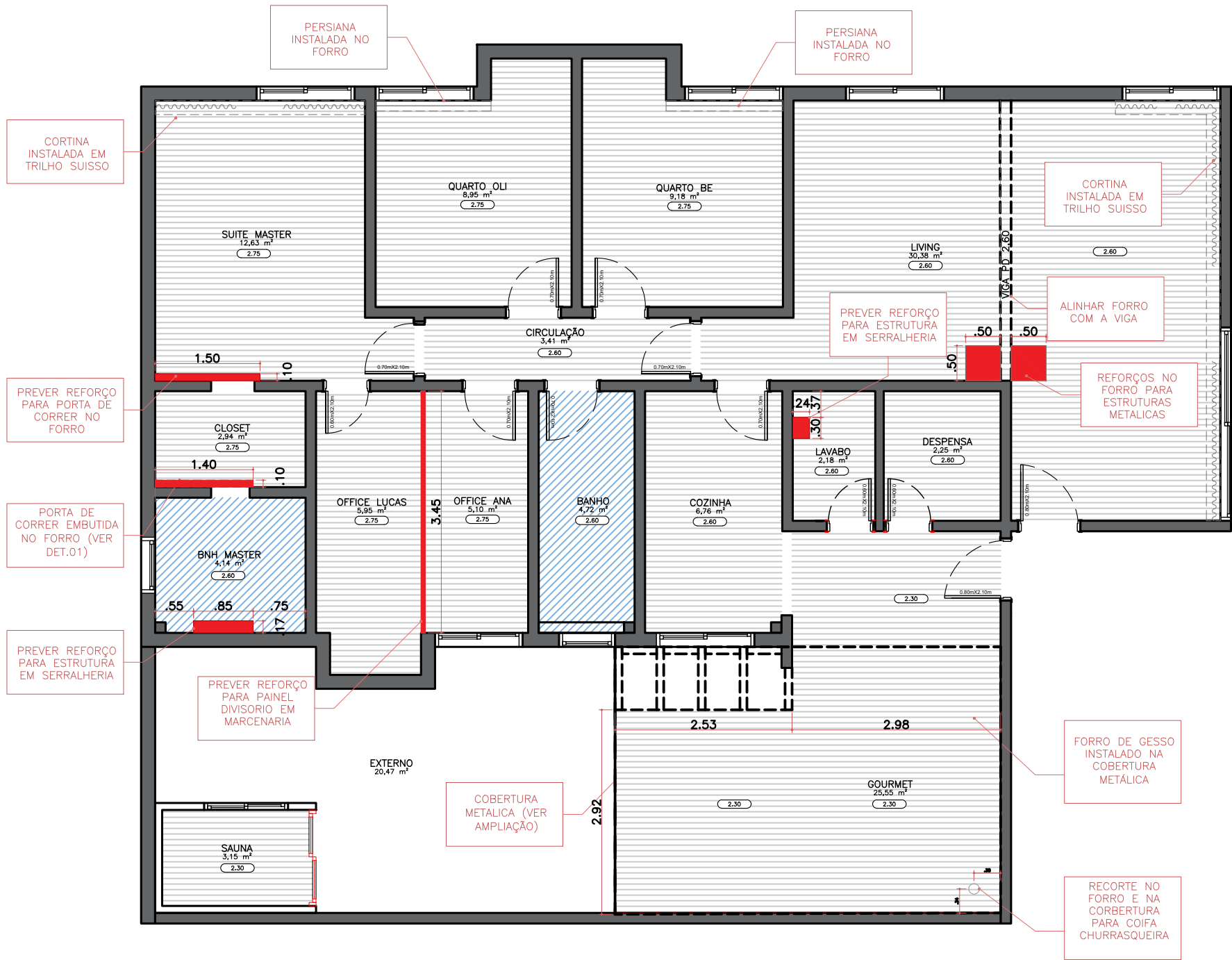
PLANTA BAIXA APTO 101 ESC. 1:75
