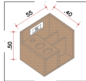
DET.07 GAVETA (SEM ESCALA)
