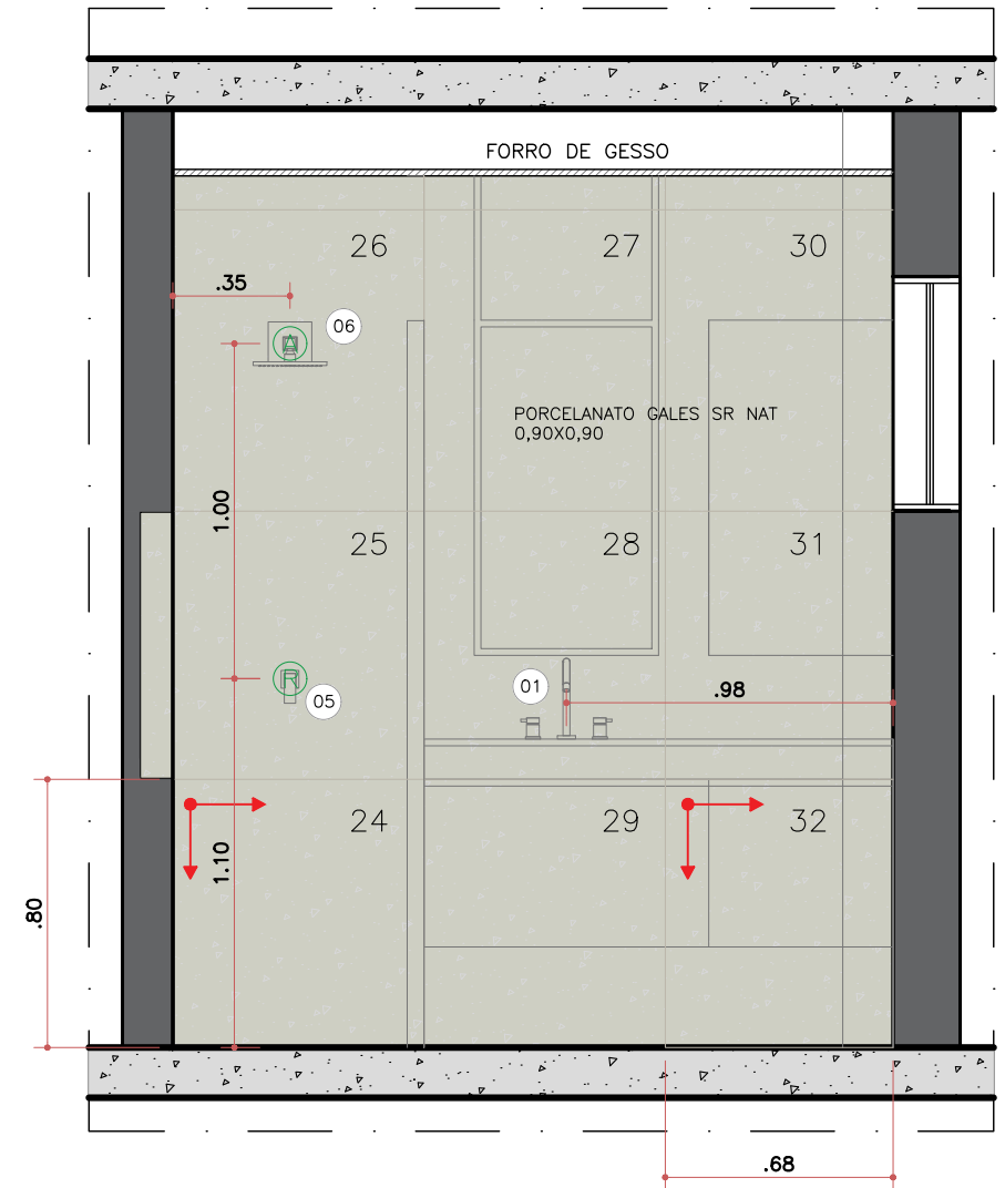
VISTA 04 BANHO MASTER ESC. 1:25
