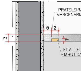
DET.6 FITA LED (SEM ESCALA)
