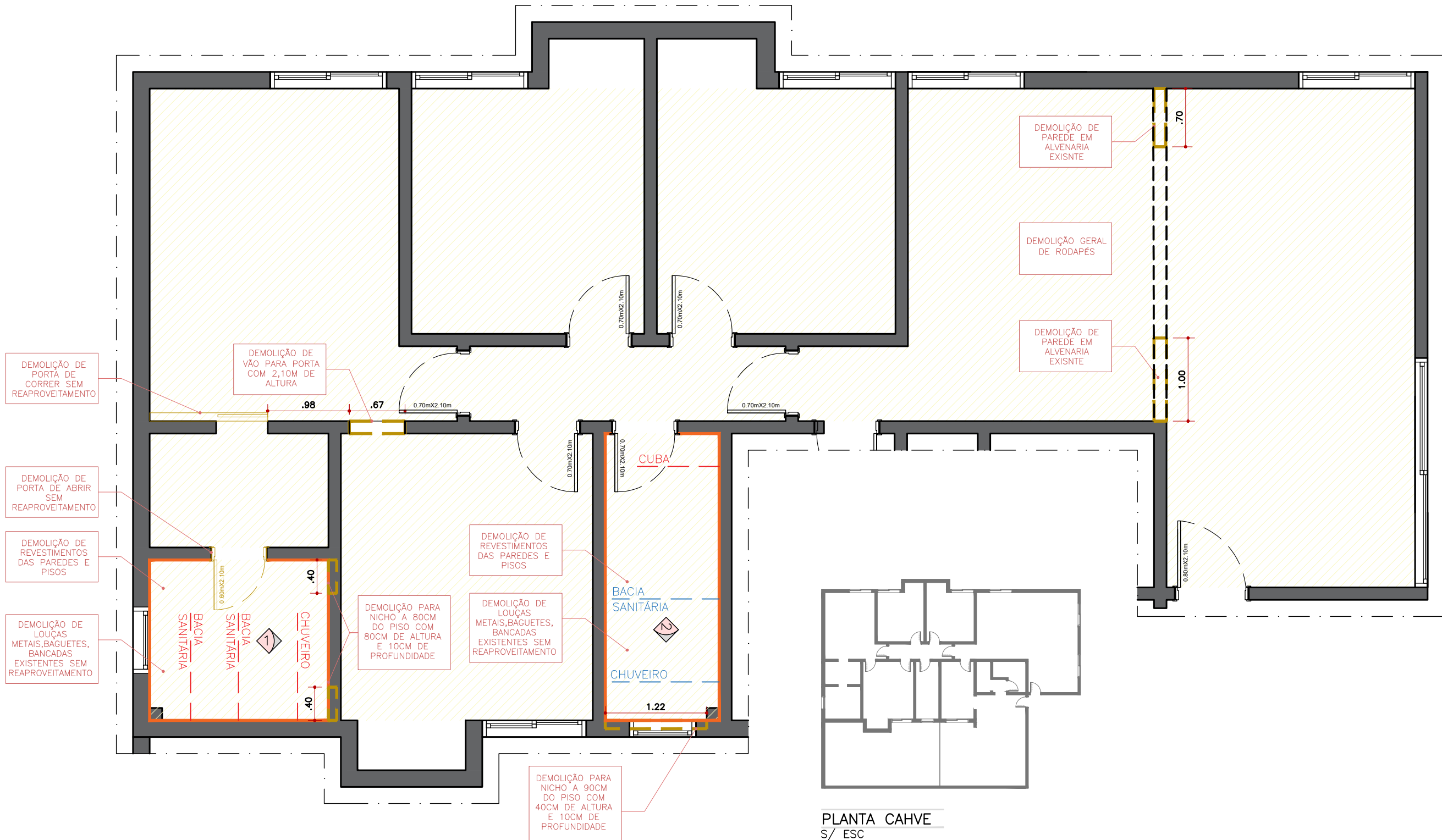
PLANTA BAIXA SECÇÃO 01 ESC. 1:50
