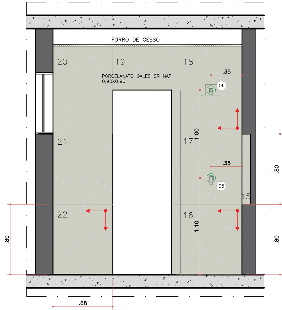
VISTA 02 BANHO MASTER ESC. 1:25
