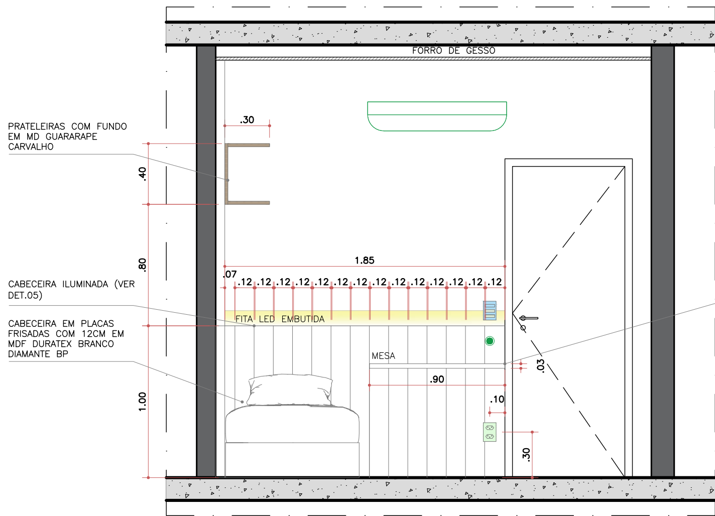
MESA ESTUDOS EM MDF DURATEX BRANCO DIAMANTE BP
