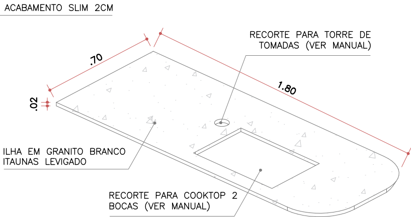
ISOMETRICA PEDRA S/ESCALA
