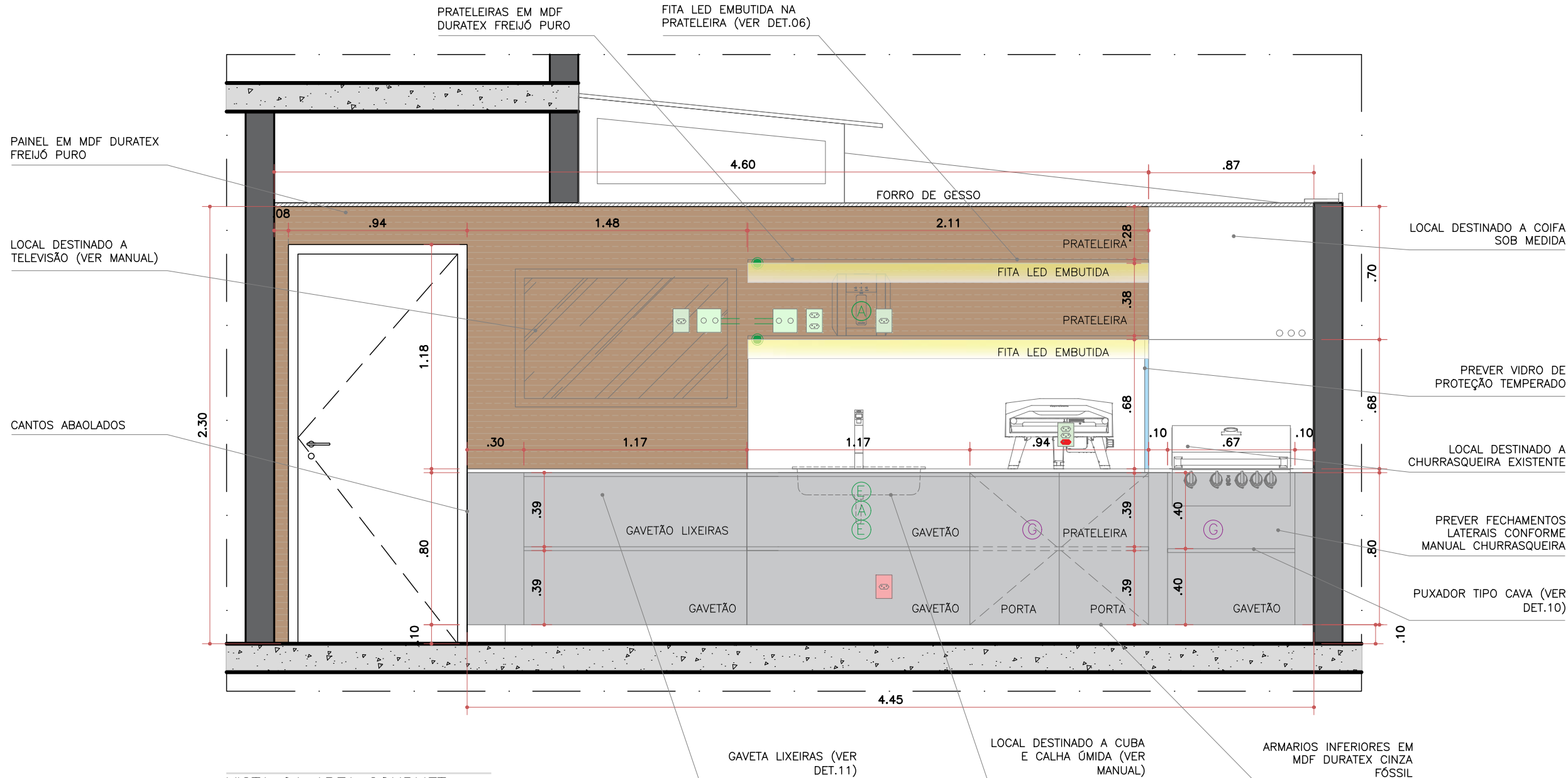
VISTA 01 AREA GOURMET ESC. 1:25
