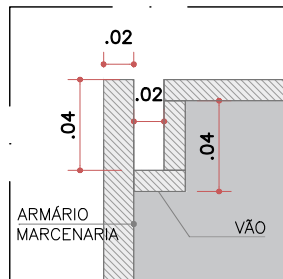
DET. 01 PUXADOR (SEM ESCALA)
