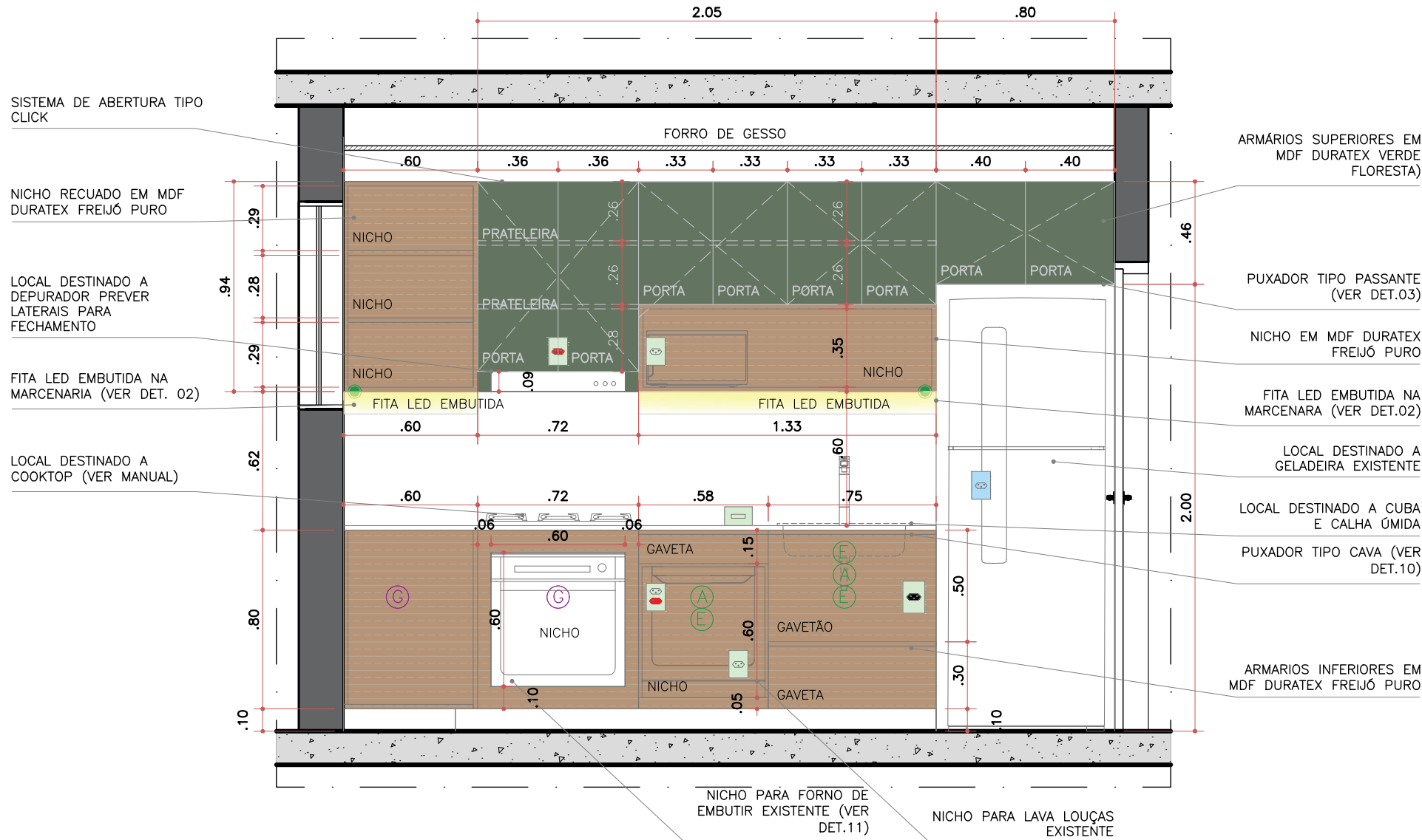
VISTA 01 COZINHA ESC. 1:25
