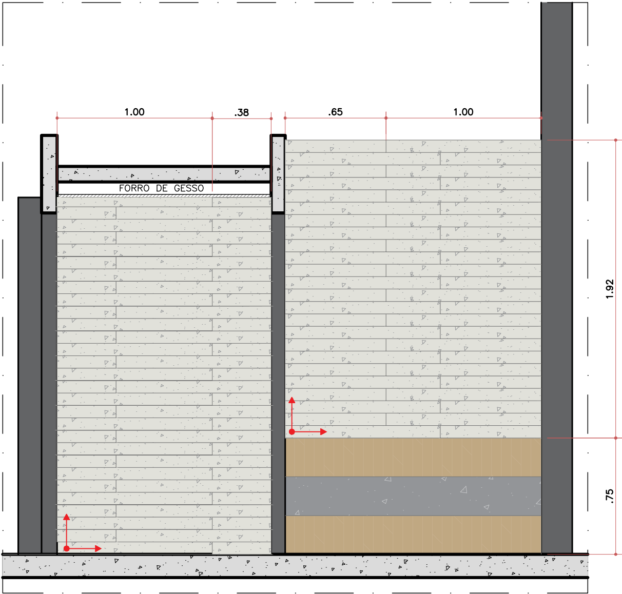
VISTA 01 HIDRO/SAUNA ESC. 1:25
