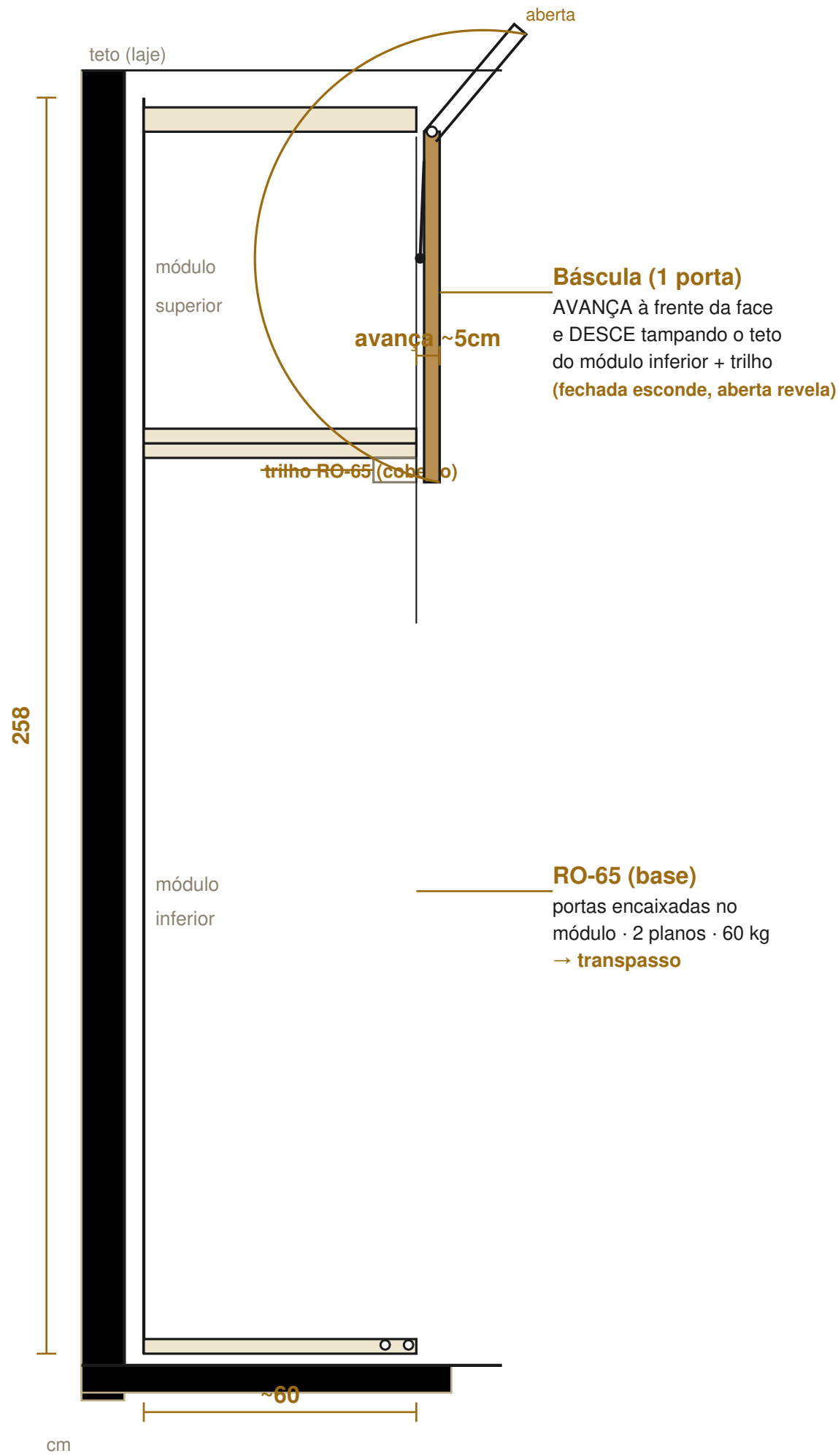
V3 — superior BÁSCULA avançada tampa o teto do módulo inferior + trilho
