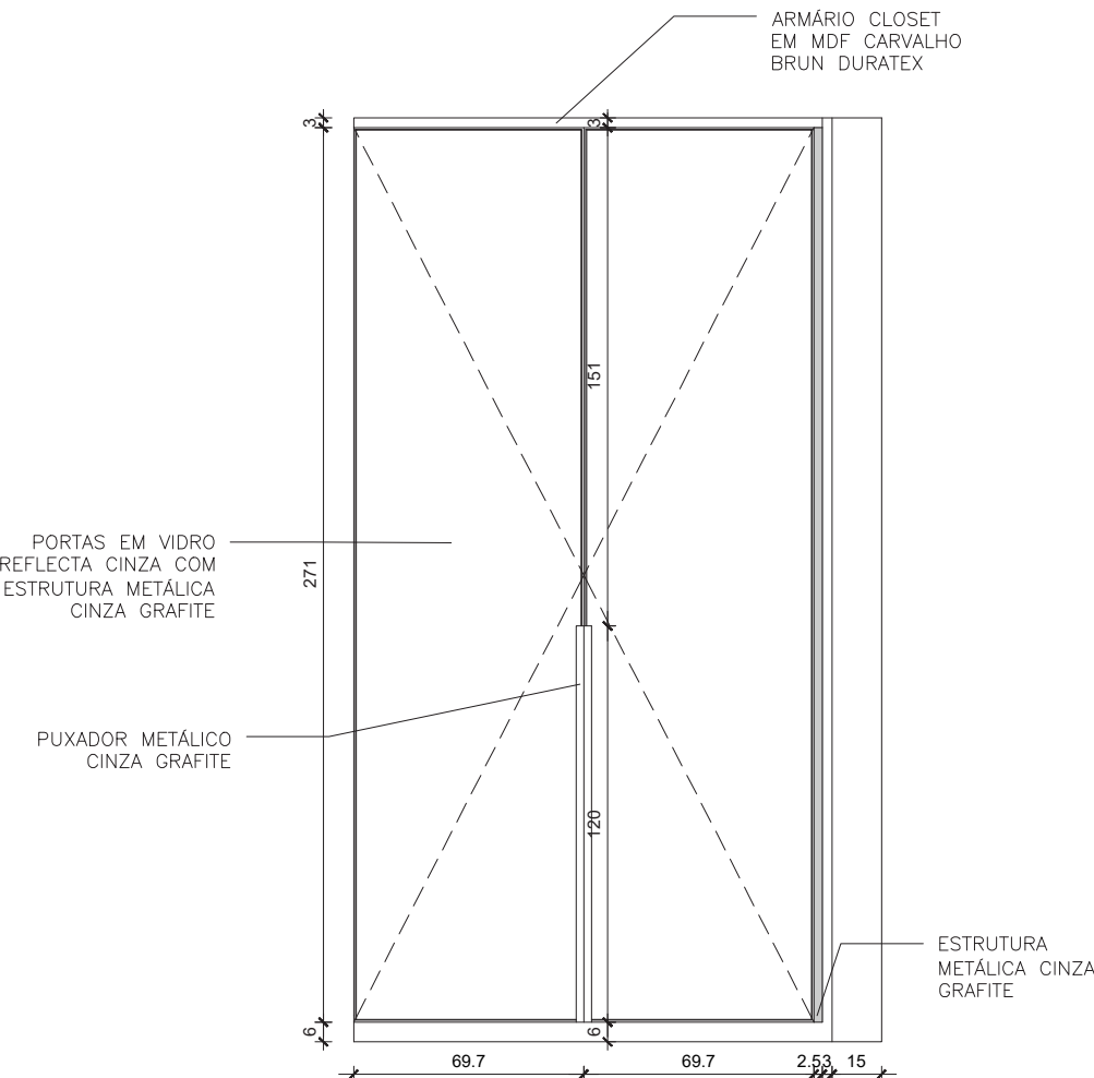
ELEVAÇÃO V5 ESCALA 1:25
