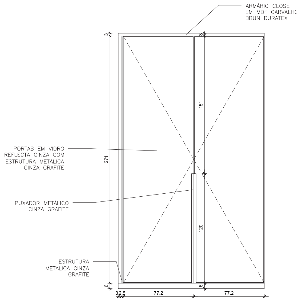
ELEVAÇÃO V3 ESCALA 1:25
