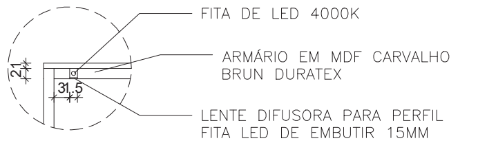
DETALHE 11 - FITA DE LED CLOSET ESCALA 1:10
