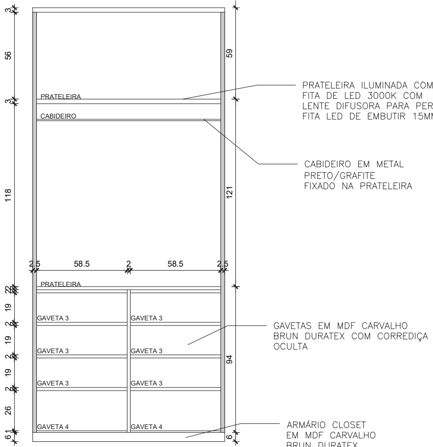
ELEVAÇÃO V4 - INTERNO ESCALA 1:25
