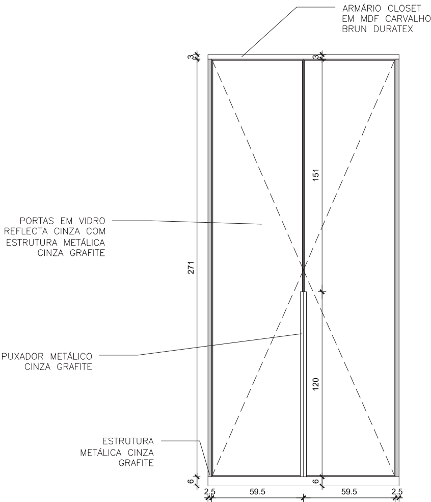
ELEVAÇÃO V4 ESCALA 1:25
