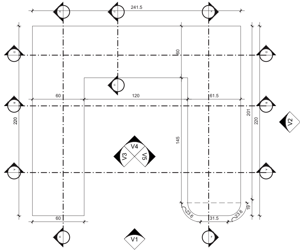
PLANTA - CLOSET ESCALA 1:25
