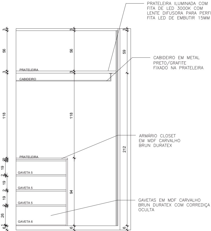
ELEVAÇÃO V5 - INTERNO ESCALA 1:25
