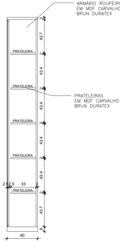
CORTE AA - ARMÁRIO ROUPEIRO ESCALA 1:25
