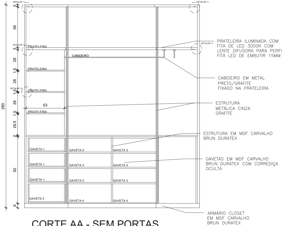
CORTE AA - SEM PORTAS ESCALA 1:25
