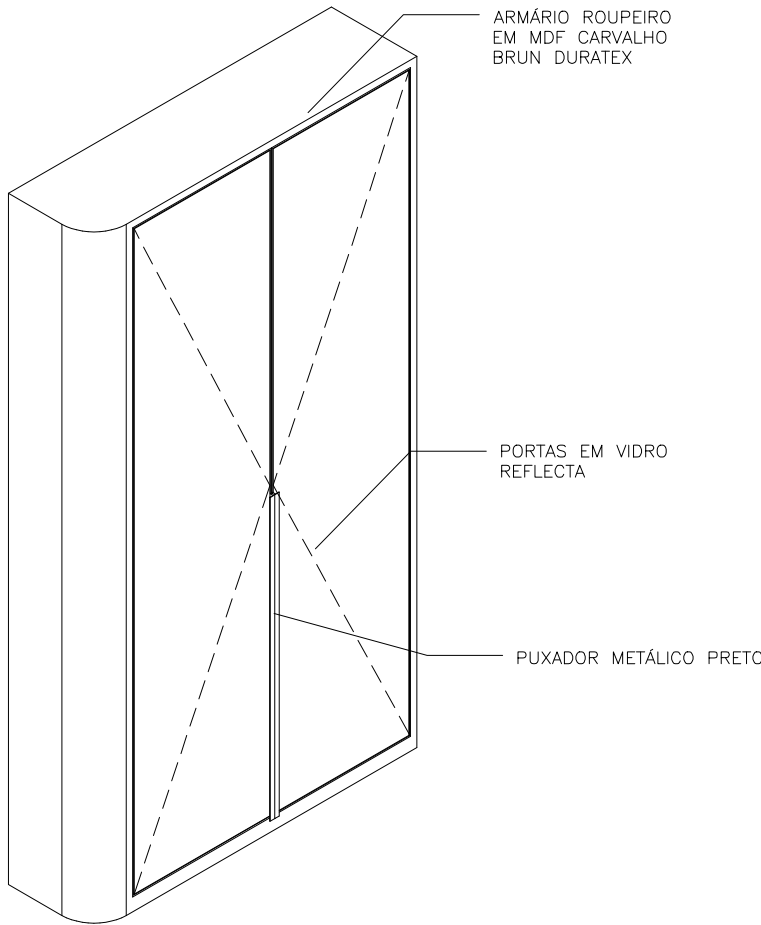
ISOMÉTRICA - ARMÁRIO ROUPEIRO ESCALA 1:25
