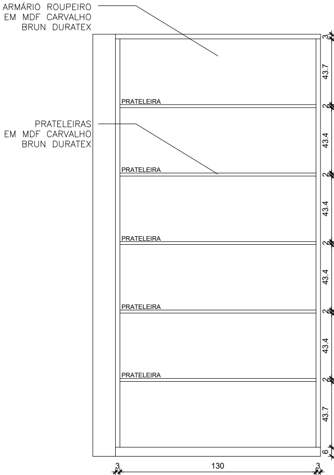
ELEVAÇÃO FRONTAL INTERNO - ARMÁRIO ROUPEIRO ESCALA 1:25
