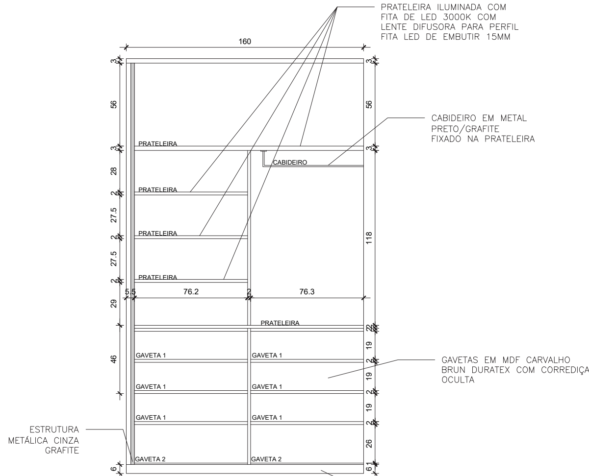
ELEVAÇÃO V3 - INTERNO ESCALA 1:25
