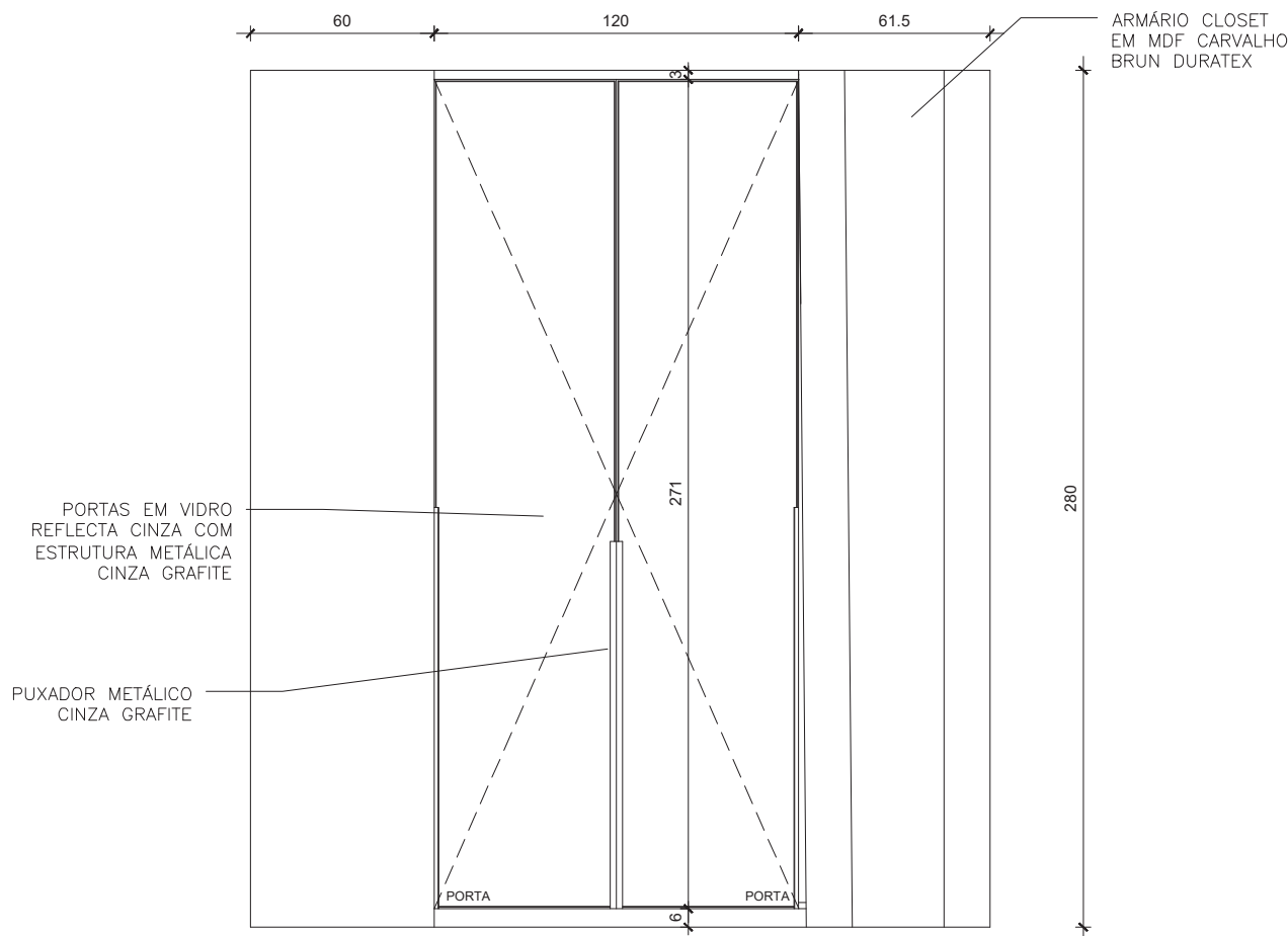
ELEVAÇÃO V1 ESCALA 1:25
