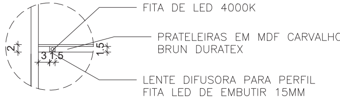
DETALHE 12 - FITA DE LED PRATELEIRAS ESCALA 1:10
