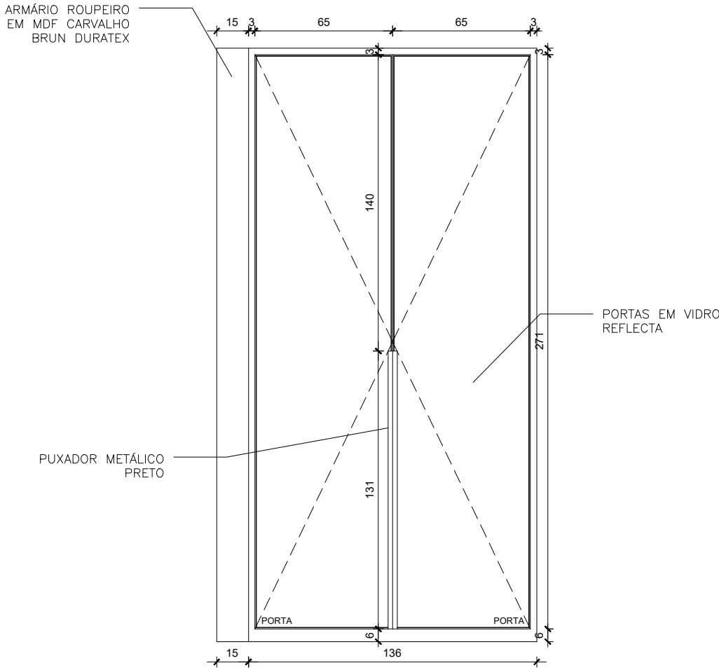
ELEVAÇÃO FRONTAL - ARMÁRIO ROUPEIRO ESCALA 1:25
