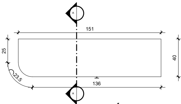
PLANTA - ARMÁRIO SAPATEIRA ESCALA 1:25
