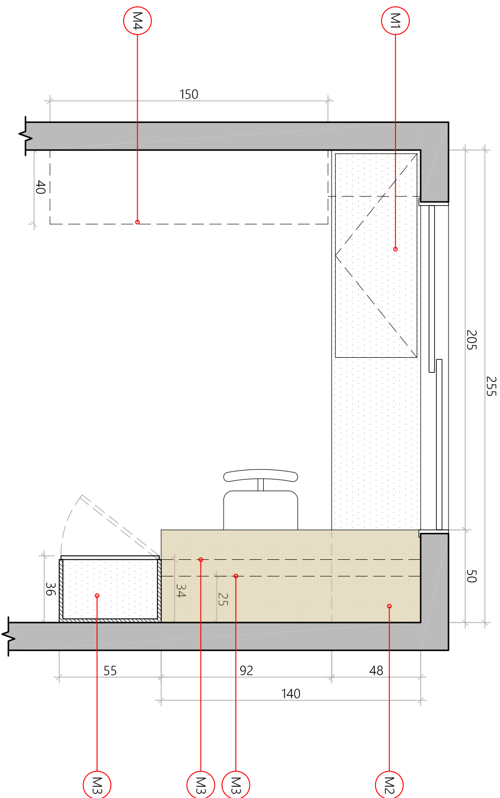
PLANTA GERAL ESC. 1/20
