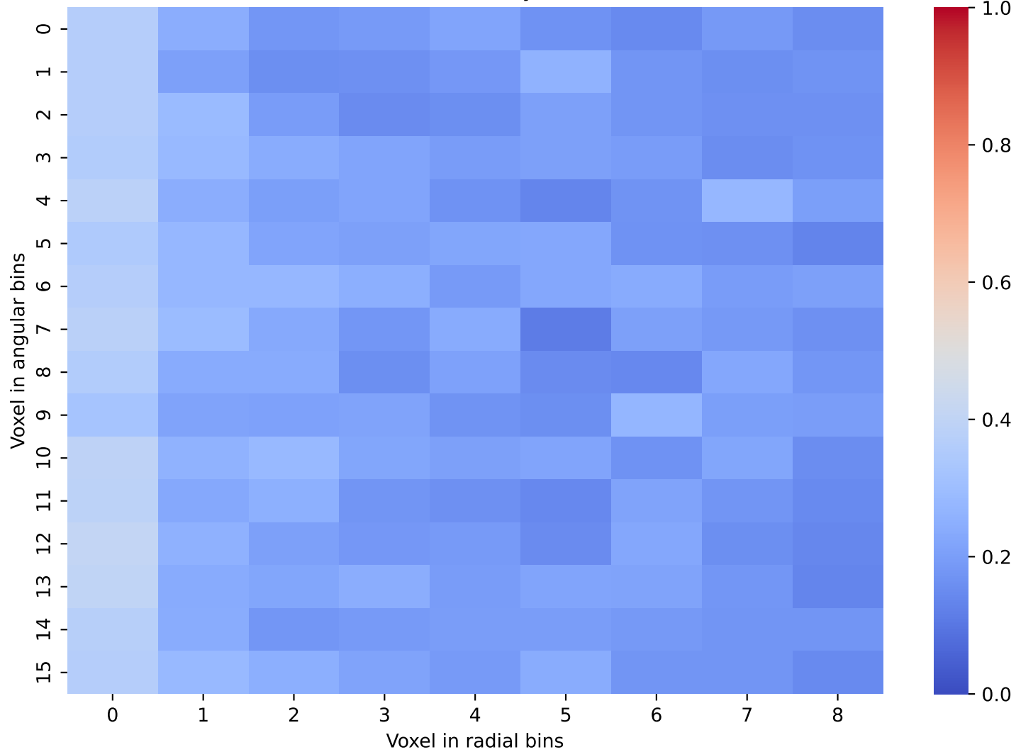
CaloDiffusion Data: Layer 37 and 38
