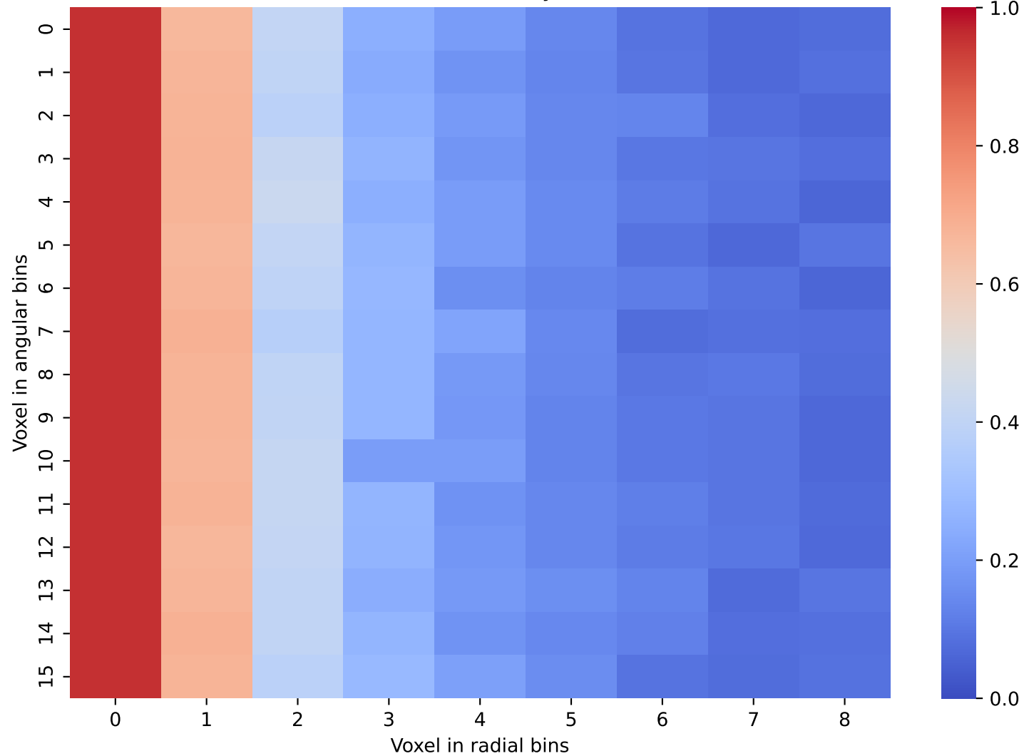
CaloDiffusion Data: Layer 8 and 9
