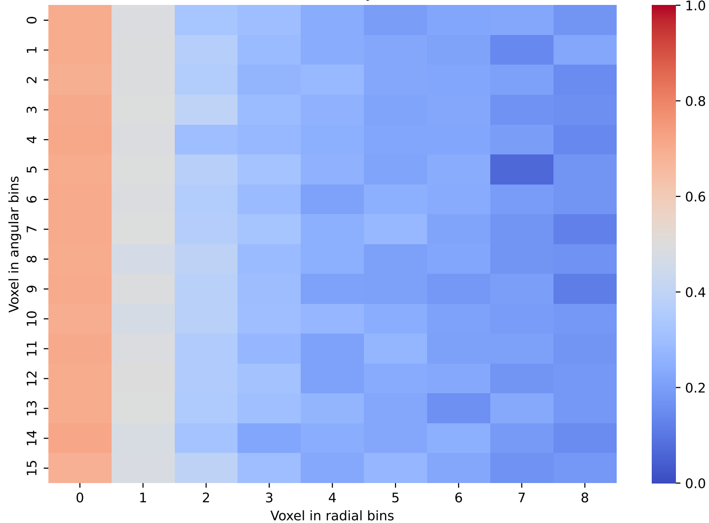
CaloDiffusion Data: Layer 32 and 33
