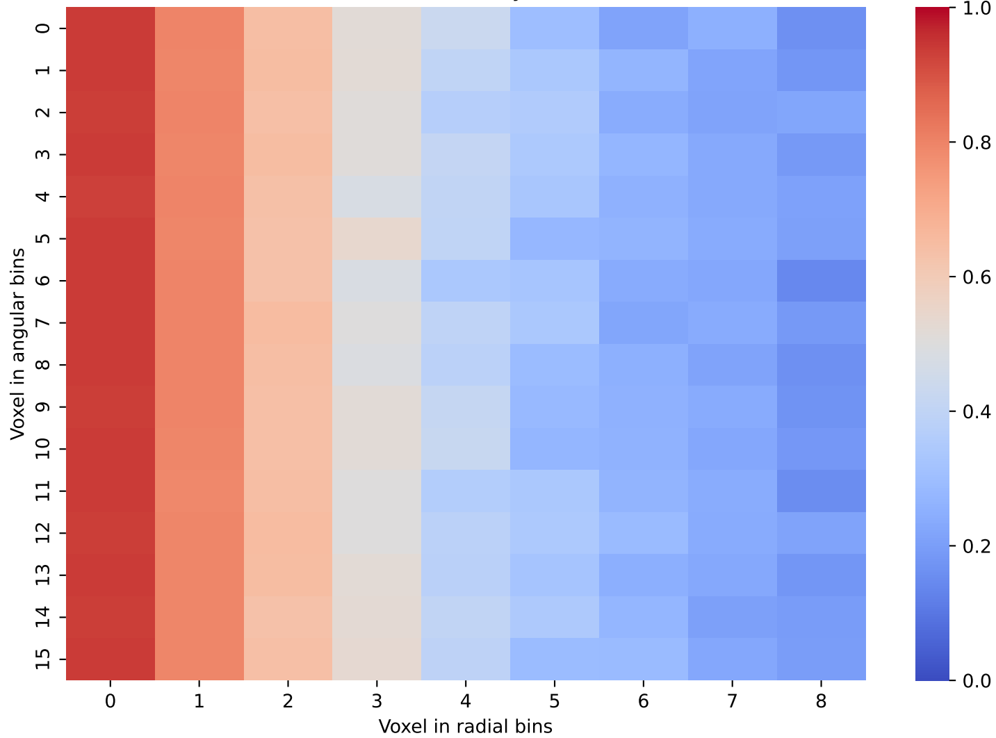
CaloDiffusion Data: Layer 24 and 25
