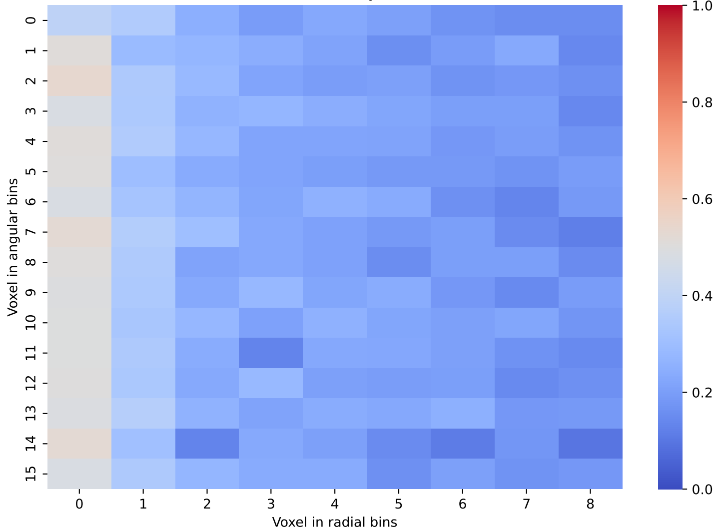
CaloDiffusion Data: Layer 35 and 36
