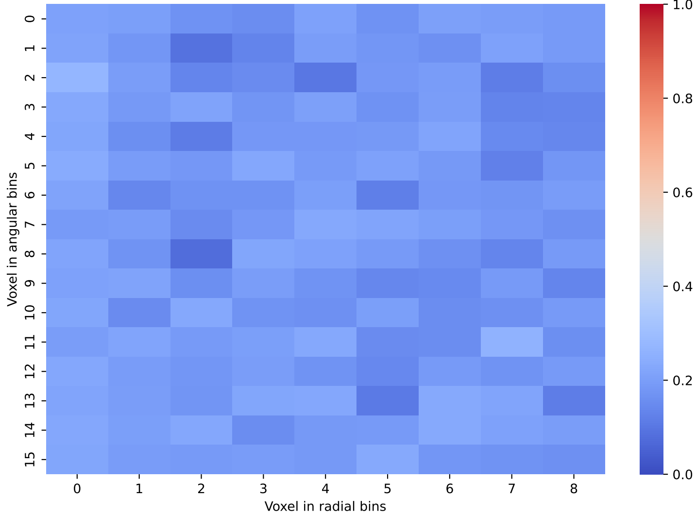
CaloDiffusion Data: Layer 40 and 41
