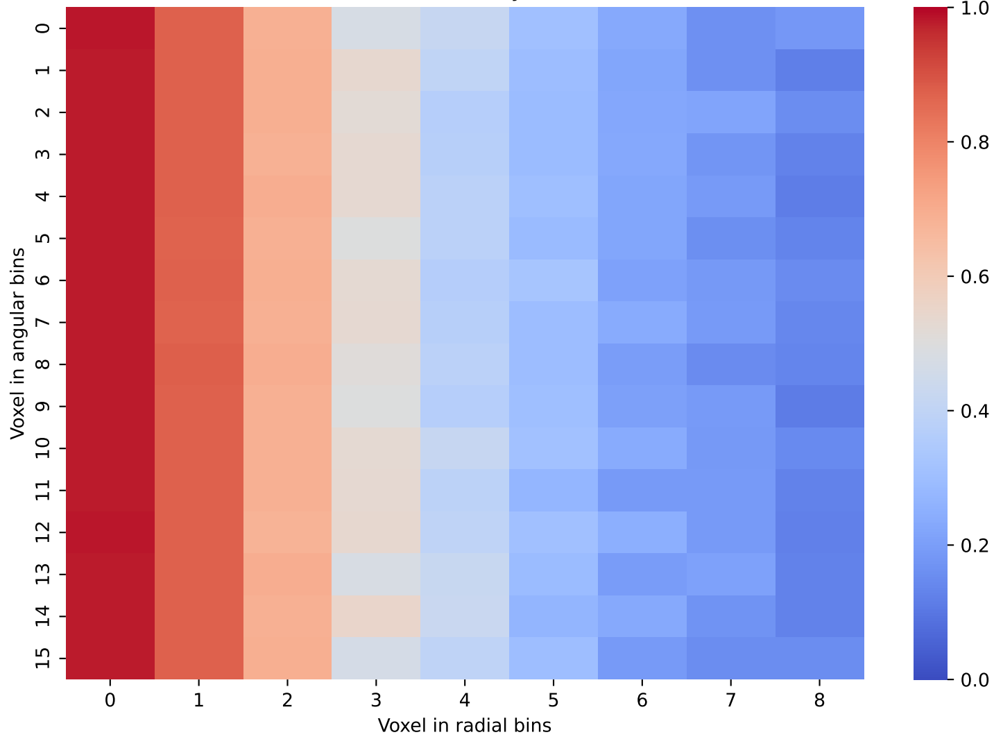
CaloDiffusion Data: Layer 14 and 15
