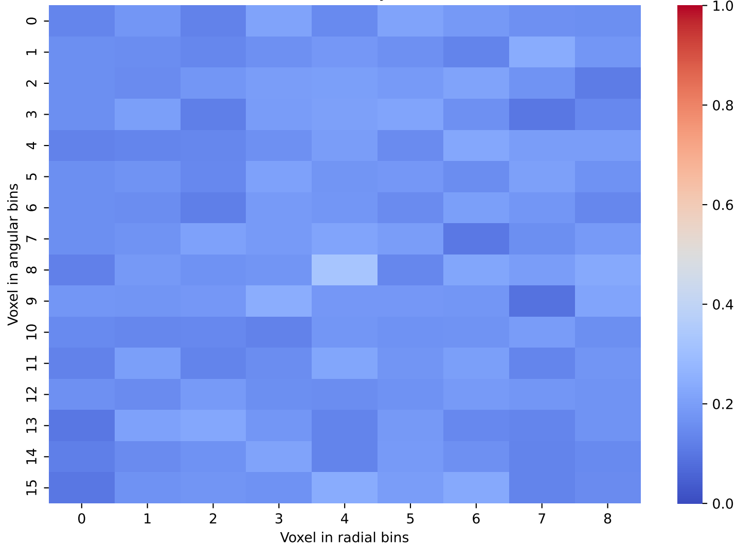
CaloDiffusion Data: Layer 42 and 43
