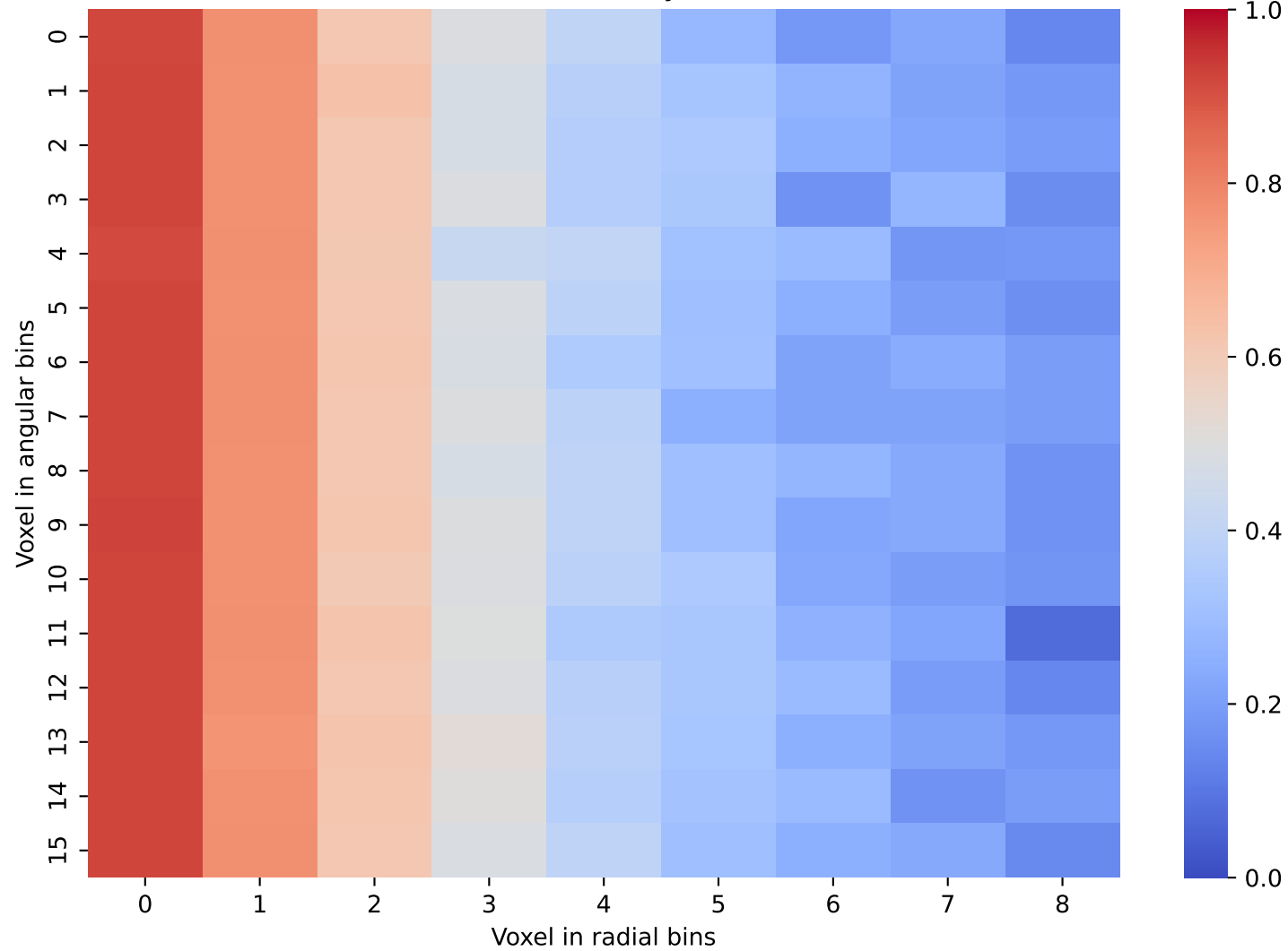
CaloDiffusion Data: Layer 25 and 26
