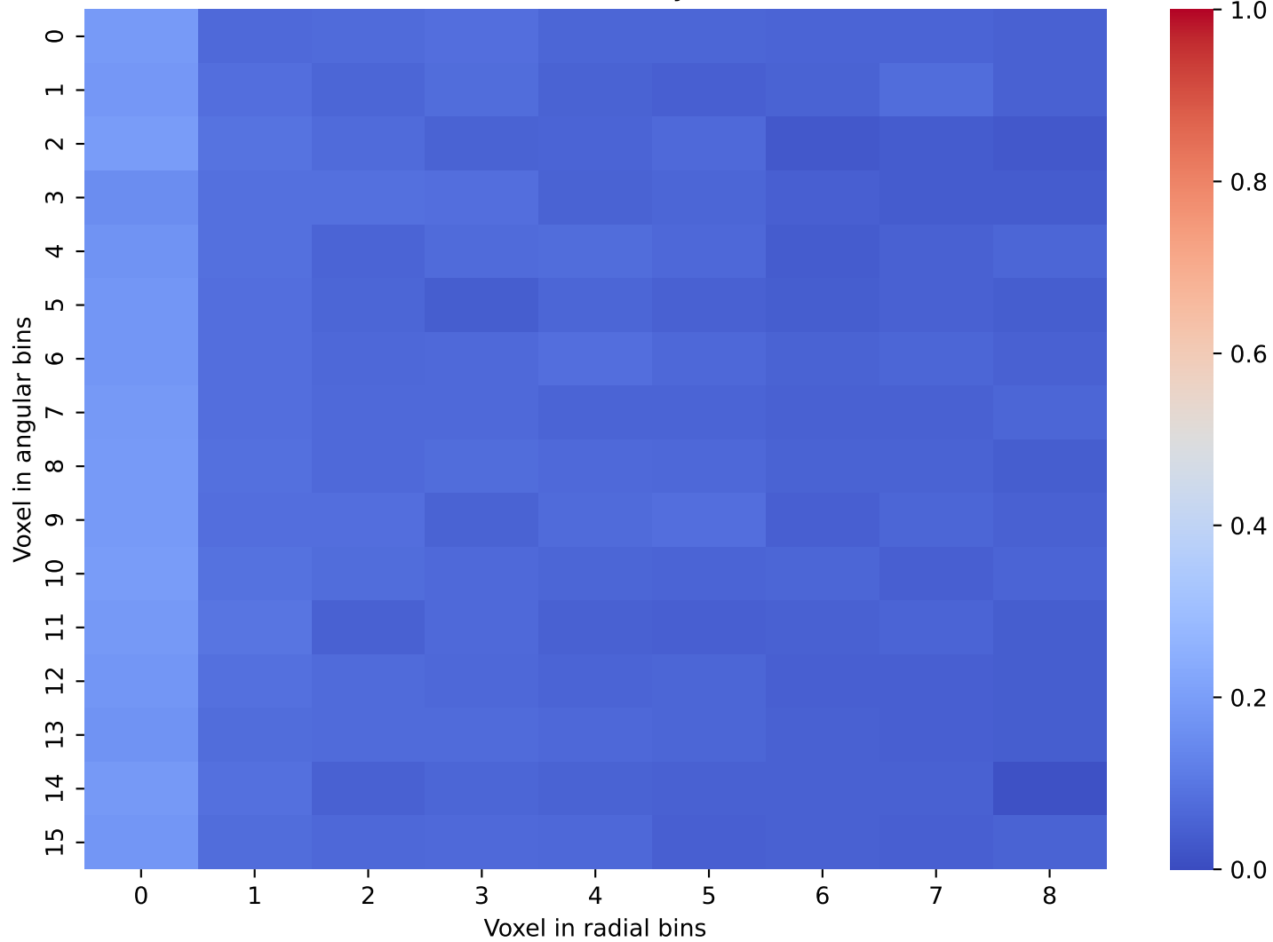
CaloDiffusion Data: Layer 2 and 3
