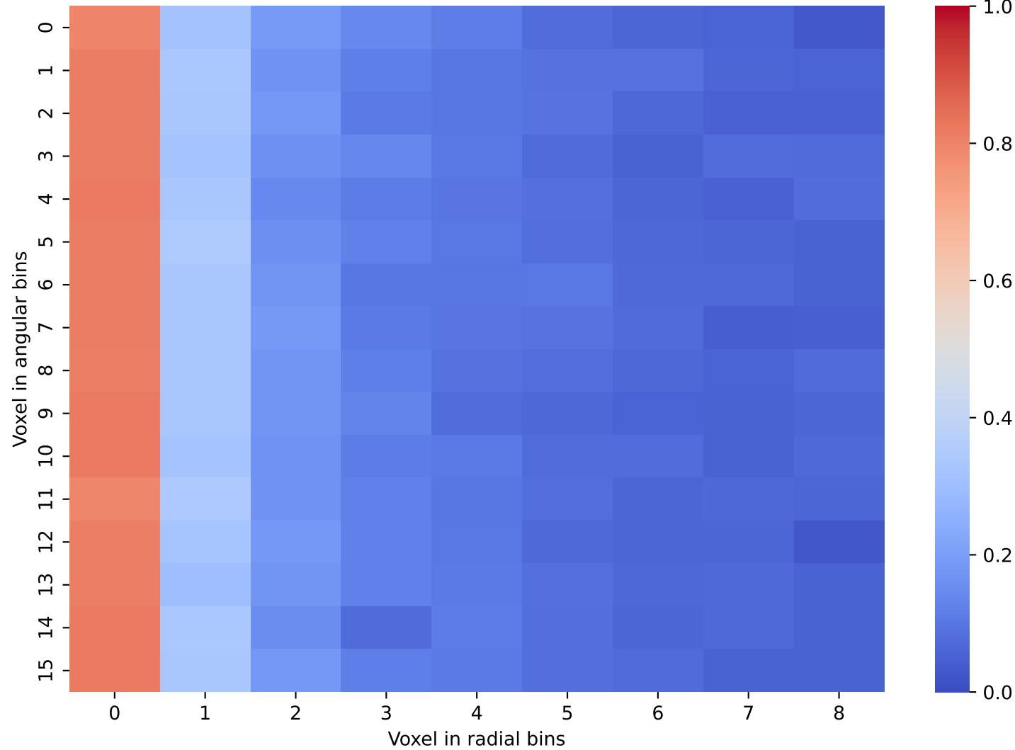
CaloDiffusion Data: Layer 5 and 6
