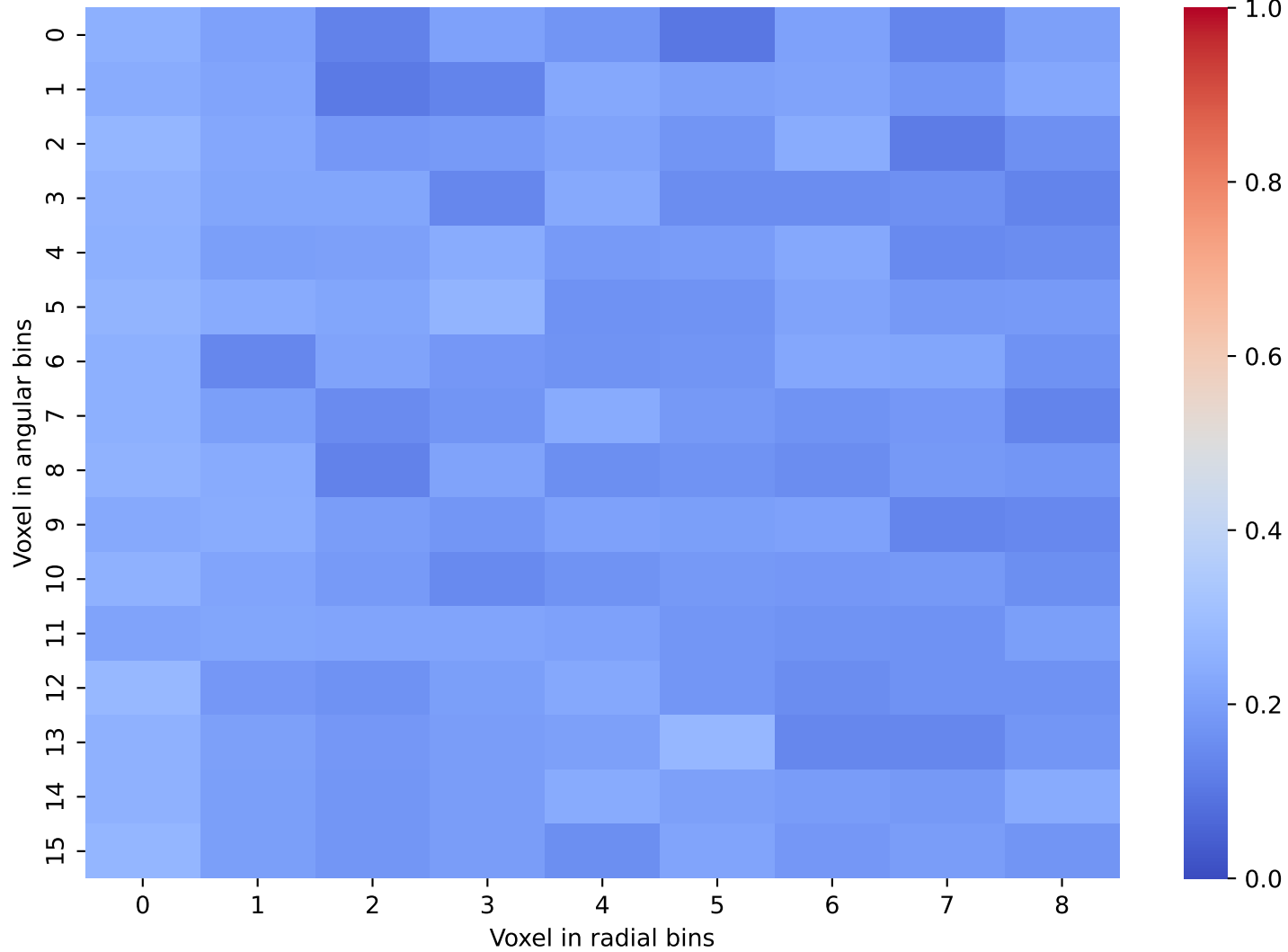
CaloDiffusion Data: Layer 39 and 40
