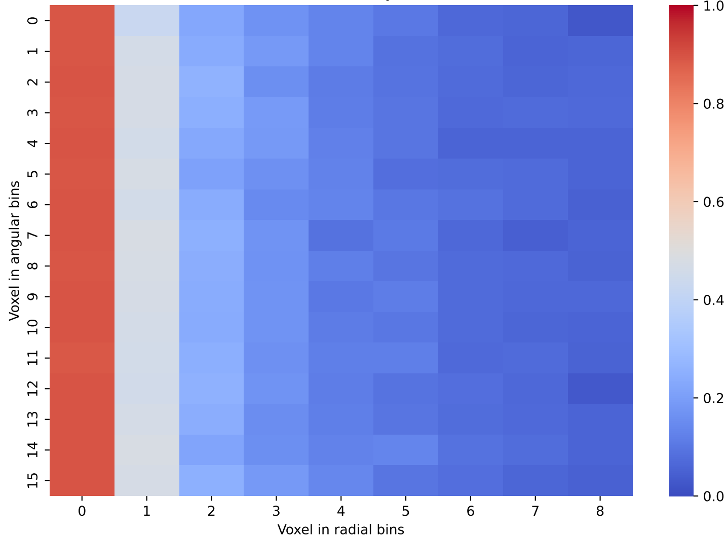
CaloDiffusion Data: Layer 6 and 7
