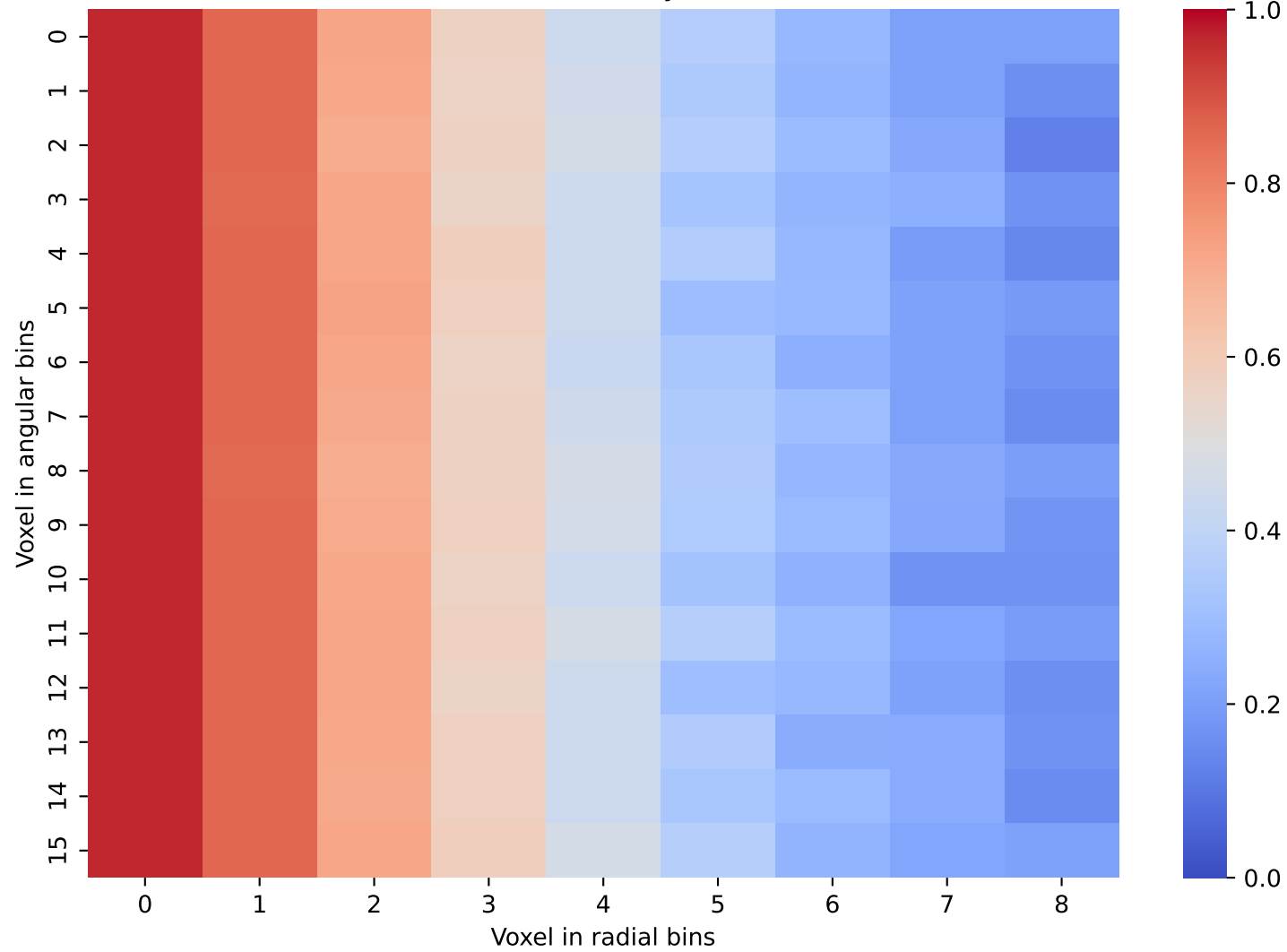
CaloDiffusion Data: Layer 20 and 21
