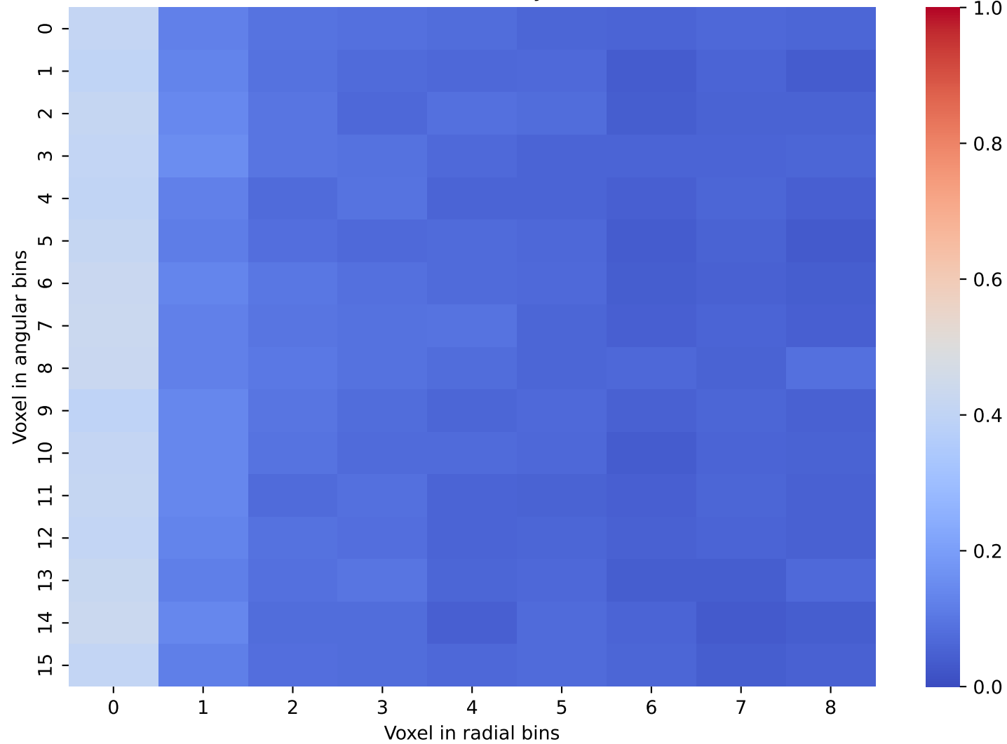
CaloDiffusion Data: Layer 3 and 4
