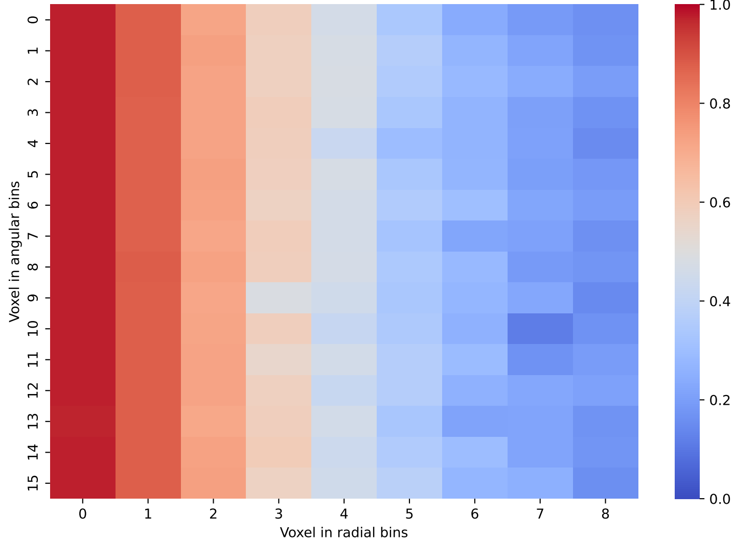
CaloDiffusion Data: Layer 18 and 19
