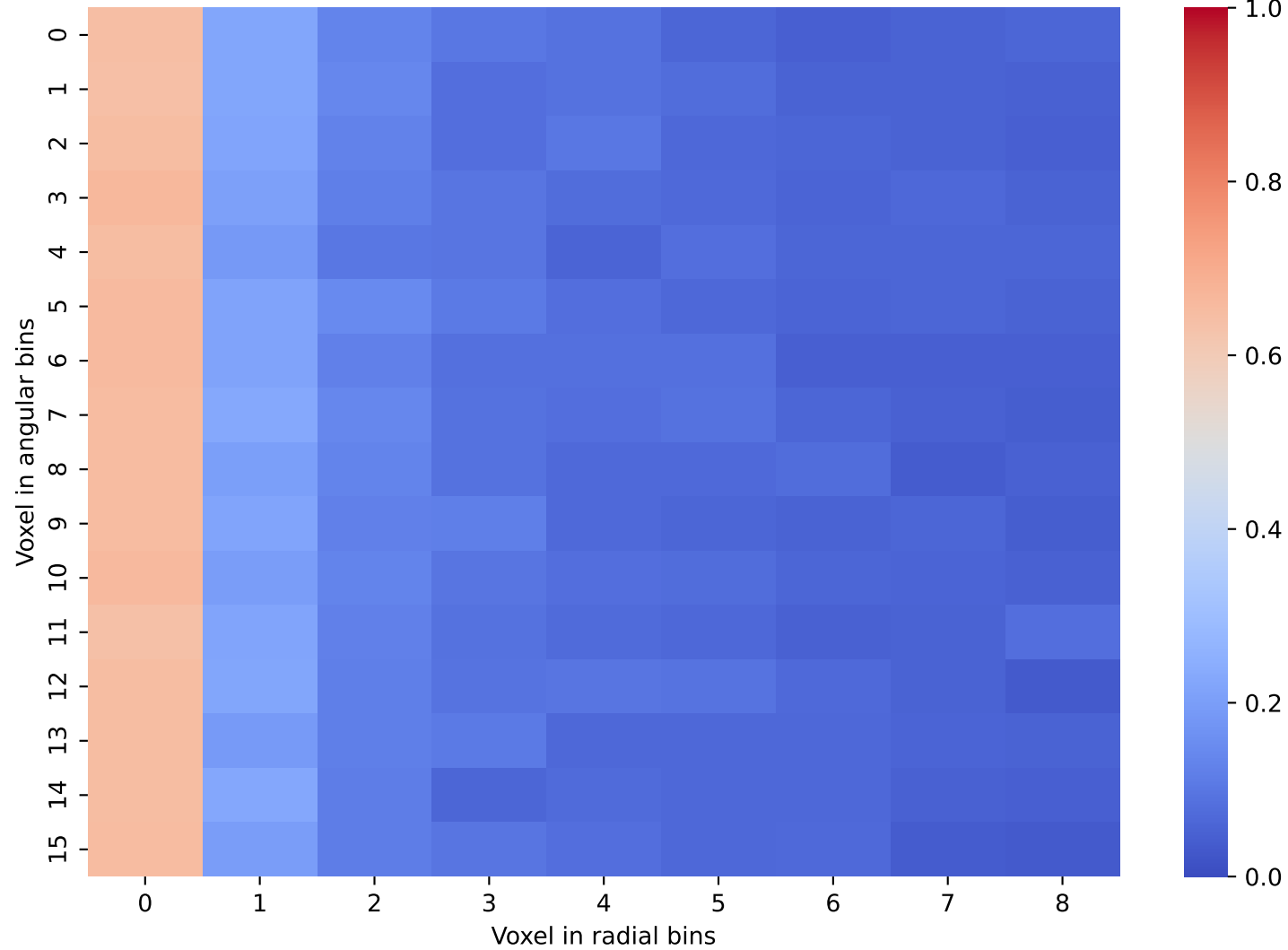
CaloDiffusion Data: Layer 4 and 5
