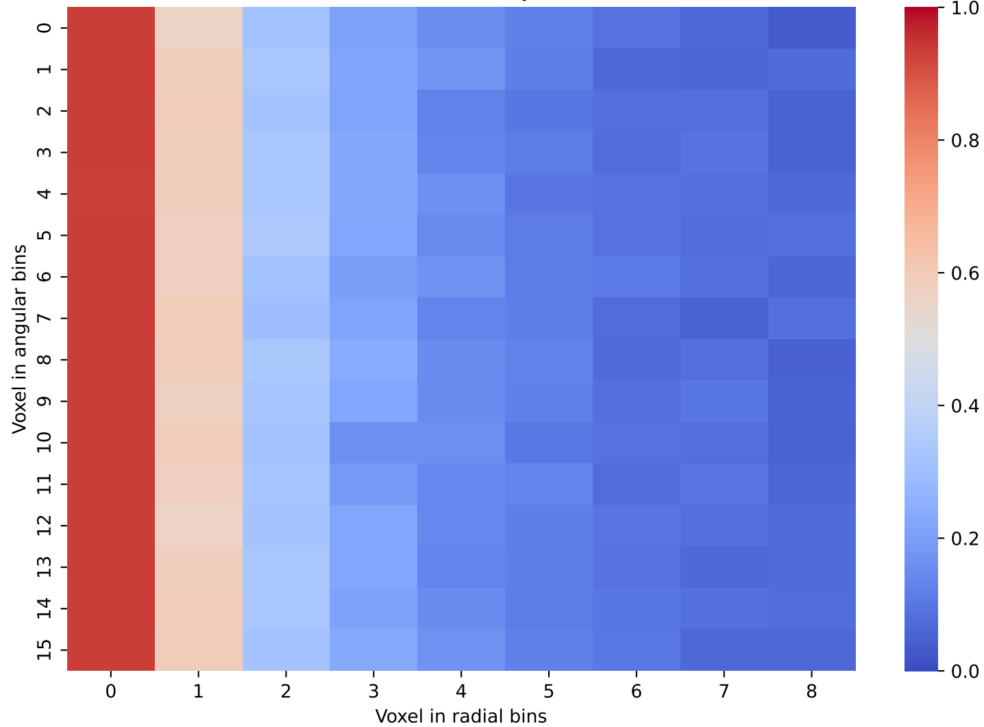
CaloDiffusion Data: Layer 7 and 8
