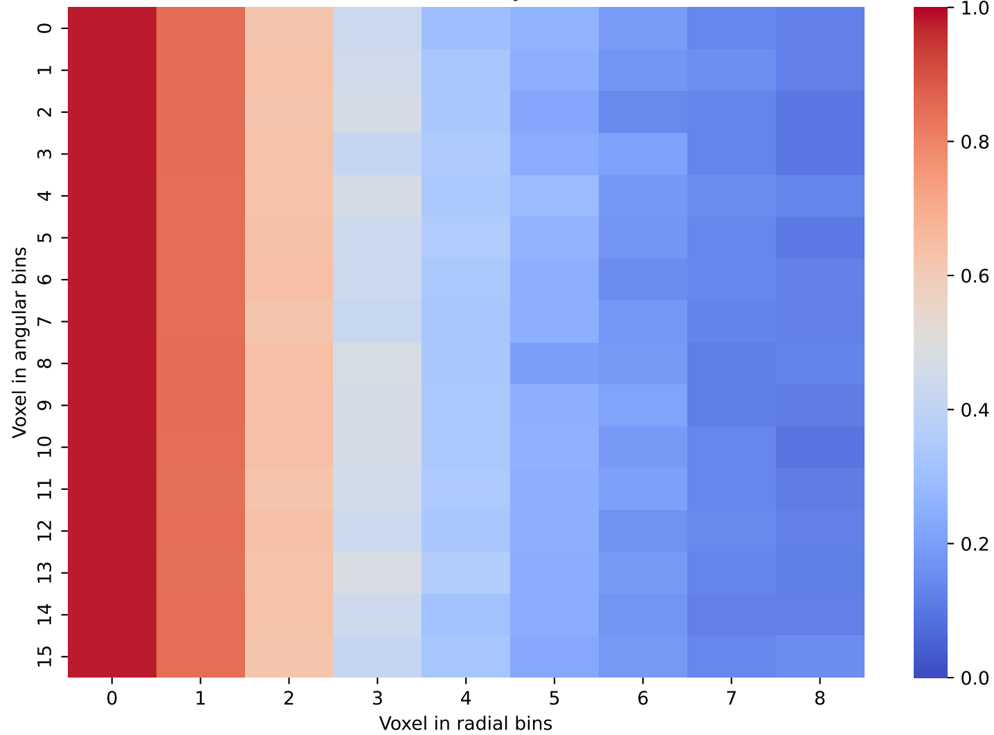
CaloDiffusion Data: Layer 12 and 13
