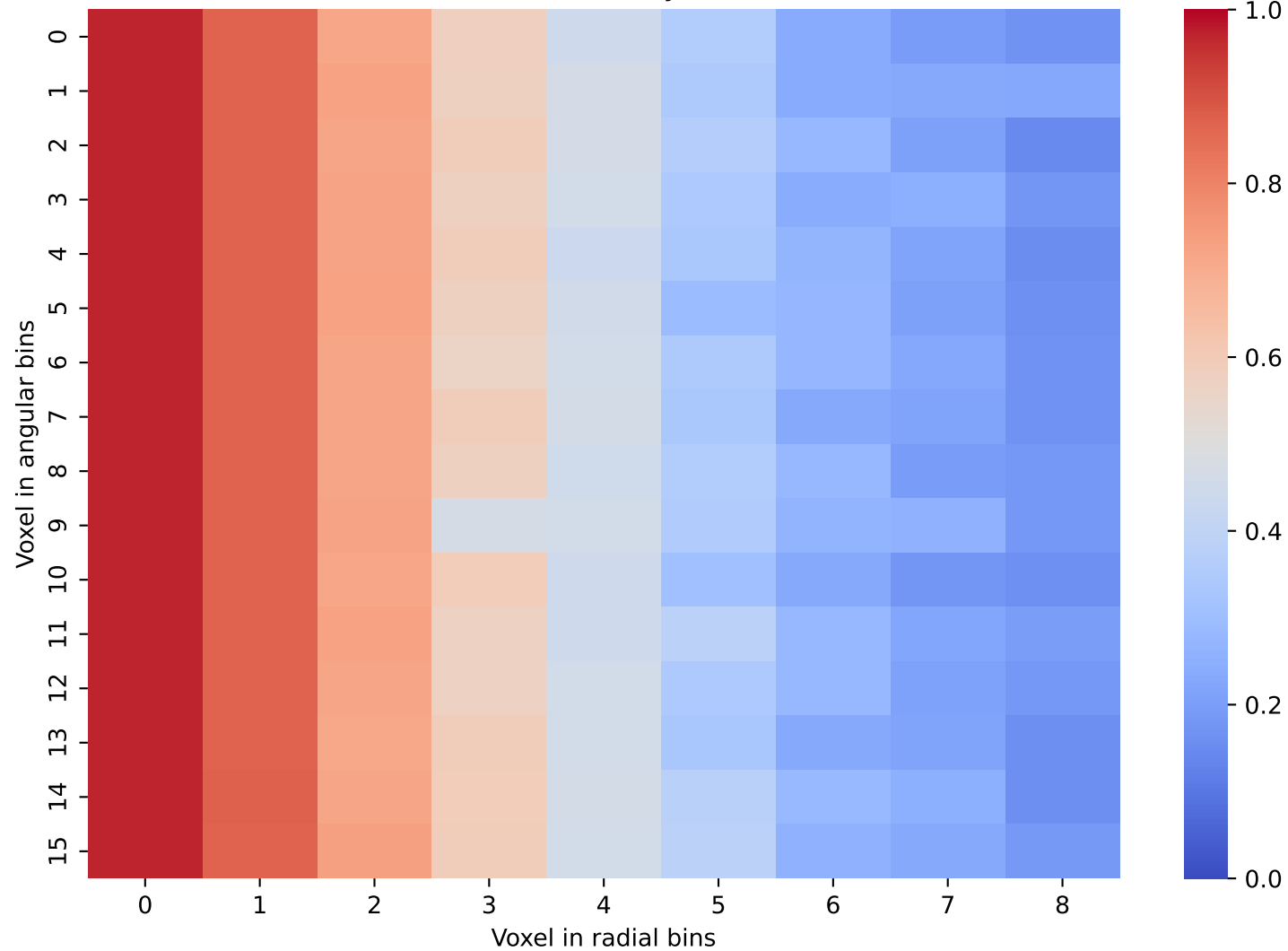
CaloDiffusion Data: Layer 19 and 20
