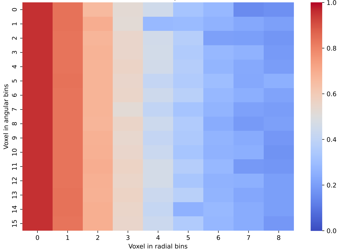
CaloDiffusion Data: Layer 22 and 23
