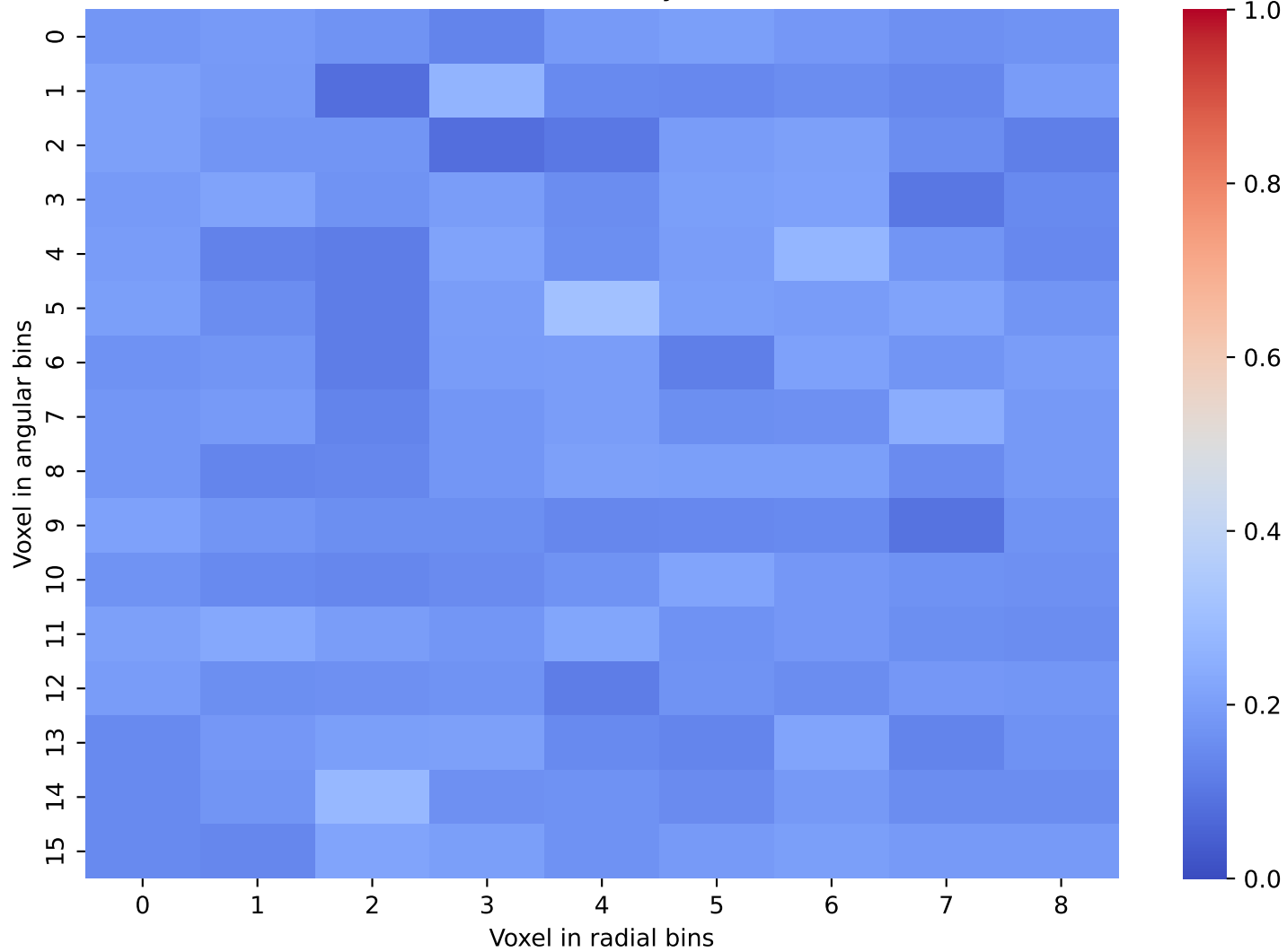
CaloDiffusion Data: Layer 41 and 42
