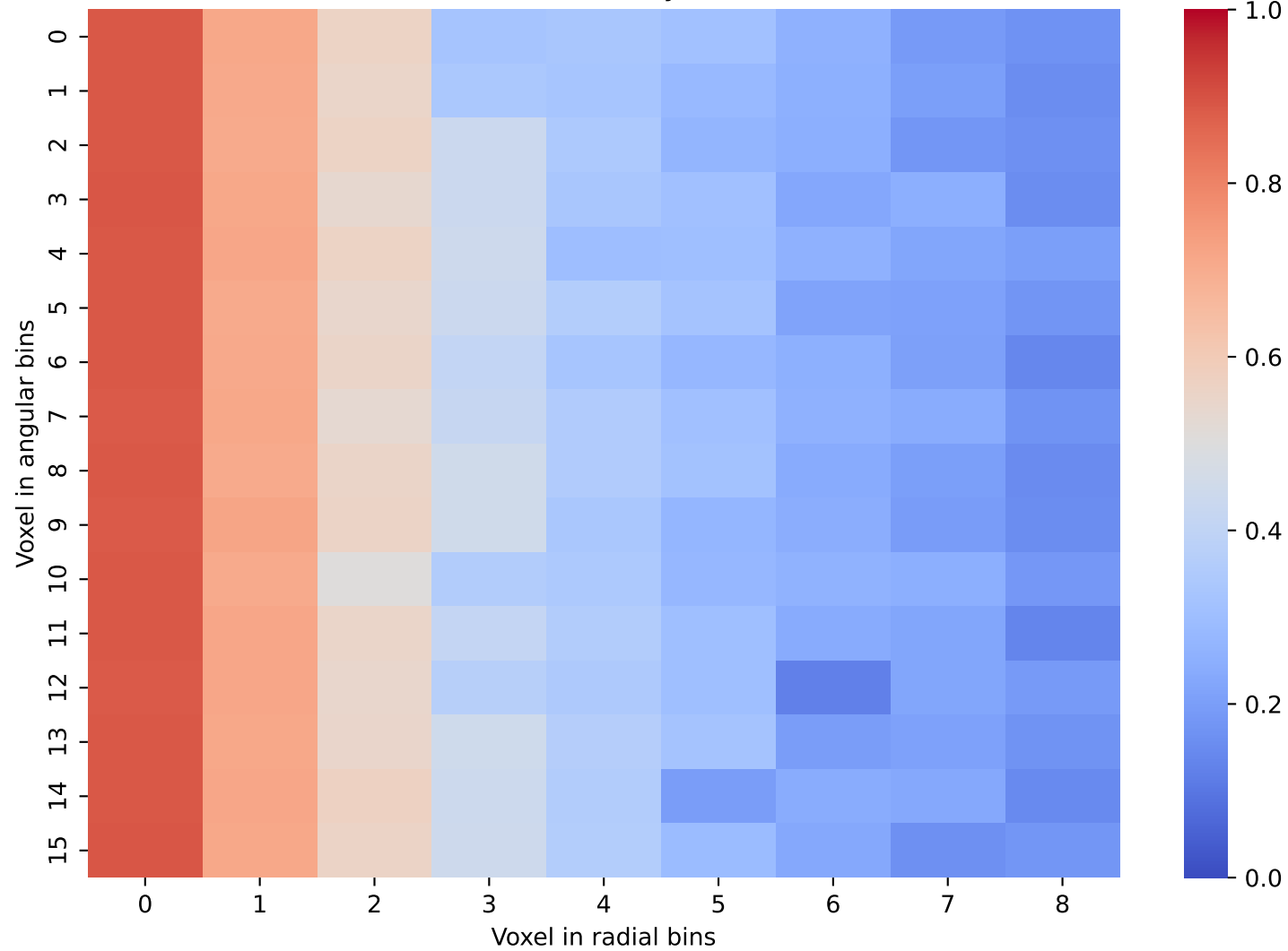
CaloDiffusion Data: Layer 27 and 28
