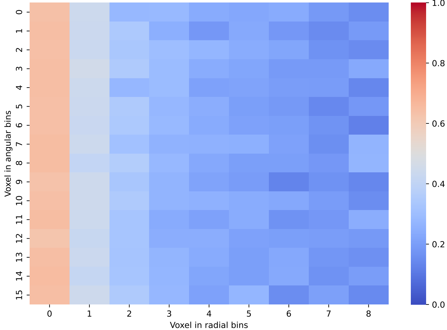
CaloDiffusion Data: Layer 33 and 34
