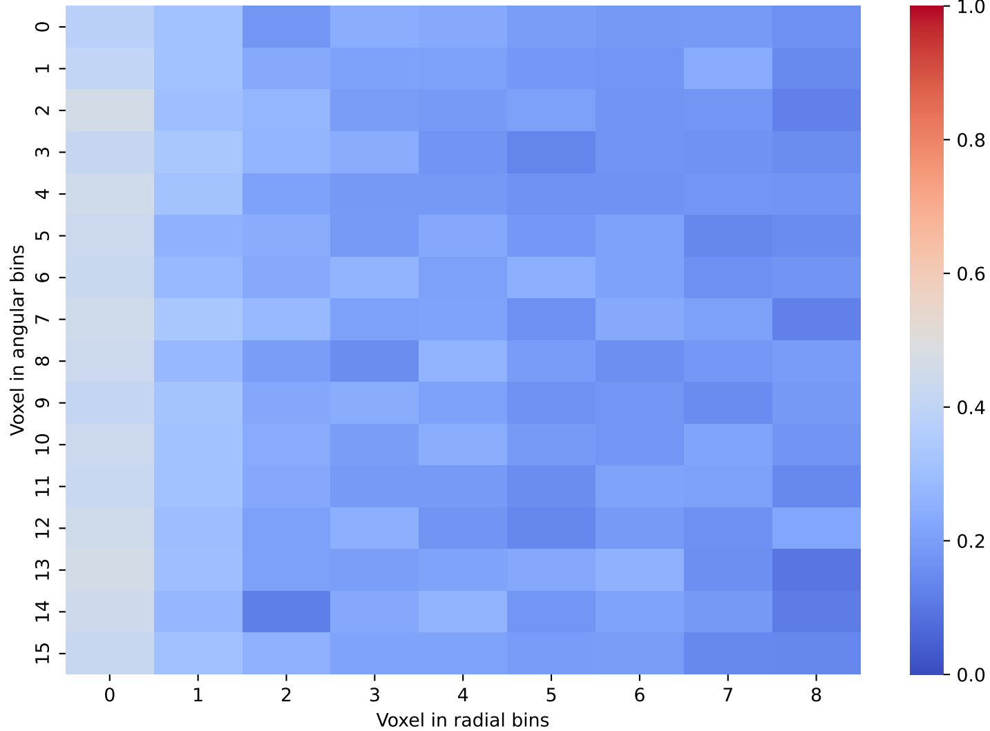
CaloDiffusion Data: Layer 36 and 37
