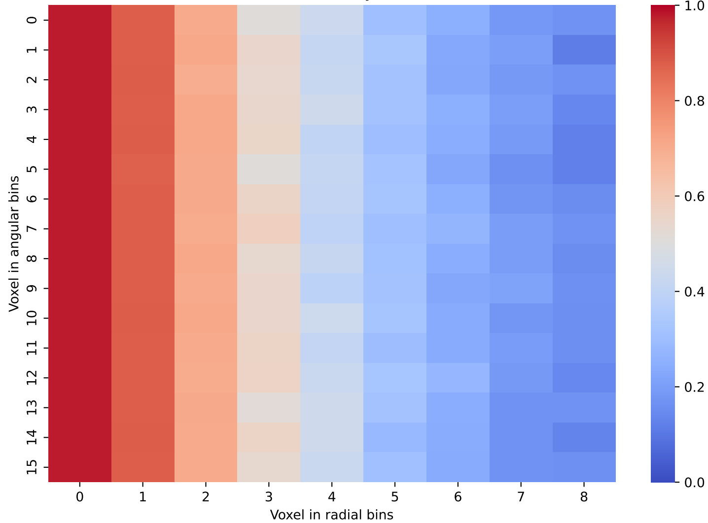
CaloDiffusion Data: Layer 15 and 16
