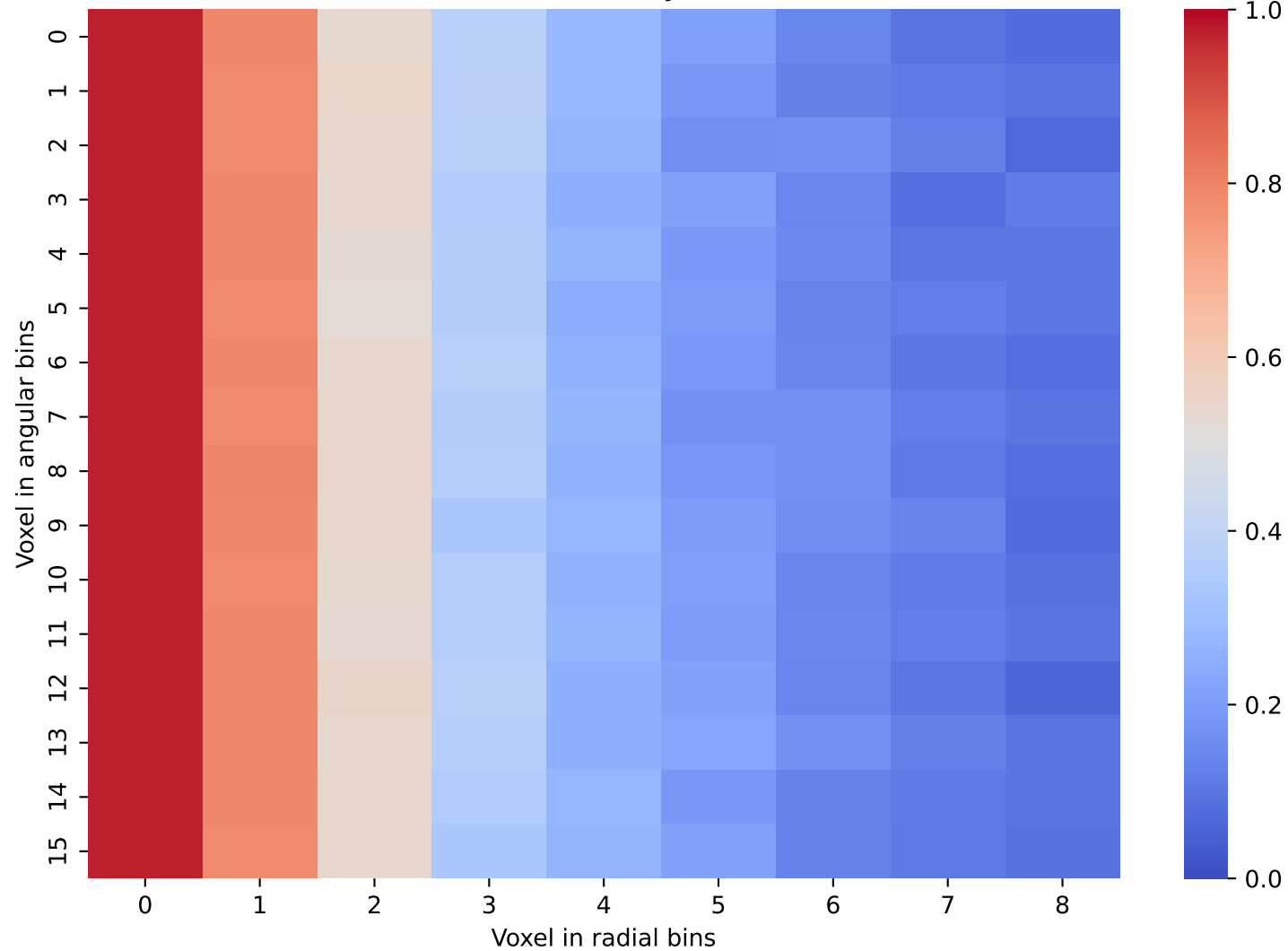
CaloDiffusion Data: Layer 10 and 11
