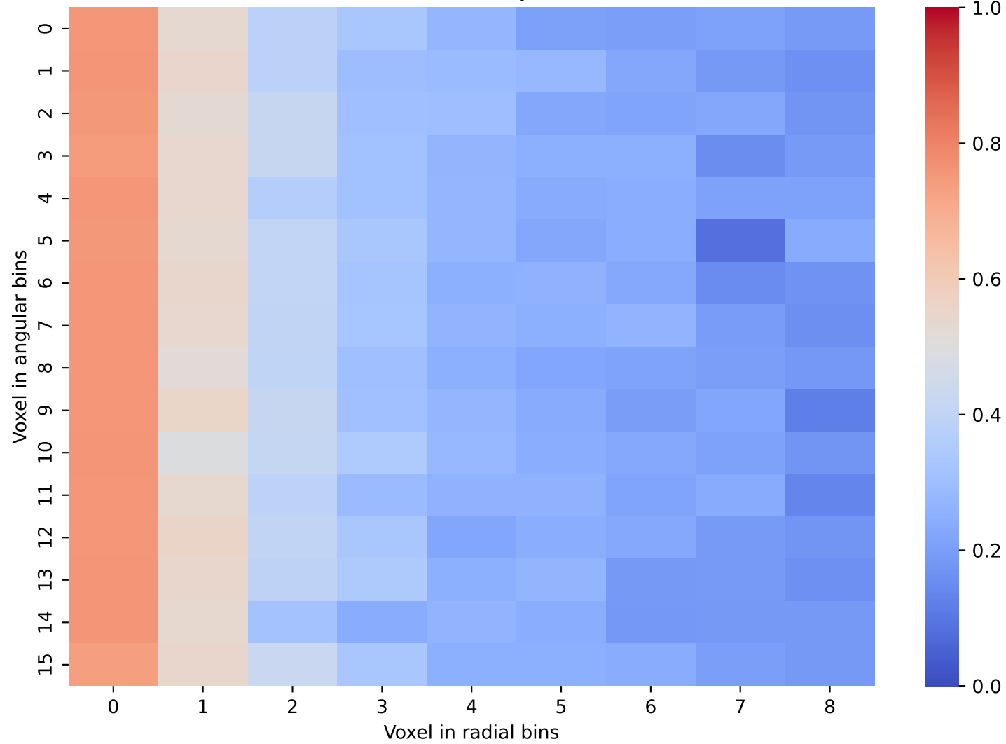
CaloDiffusion Data: Layer 31 and 32
