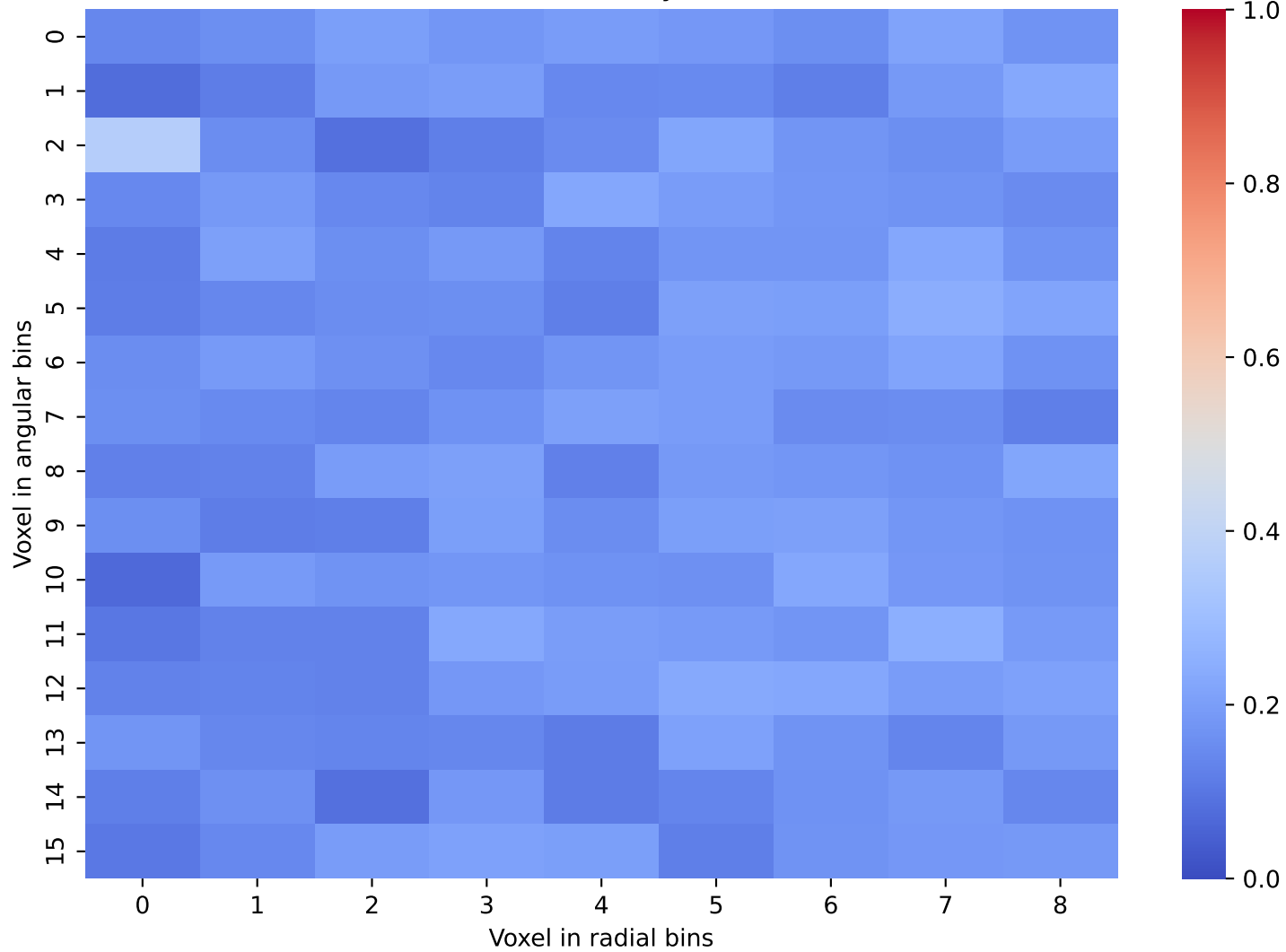
CaloDiffusion Data: Layer 44 and 45
