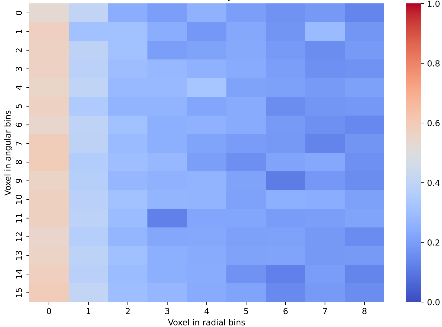
CaloDiffusion Data: Layer 34 and 35
