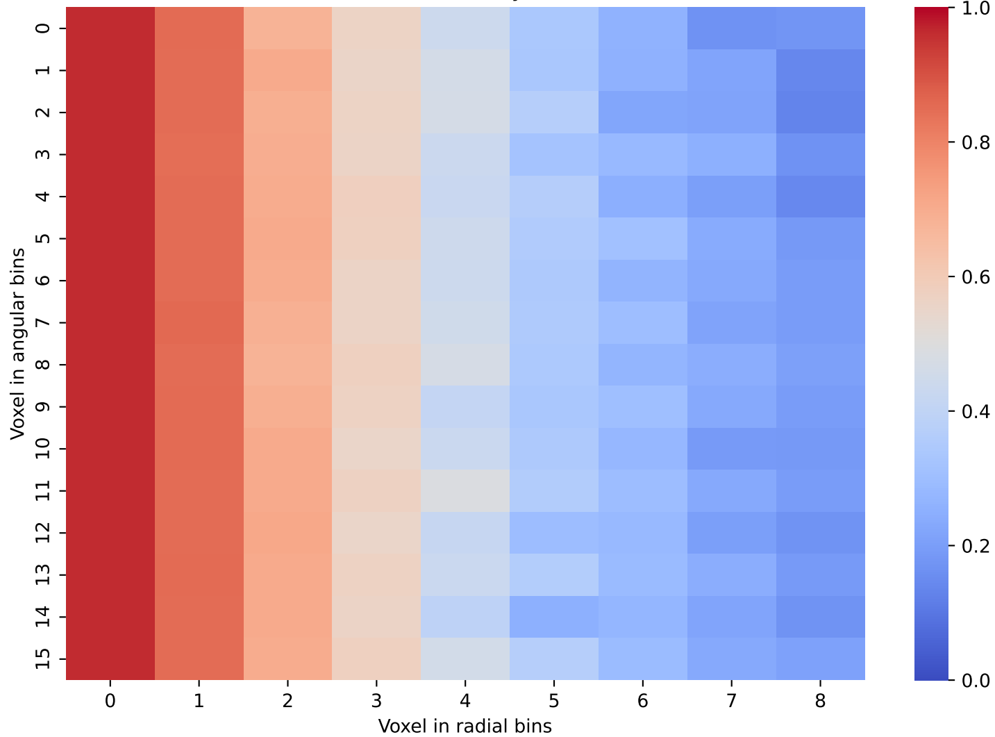
CaloDiffusion Data: Layer 21 and 22
