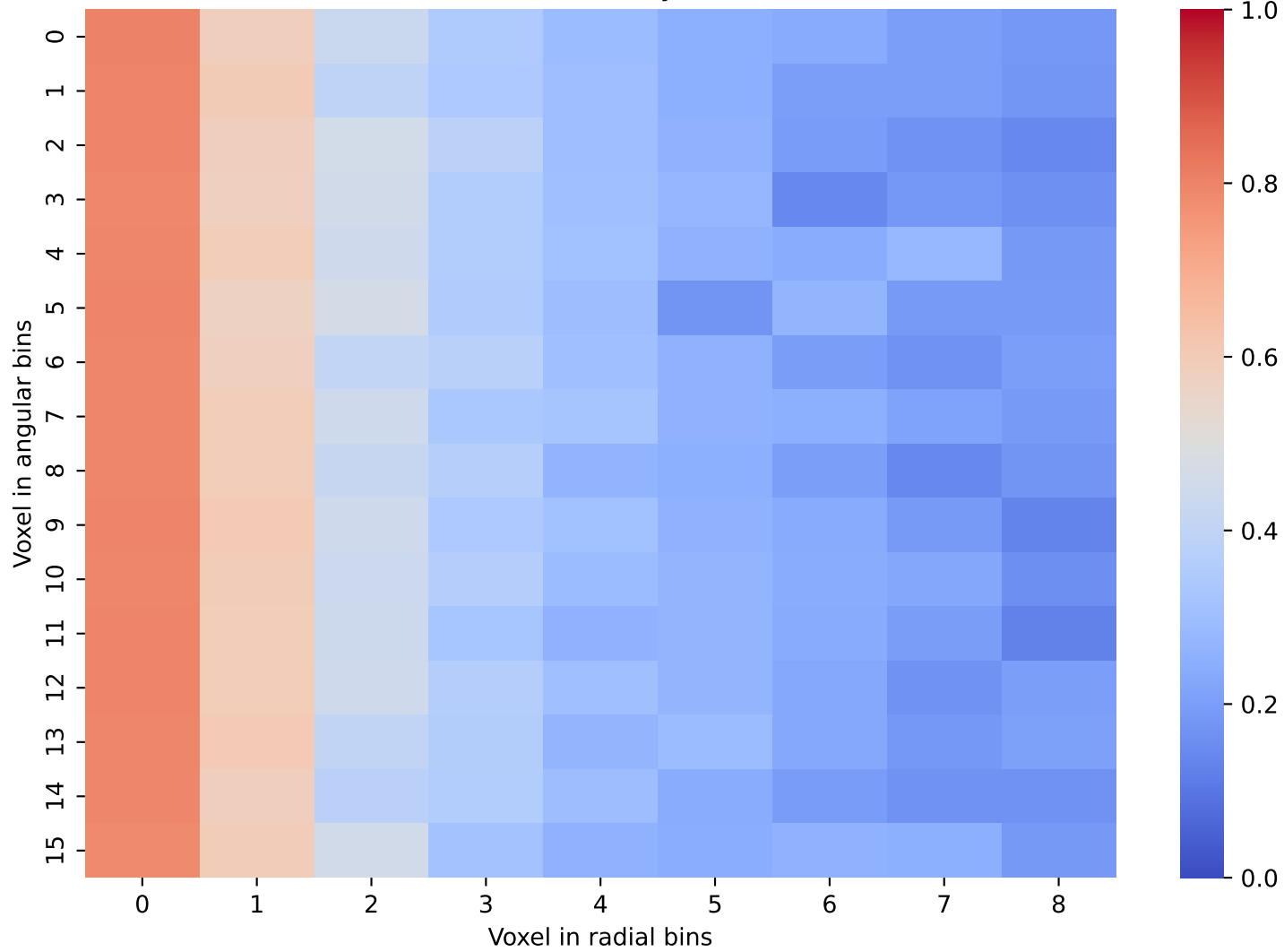
CaloDiffusion Data: Layer 30 and 31
