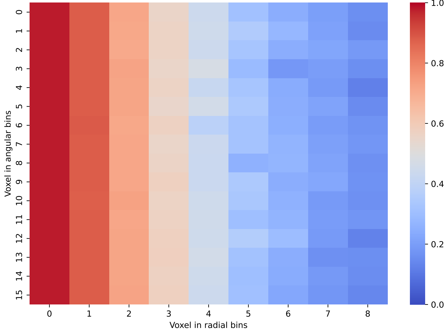
CaloDiffusion Data: Layer 16 and 17
