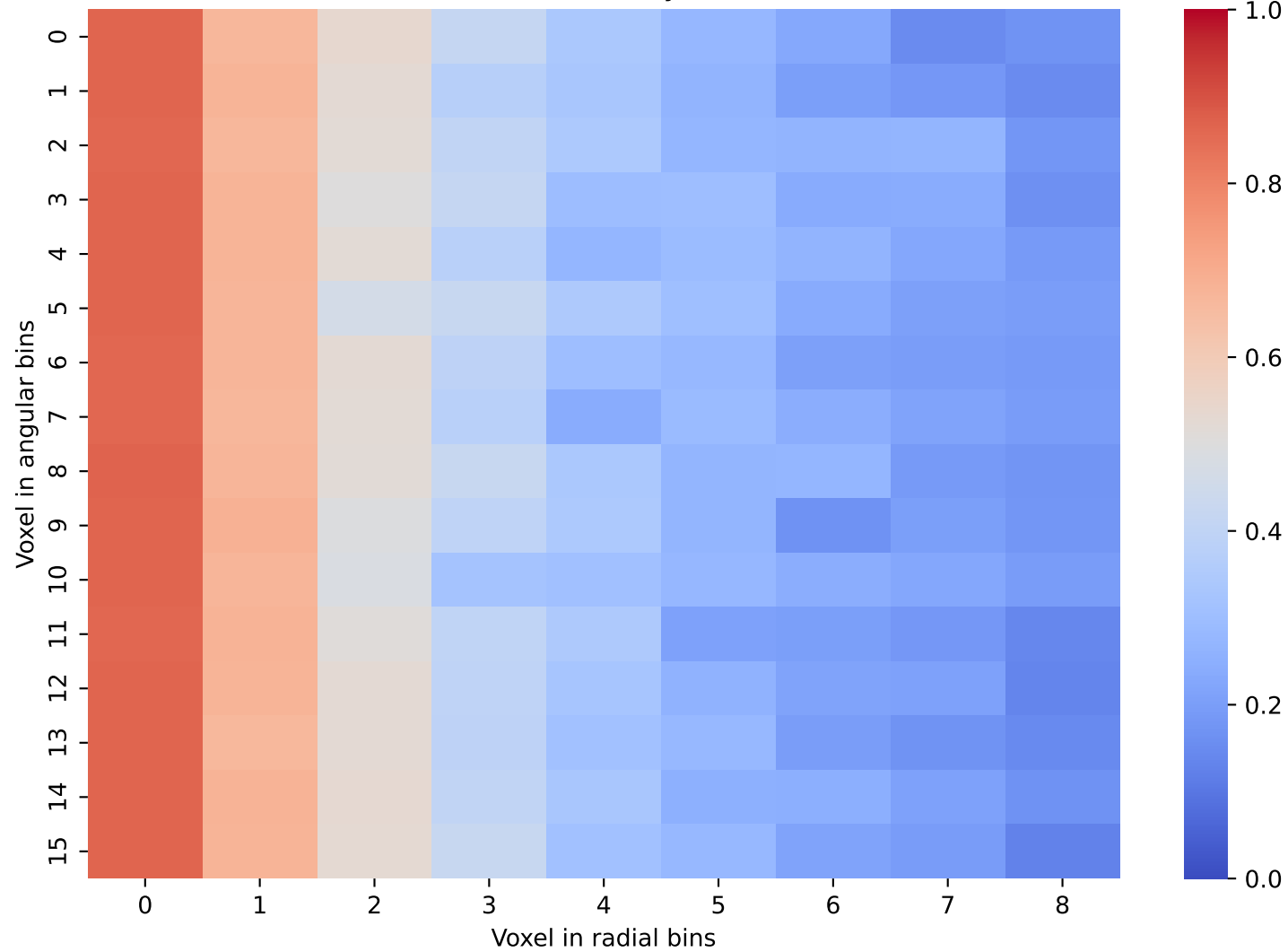
CaloDiffusion Data: Layer 28 and 29
