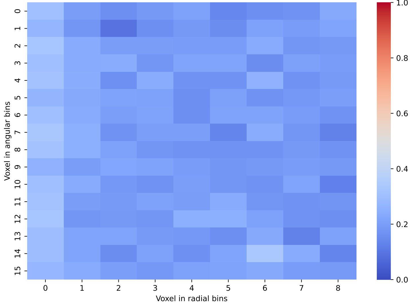
CaloDiffusion Data: Layer 38 and 39
