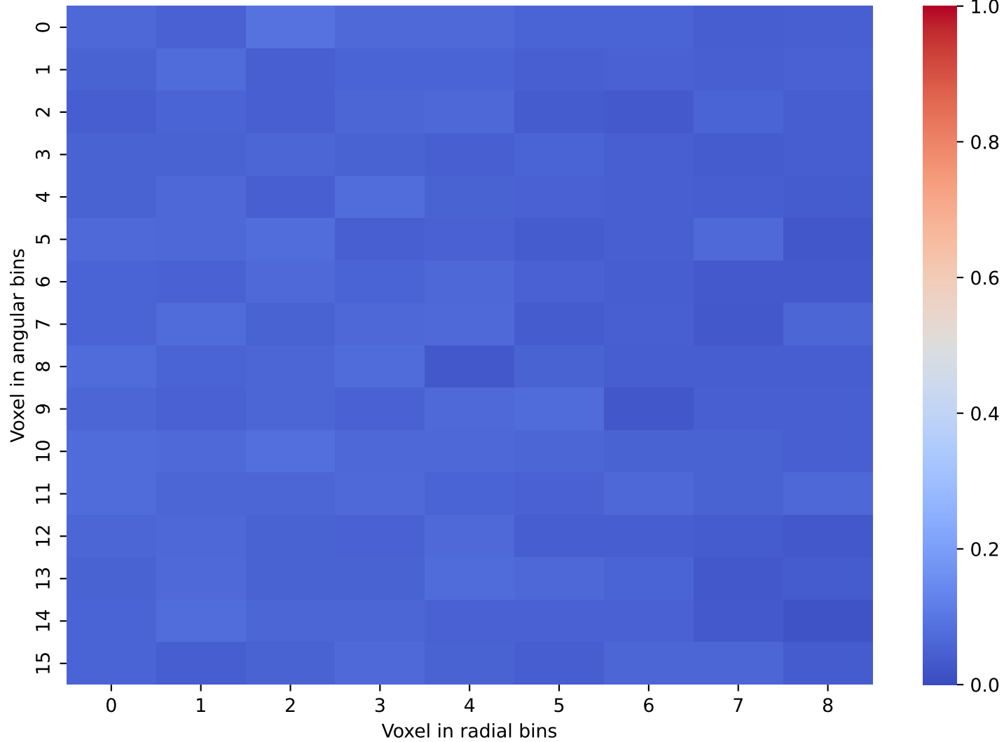
CaloDiffusion Data: Layer 1 and 2
