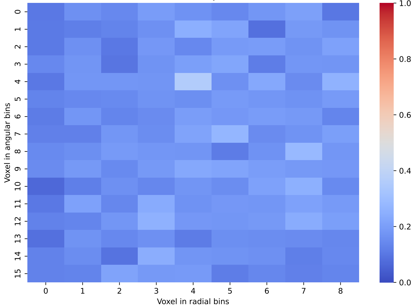
CaloDiffusion Data: Layer 43 and 44
