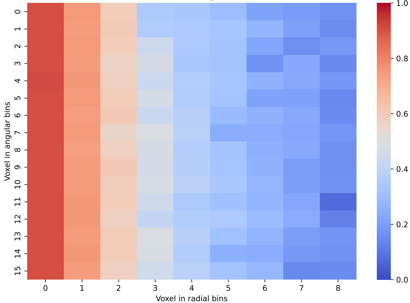
CaloDiffusion Data: Layer 26 and 27
