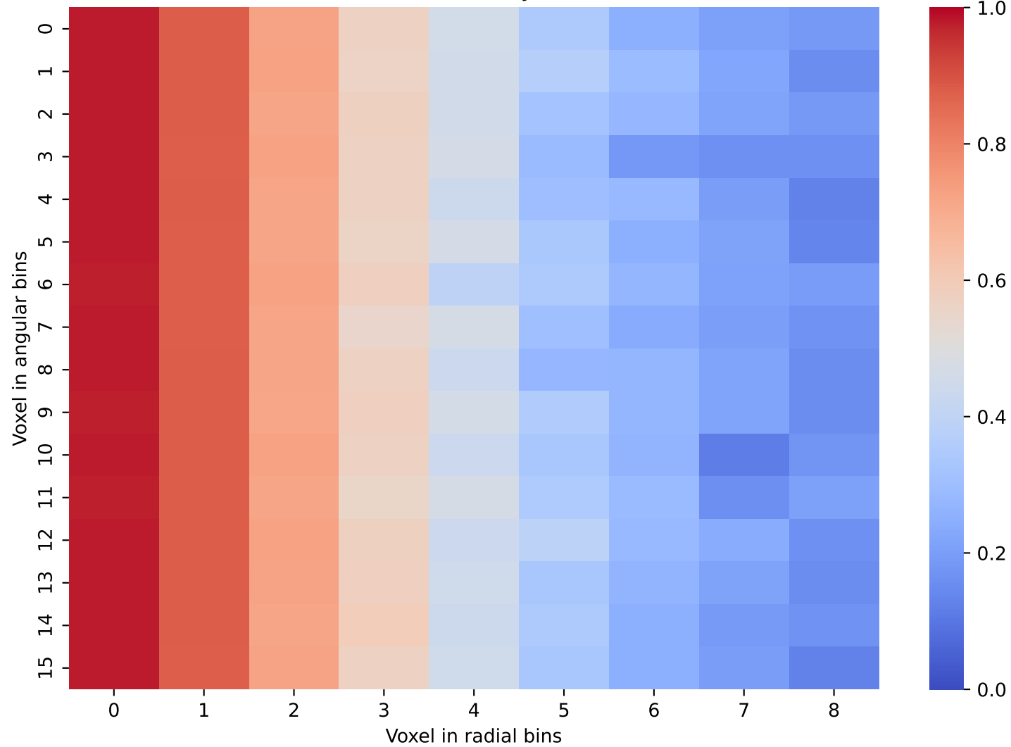
CaloDiffusion Data: Layer 17 and 18
