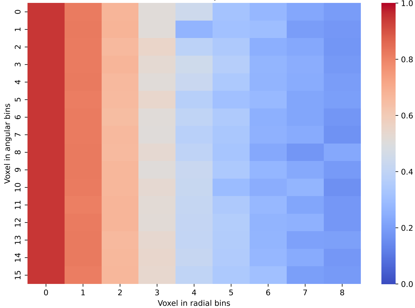
CaloDiffusion Data: Layer 23 and 24
