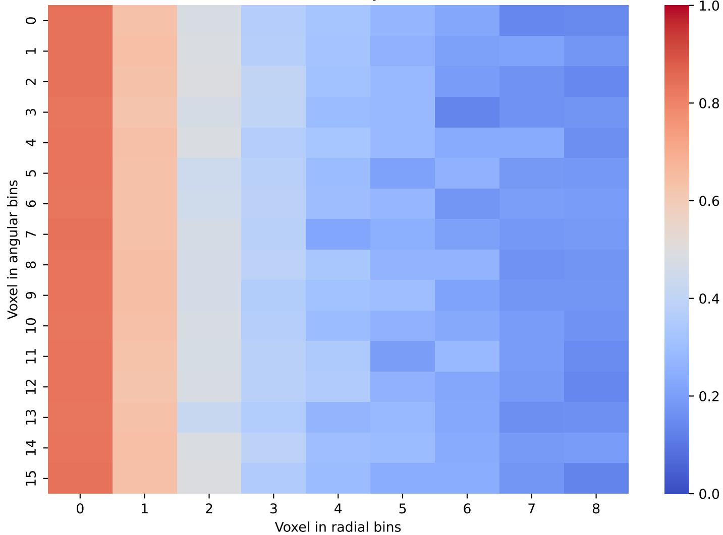
CaloDiffusion Data: Layer 29 and 30
