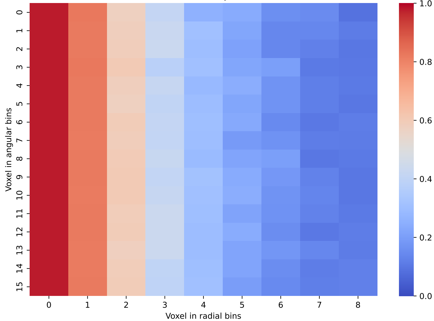
CaloDiffusion Data: Layer 11 and 12
