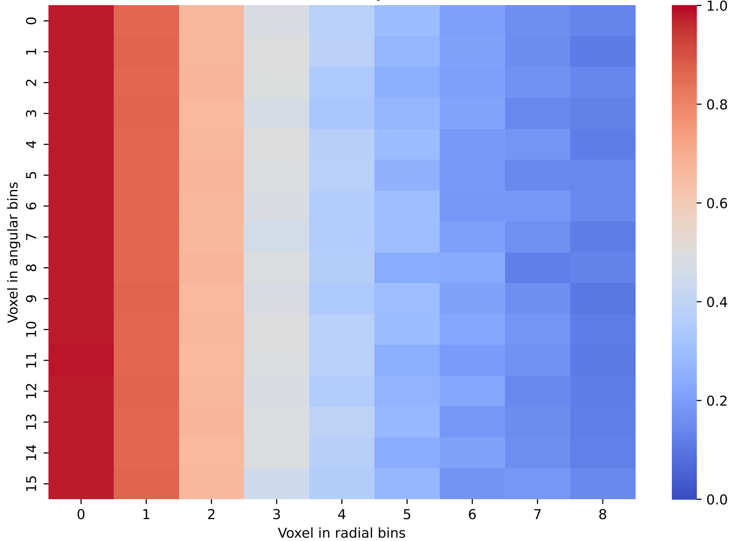
CaloDiffusion Data: Layer 13 and 14
