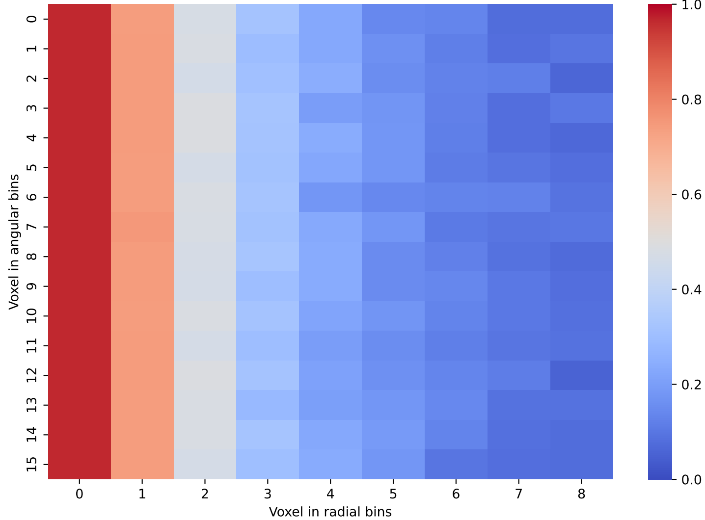
CaloDiffusion Data: Layer 9 and 10
