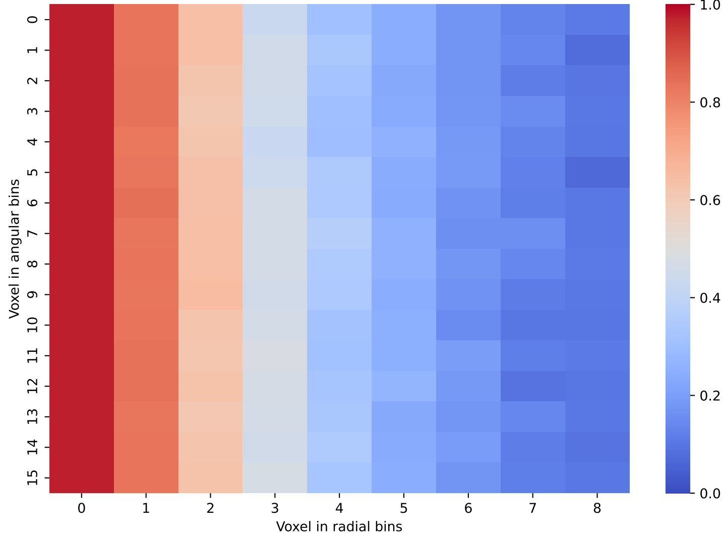
CaloDream Data: Layer 12 and 13
