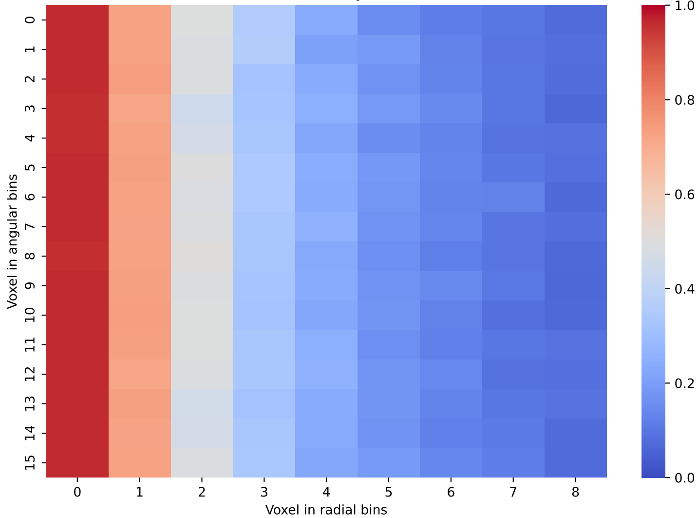
CaloDREAM Data: Layer 9 and 10
