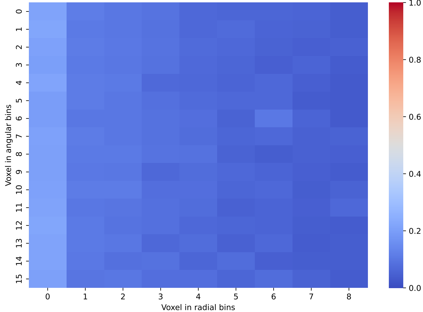
CaloDREAM Data: Layer 2 and 3
