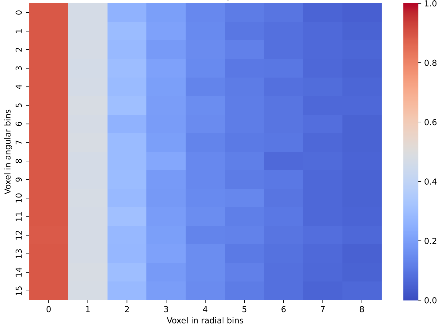
CaloDREAM Data: Layer 6 and 7
