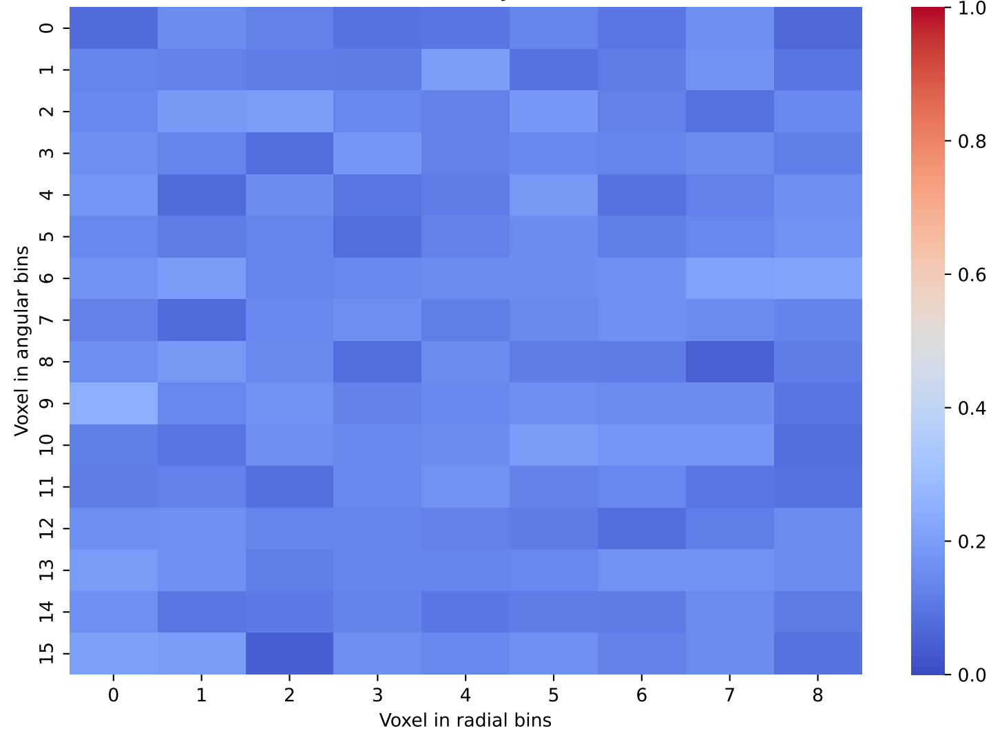
CaloDream Data: Layer 44 and 45
