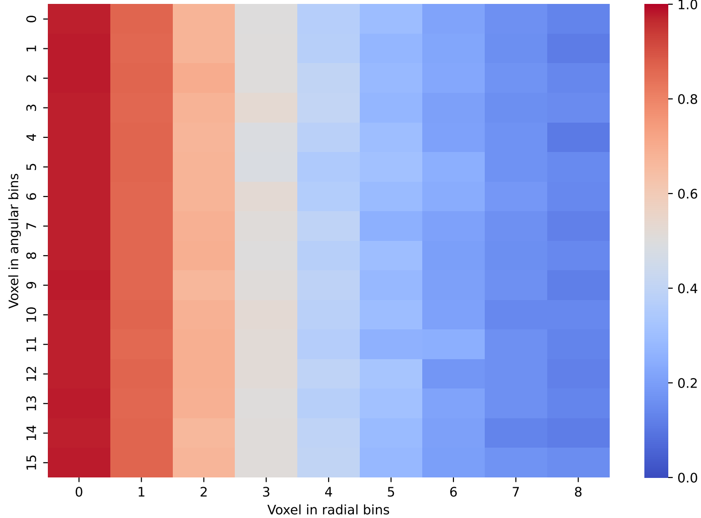
CaloDream Data: Layer 14 and 15
