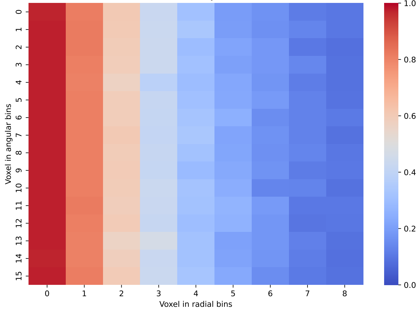
CaloDream Data: Layer 11 and 12
