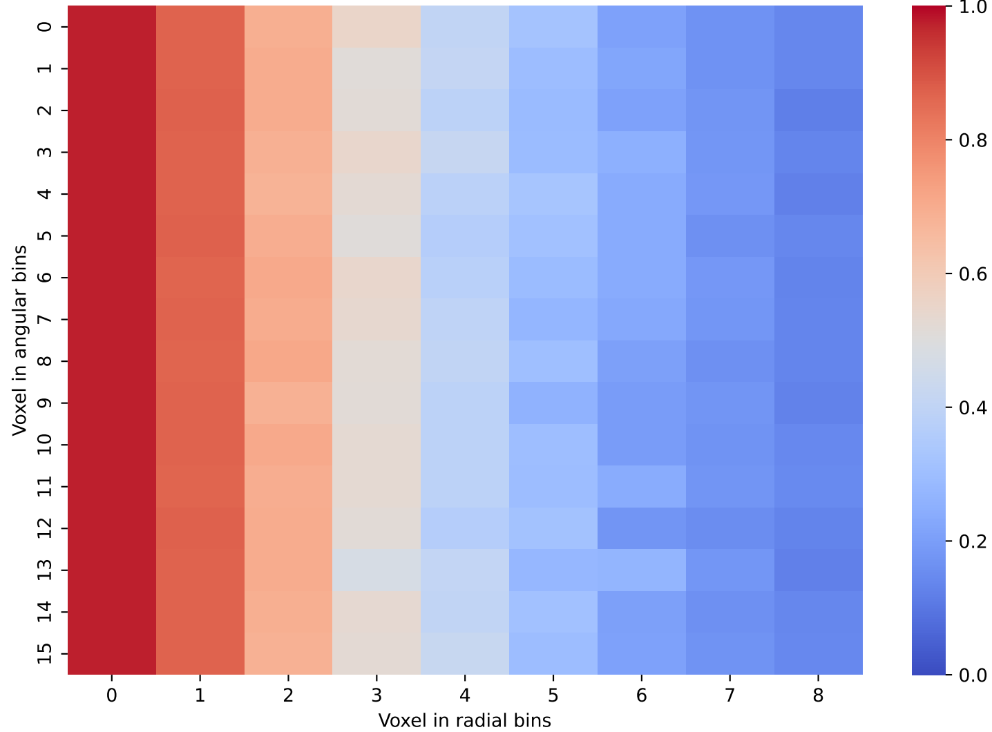
CaloDream Data: Layer 15 and 16
