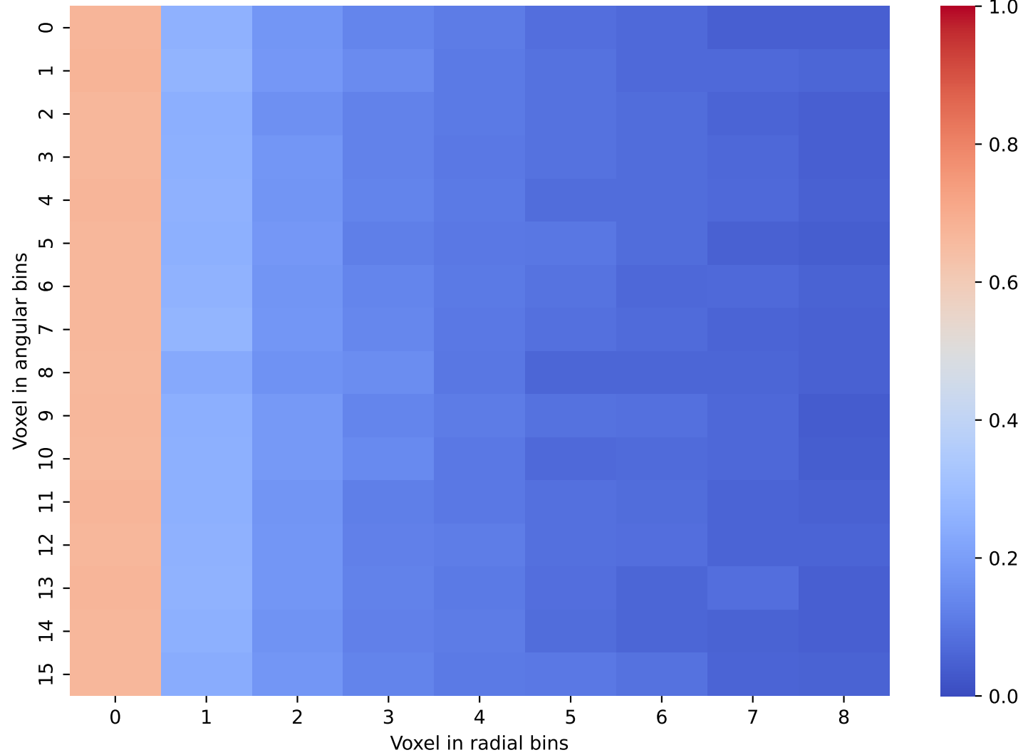
CaloDREAM Data: Layer 4 and 5
