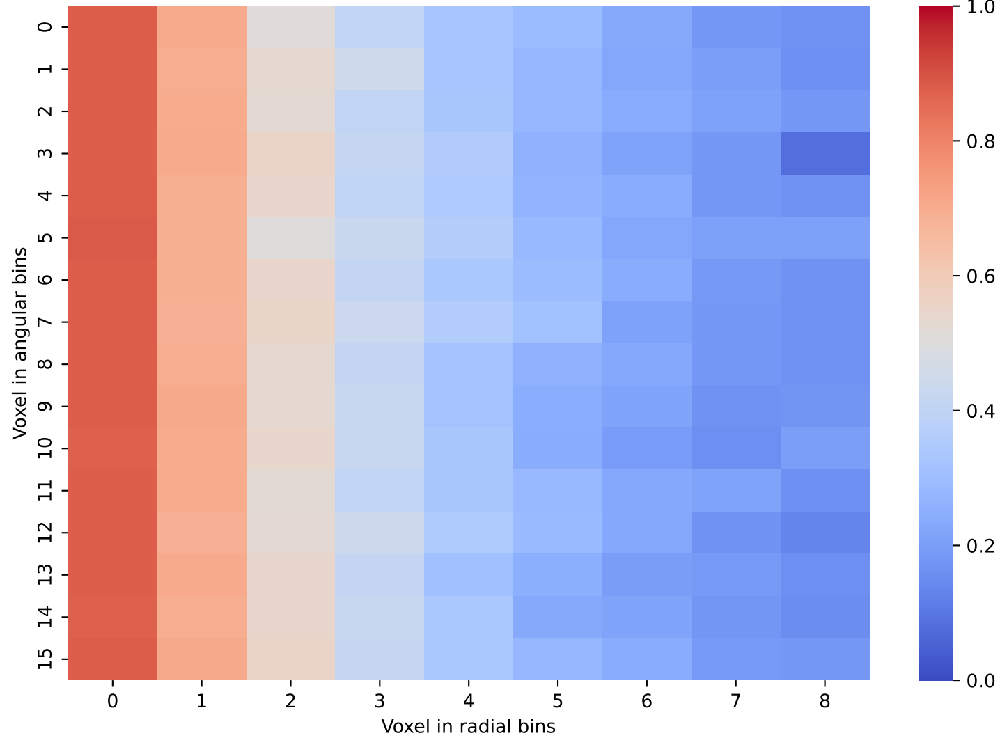
CaloDream Data: Layer 27 and 28
