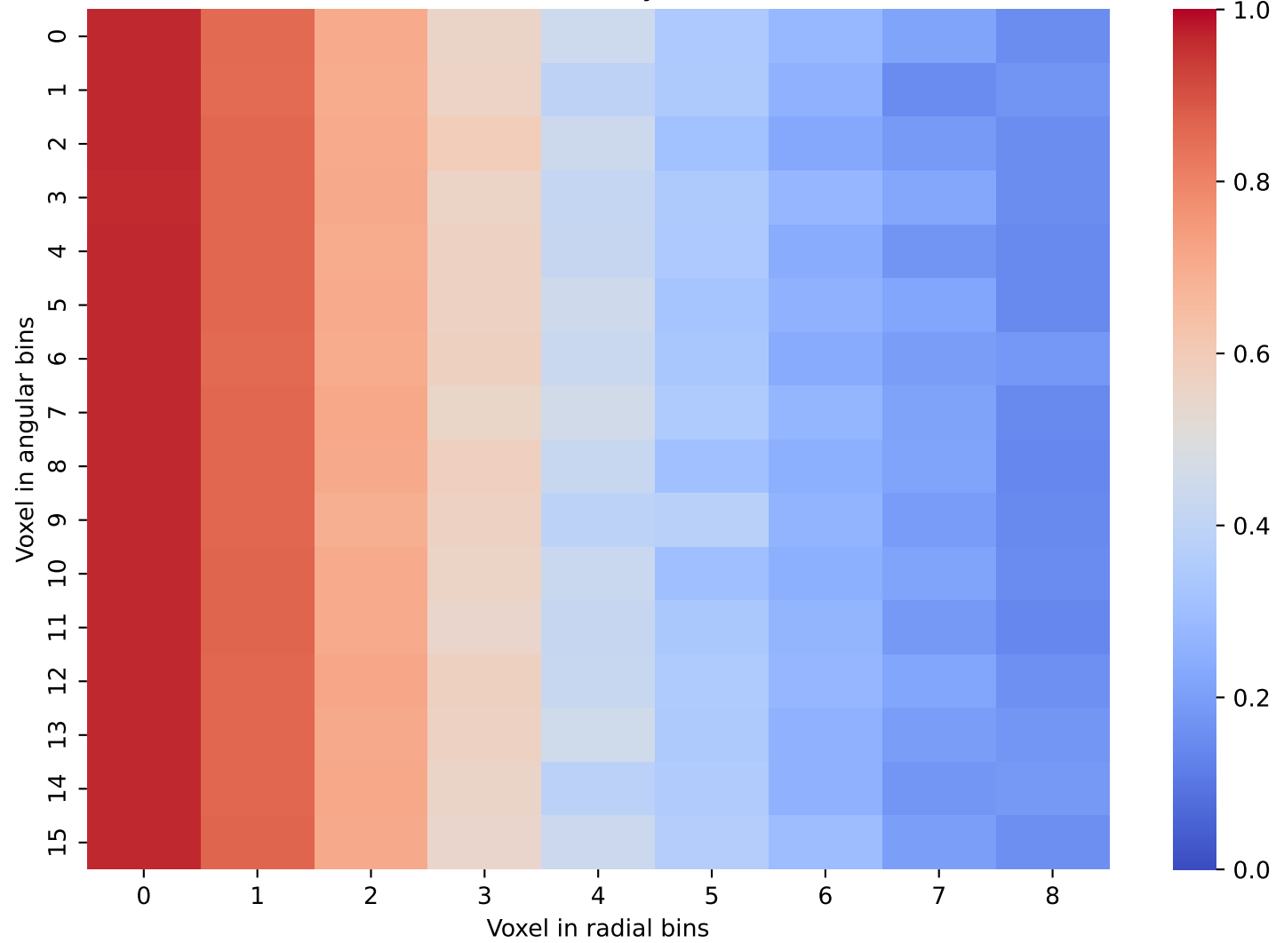
CaloDream Data: Layer 19 and 20
