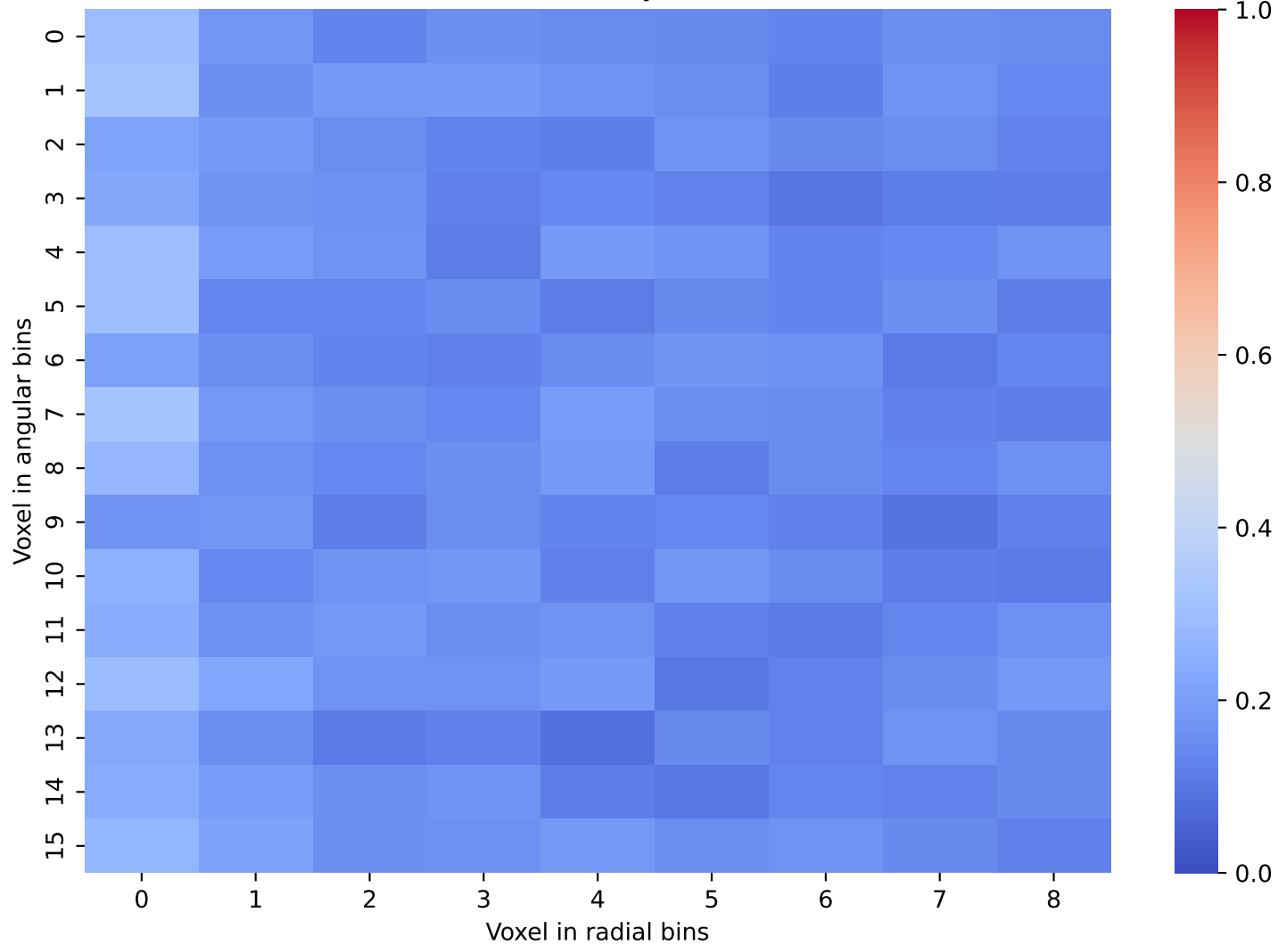
CaloDREAM Data: Layer 40 and 41
