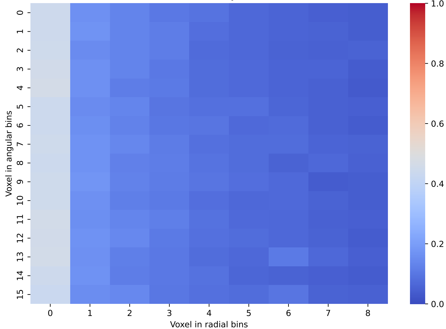
CaloDREAM Data: Layer 3 and 4
