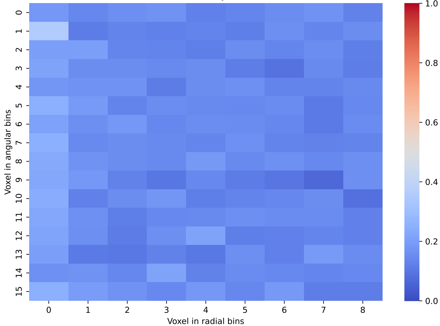
CaloDream Data: Layer 41 and 42
