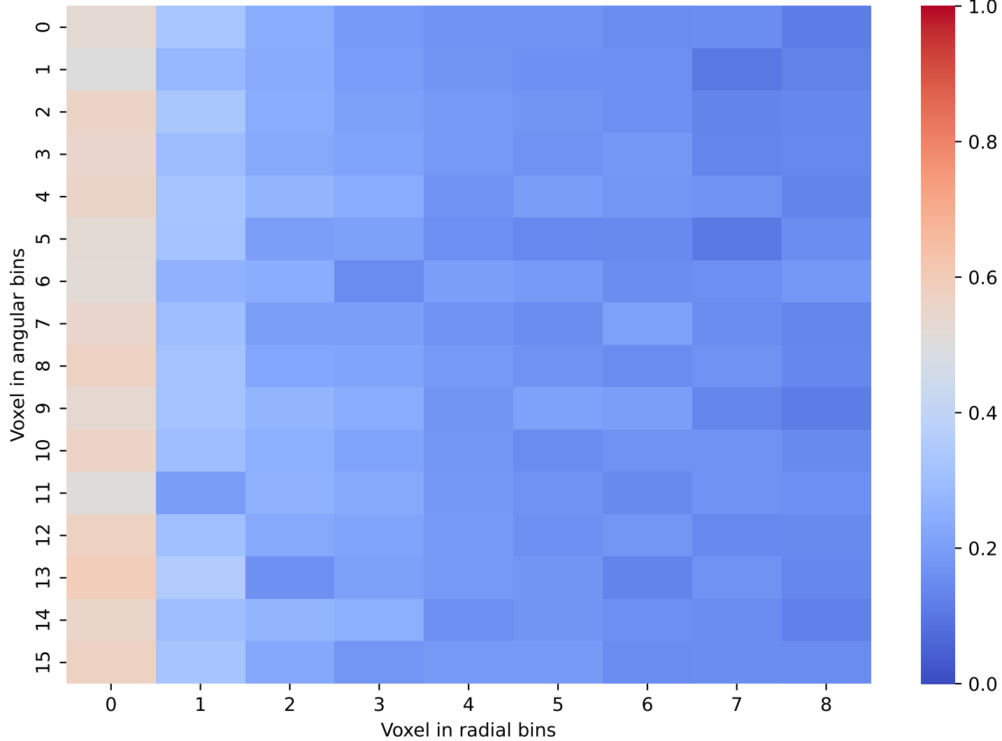
CaloDream Data: Layer 35 and 36
