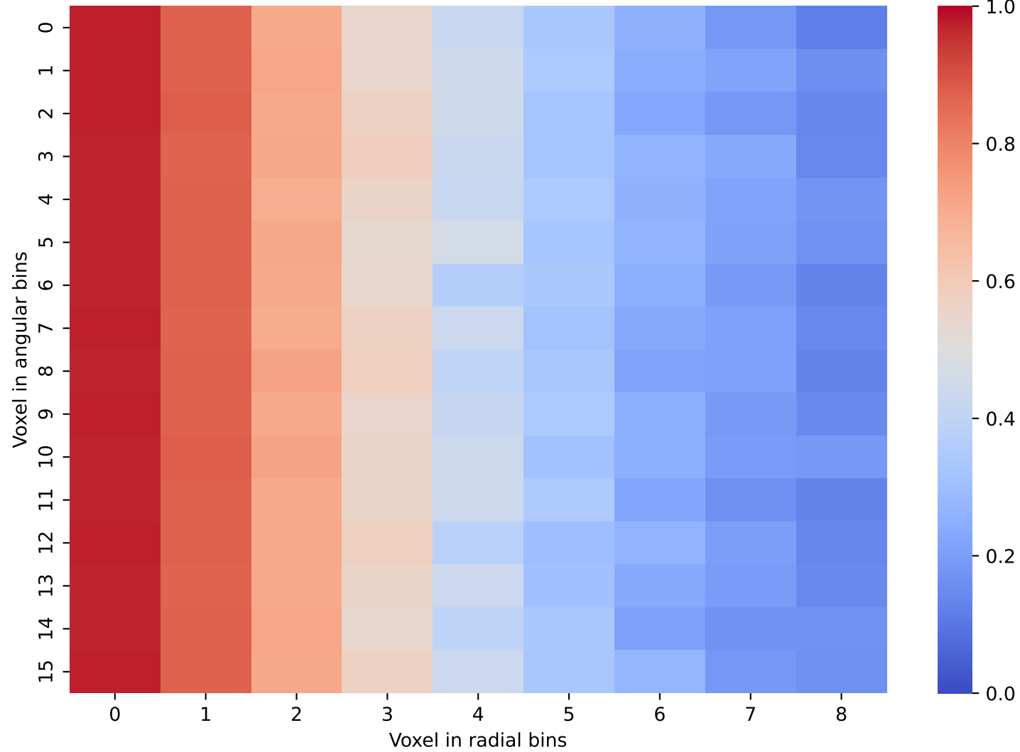
CaloDream Data: Layer 17 and 18
