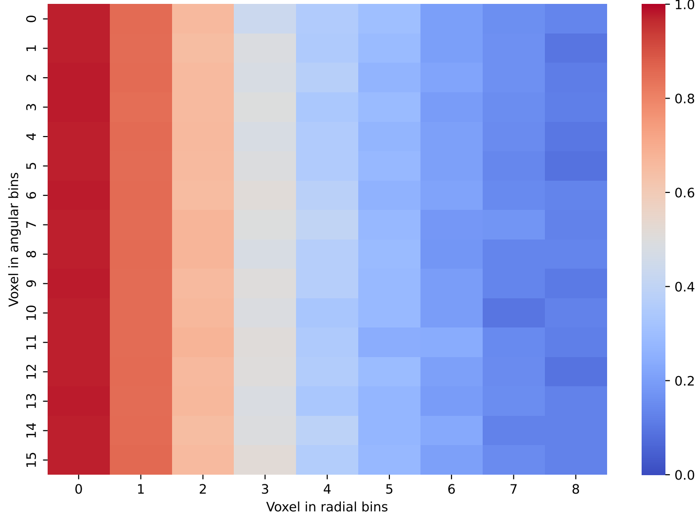
CaloDream Data: Layer 13 and 14
