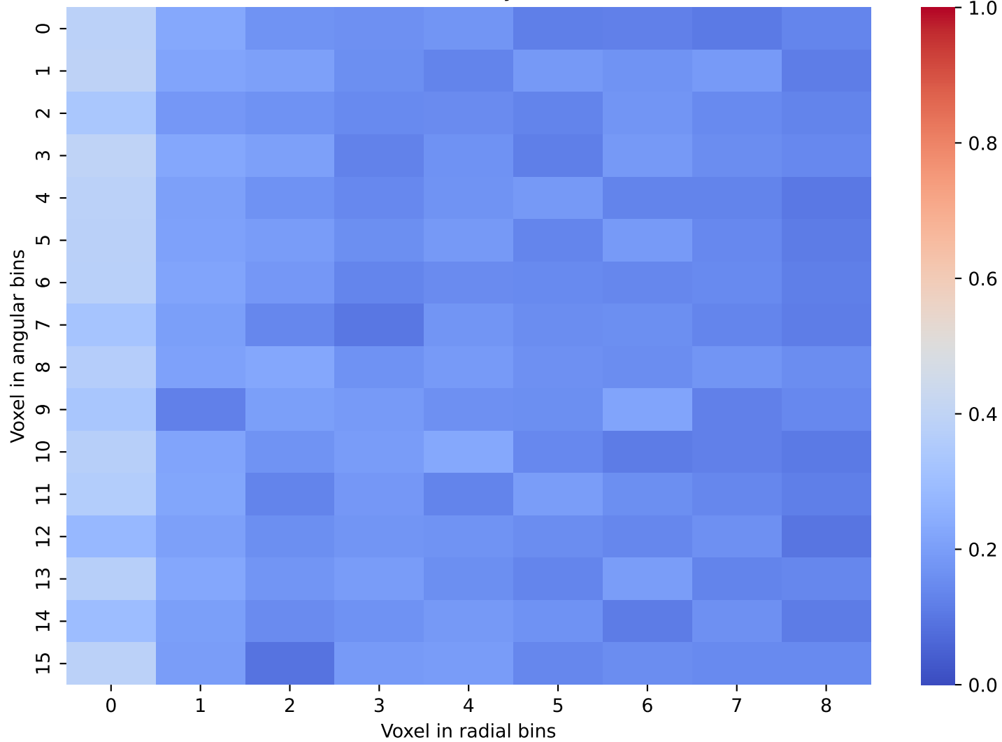
CaloDream Data: Layer 38 and 39
