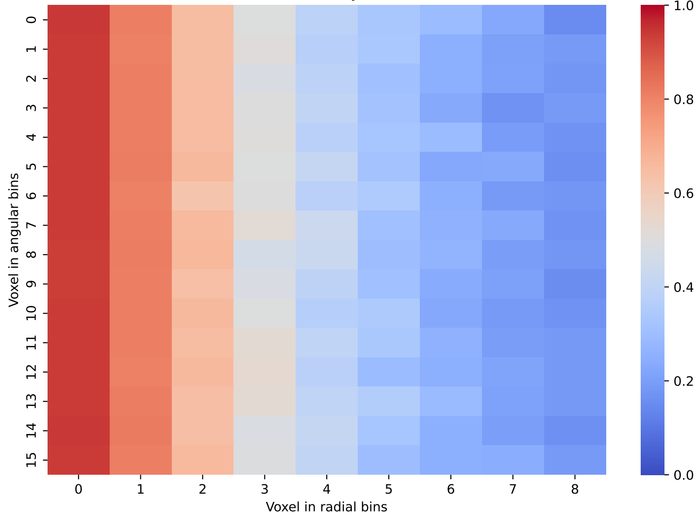
CaloDream Data: Layer 23 and 24
