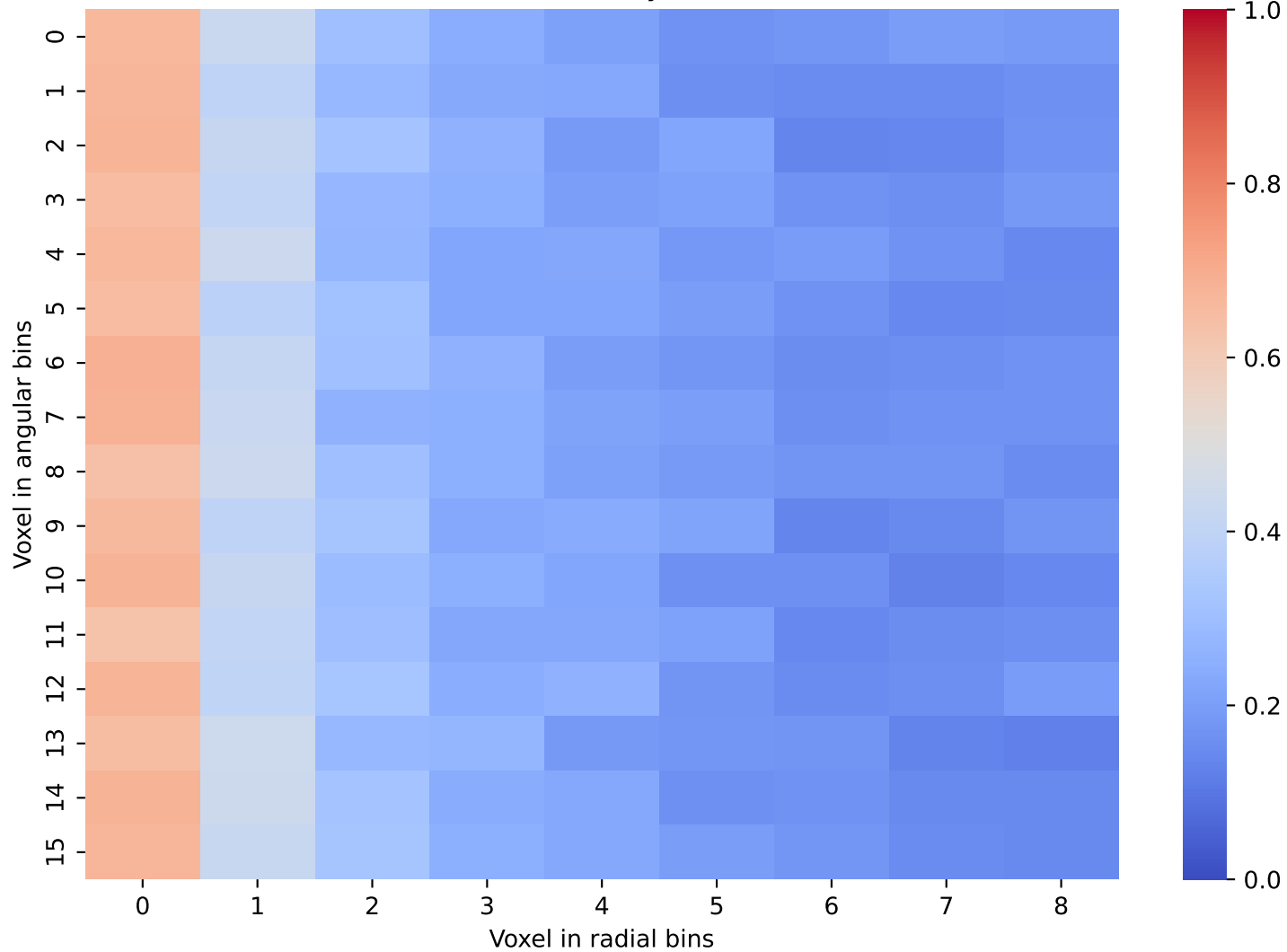
CaloDream Data: Layer 33 and 34
