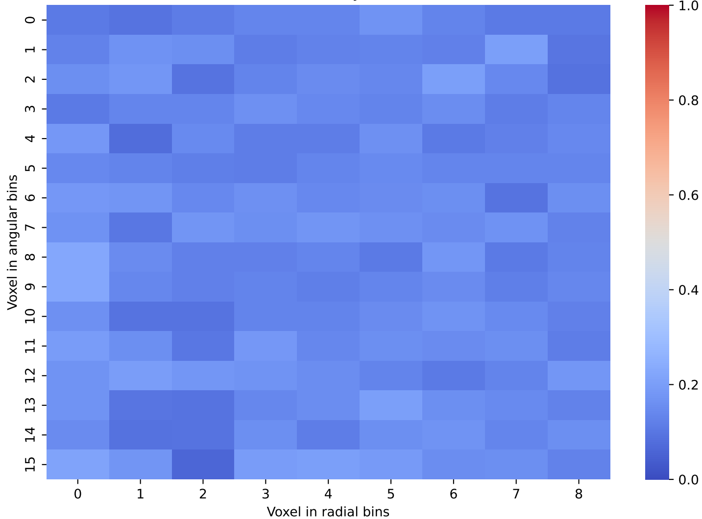
CaloDream Data: Layer 43 and 44
