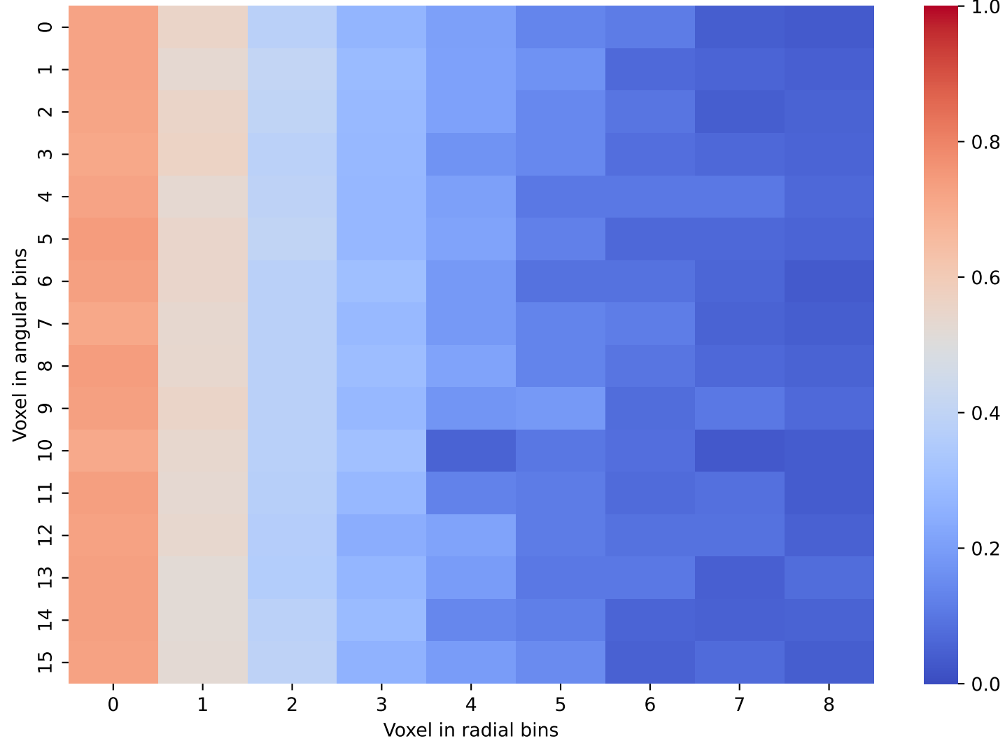
CaloINN Data: Layer 23 and 24
