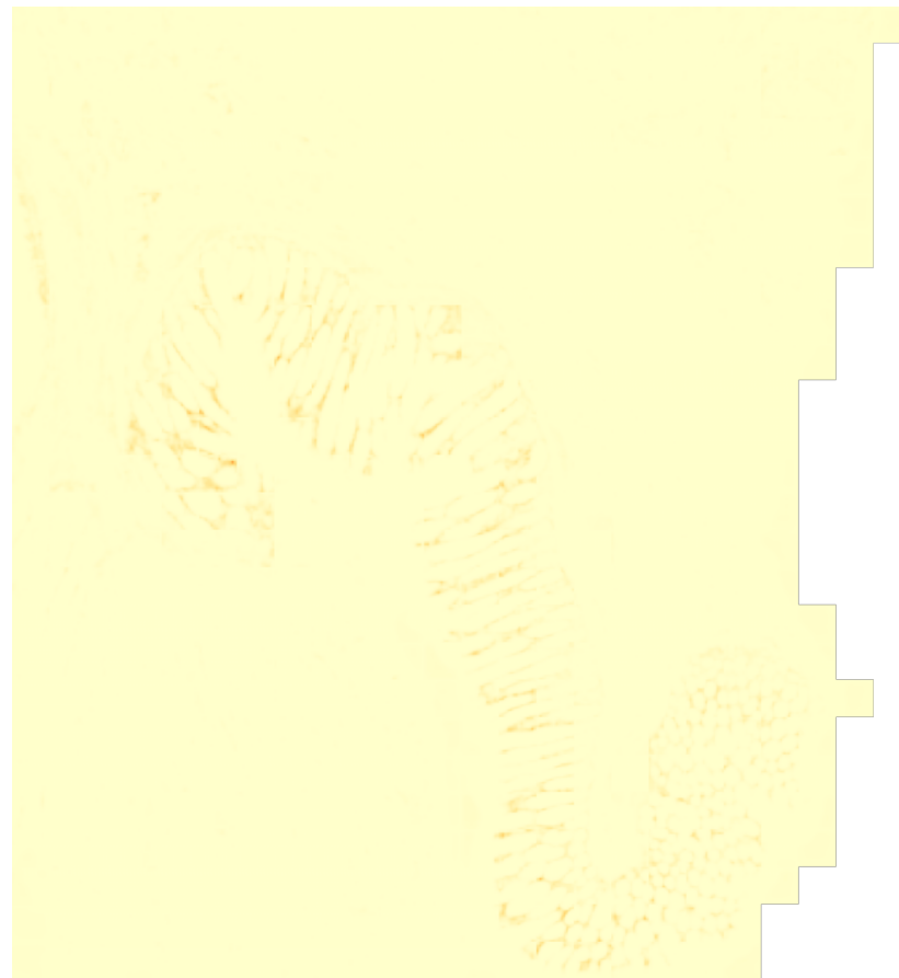
Model E (Poisson)
