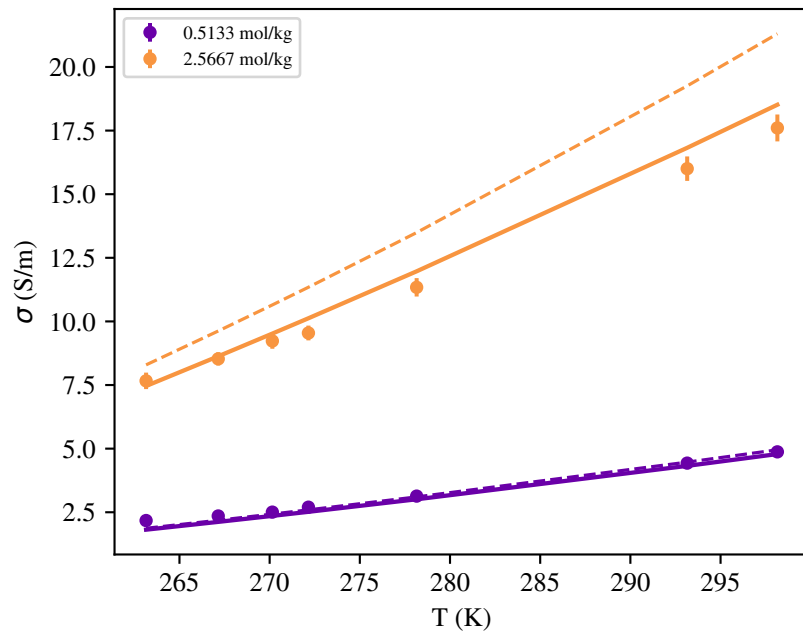
NaCl
