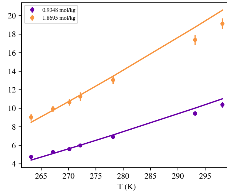
NH4Cl
