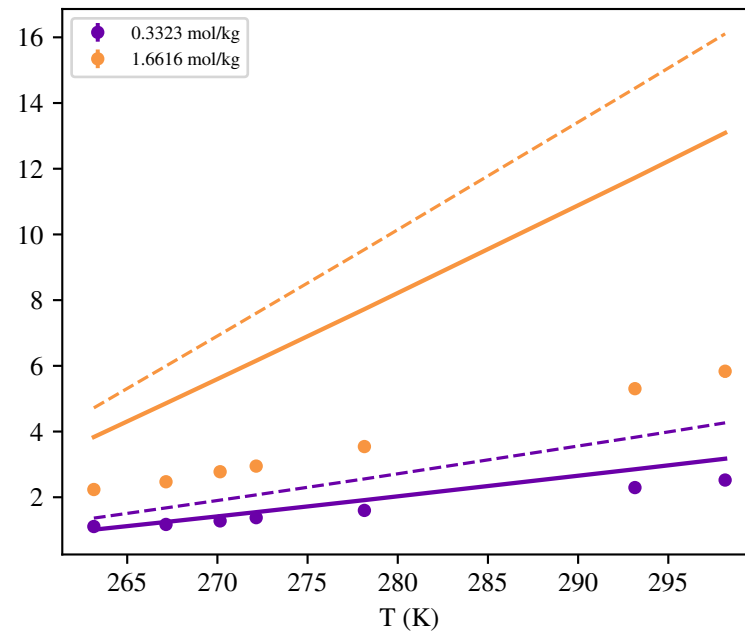
MgSO4
