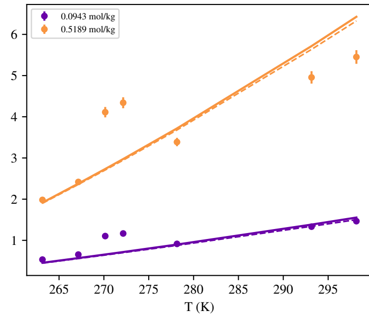
Na2CO3
