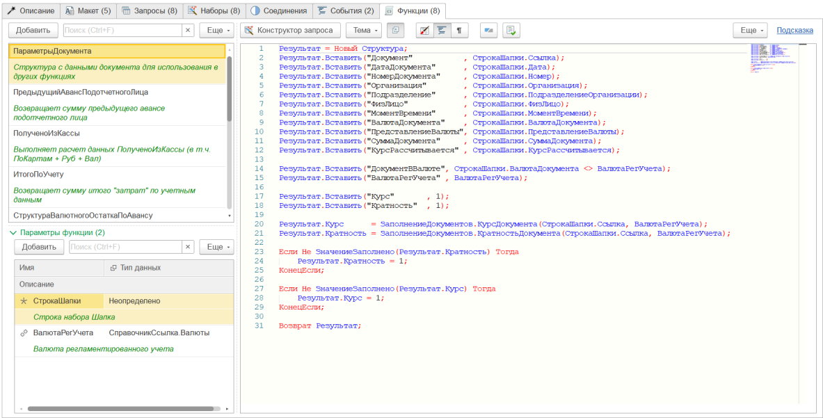
Рисунок 21. Закладка «Функции»
