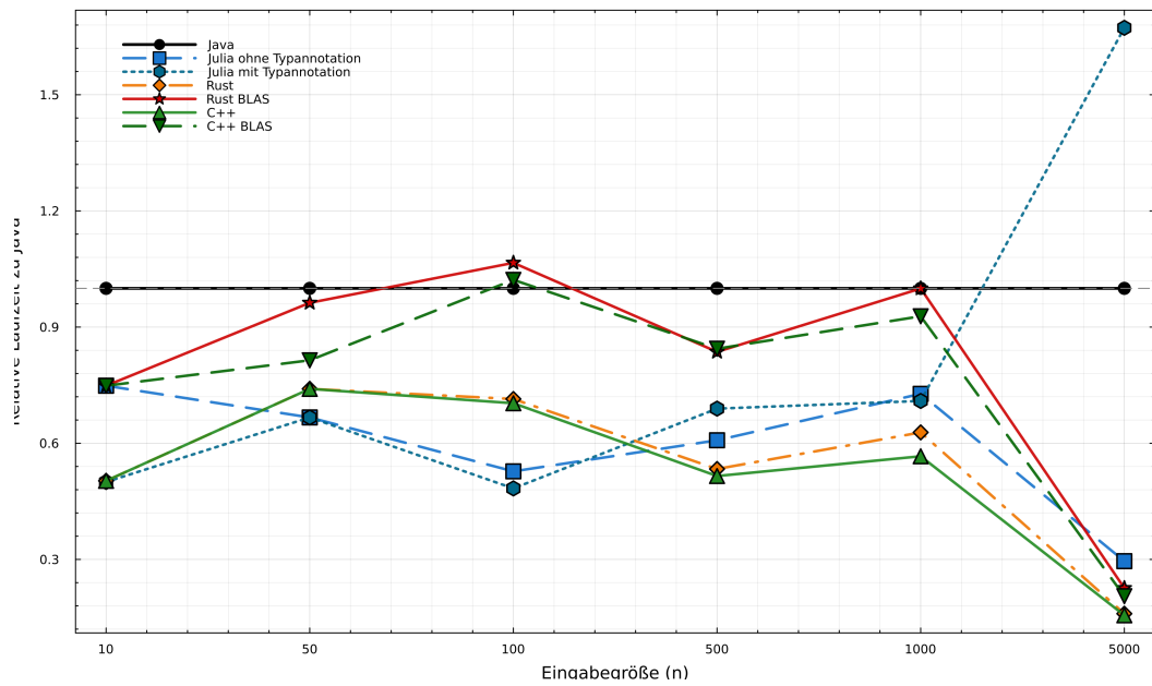
Abbildung 17: Relativer Laufzeit für Algorithmus 1
