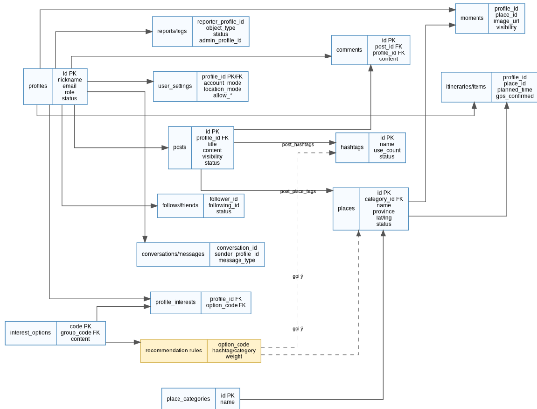
Hình 3.3. ERD mức khái quát theo cụm dữ liệu
