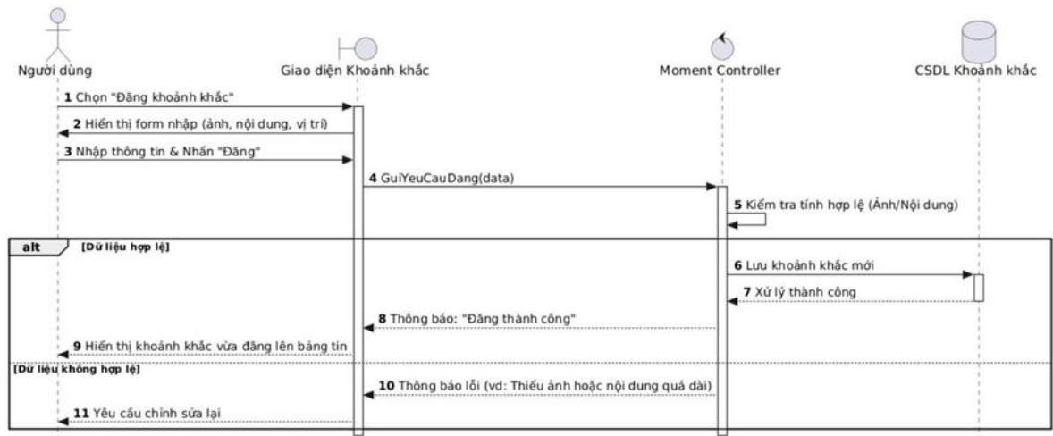
Hình 4.13. Sơ đồ tuần tự chức năng chia sẻ khoảnh khắc
