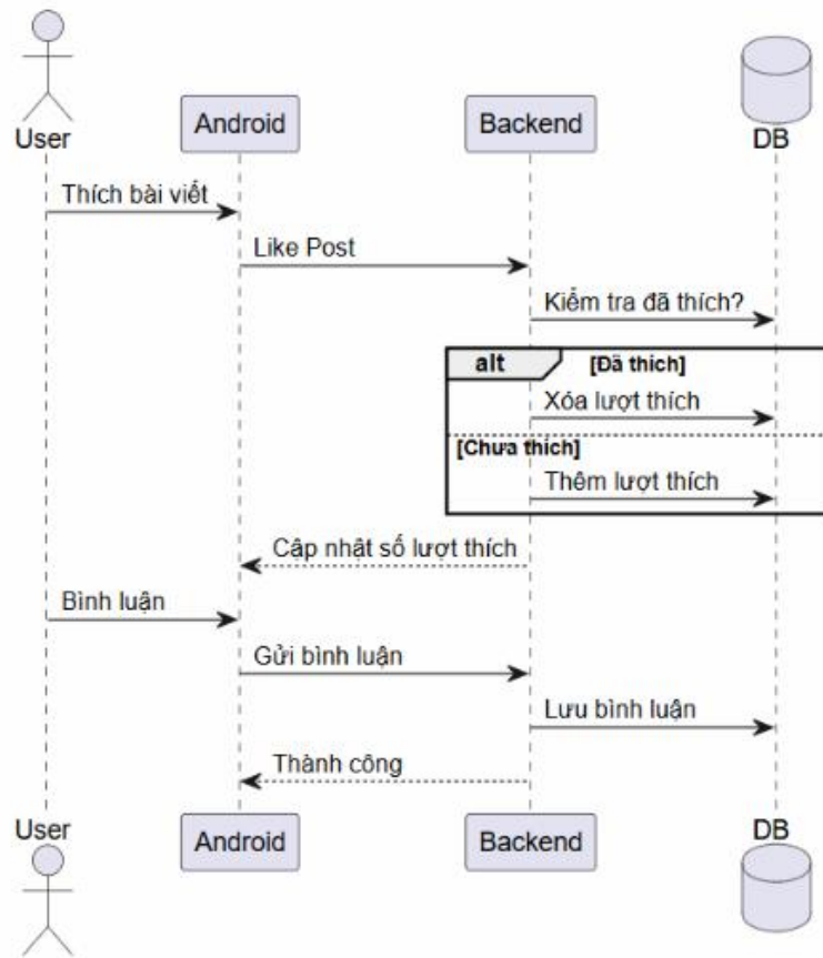
Hình 4.6. Sơ đồ tuần tự chức năng tương tác bài viết
