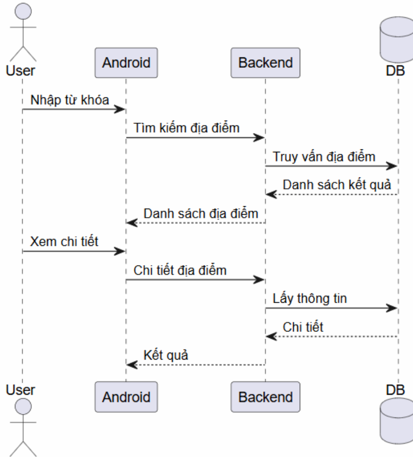
Hình 4.14. Sơ đồ tuần tự chức năng tìm kiếm địa điểm
