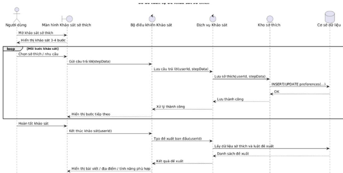
Hình 4.4. Sơ đồ tuần tự chức năng khảo sát sở thích
