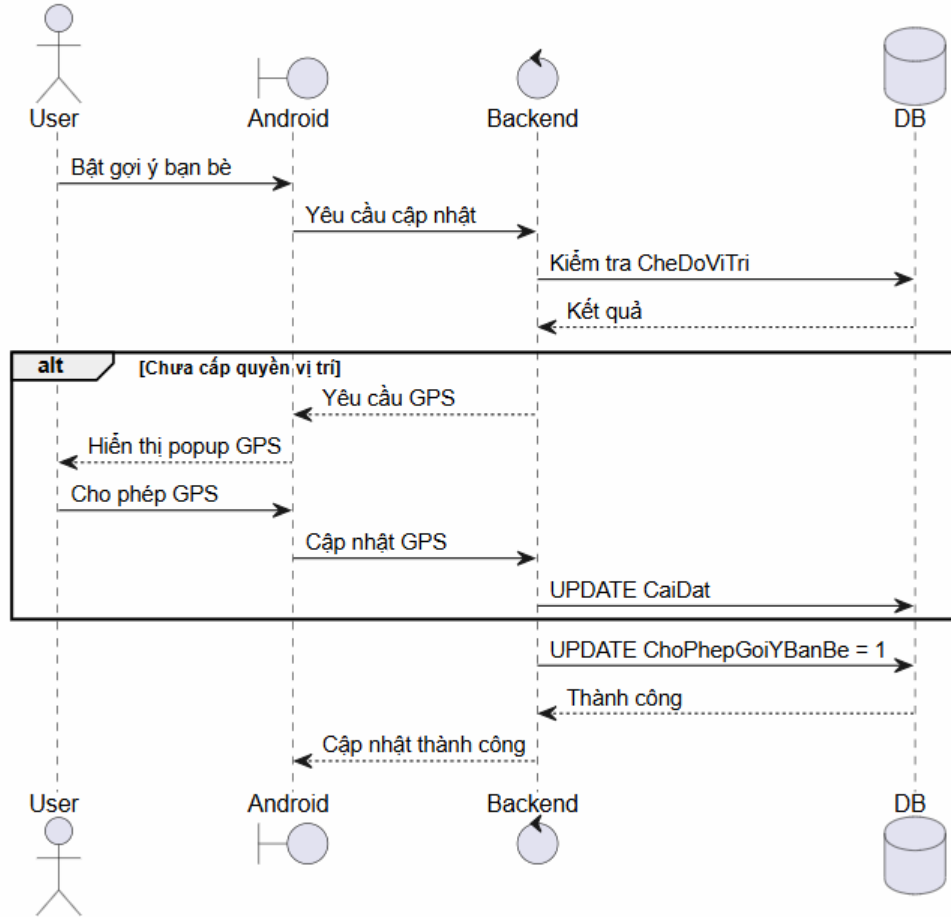
Hình 4.8. Sơ đồ tuần tự chức năng cài đặt gợi ý kết bạn
