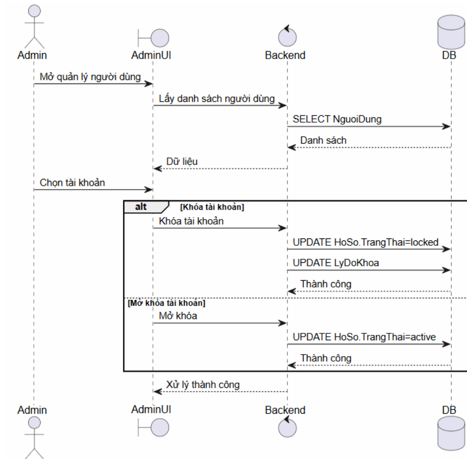
Hình 4.17. Sơ đồ tuần tự chức năng quản lý người dùng
