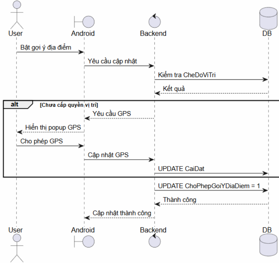
Hình 4.9. Sơ đồ tuần tự chức năng cài đặt gợi ý địa điểm
