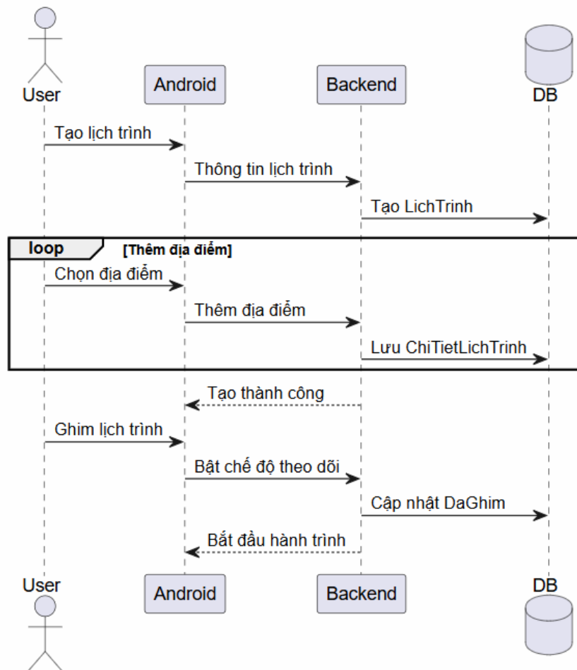
Hình 4.15. Sơ đồ tuần tự chức năng tạo lịch trình
