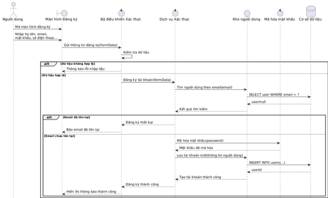
Hình 4.2. Sơ đồ tuần tự chức năng đăng kí
