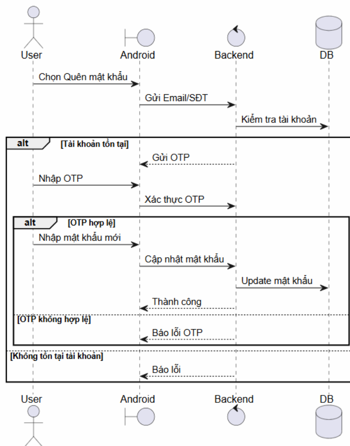
Hình 4.3. Sơ đồ tuần tự chức năng quên mật khẩu
