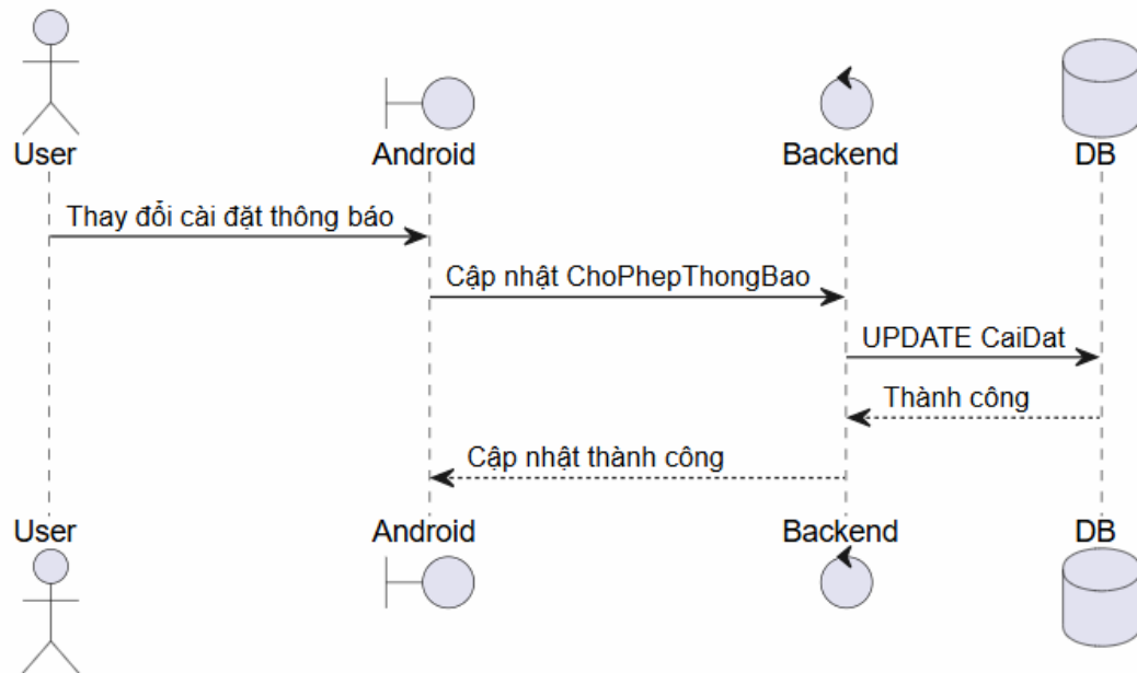
Hình 4.10. Sơ đồ tuần tự chức năng cài đặt thông báo
