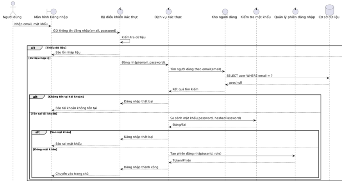
Hình 4.1. Sơ đồ tuần tự chức năng đăng nhập
