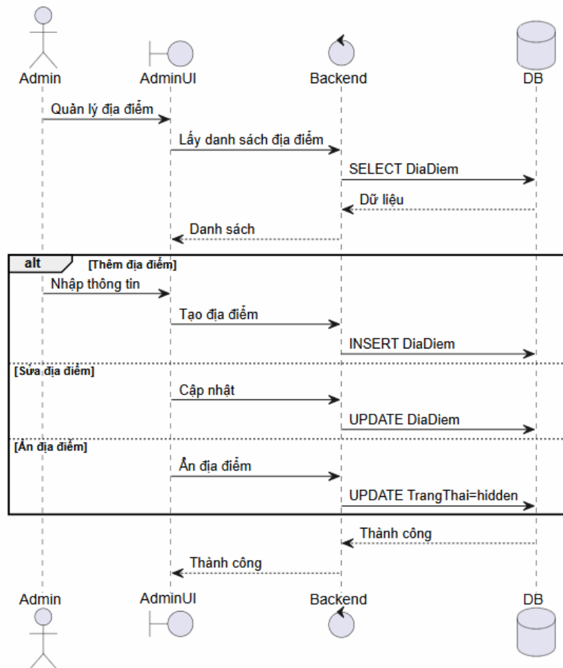
Hình 4.18. Sơ đồ tuần tự chức năng quản lý địa điểm
