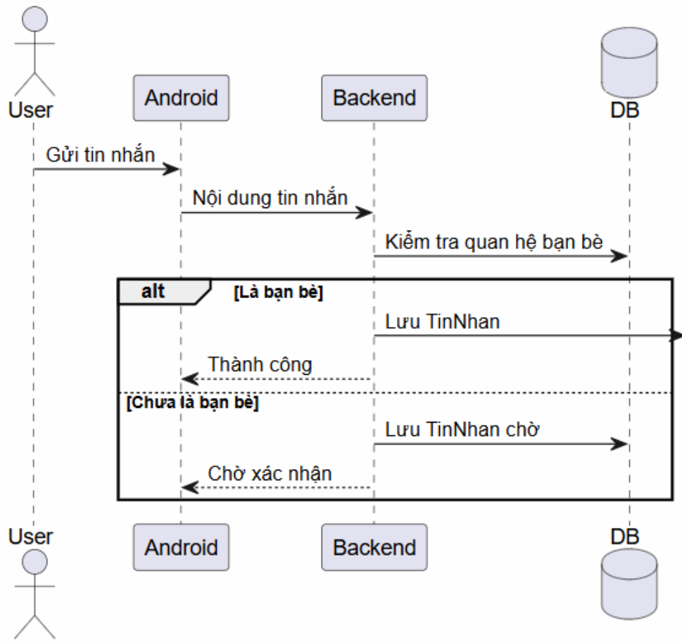
Hình 4.12. Sơ đồ tuần tự chức năng tin nhắn
