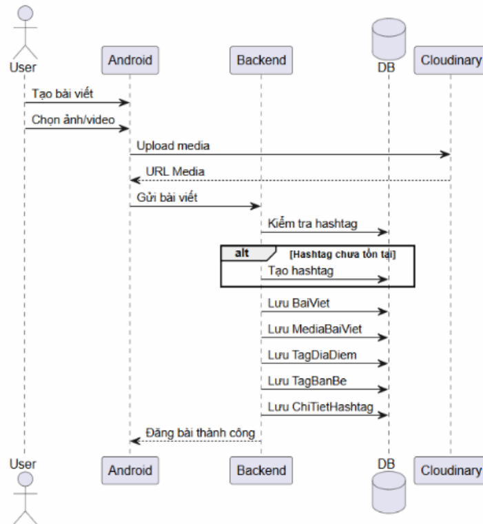
Hình 4.5. Sơ đồ tuần tự chức năng đăng bài viết
