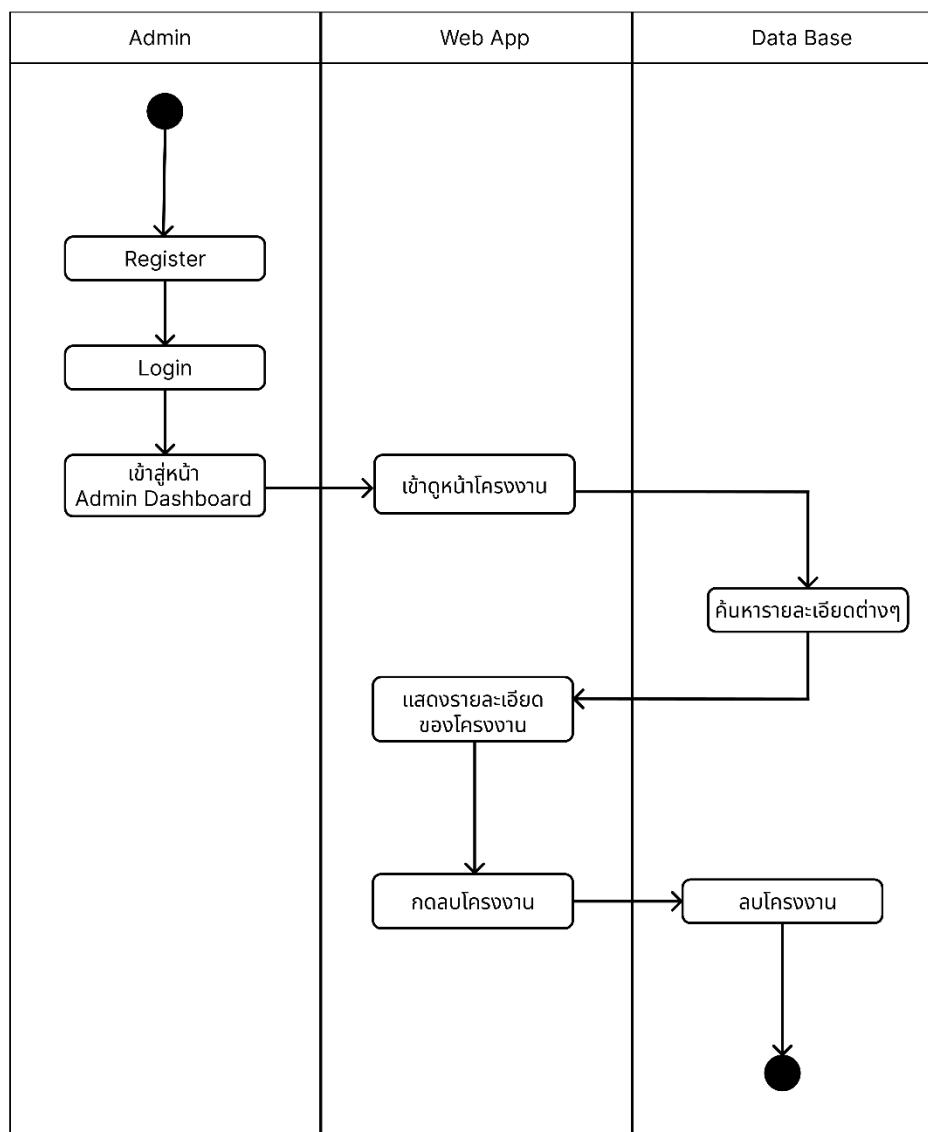
ภาพที่ 21 แผนภาพกิจกรรมของการลบโครงการ
