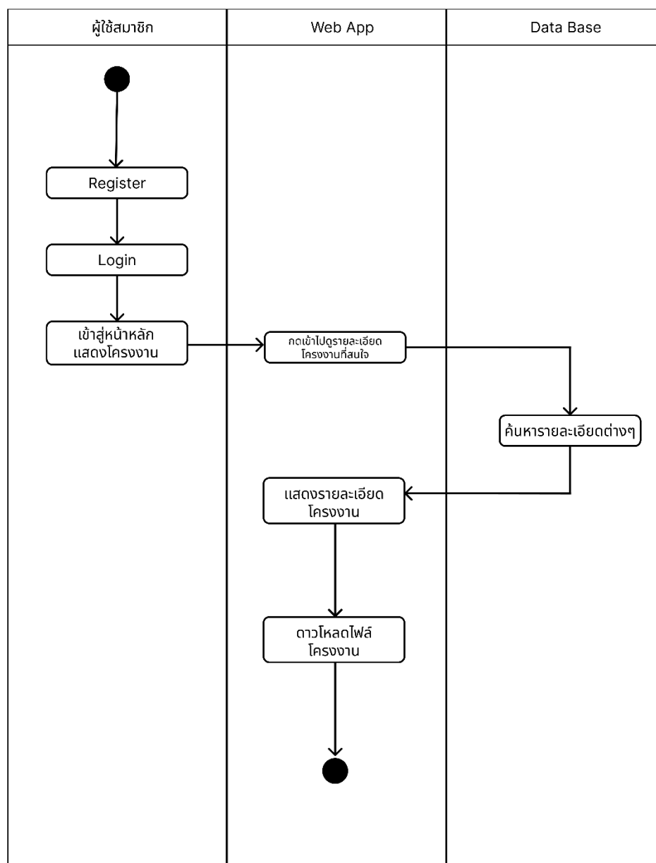
ภาพที่ 12 แผนภาพกิจกรรมของการดาวน์โหลดเอกสาร
