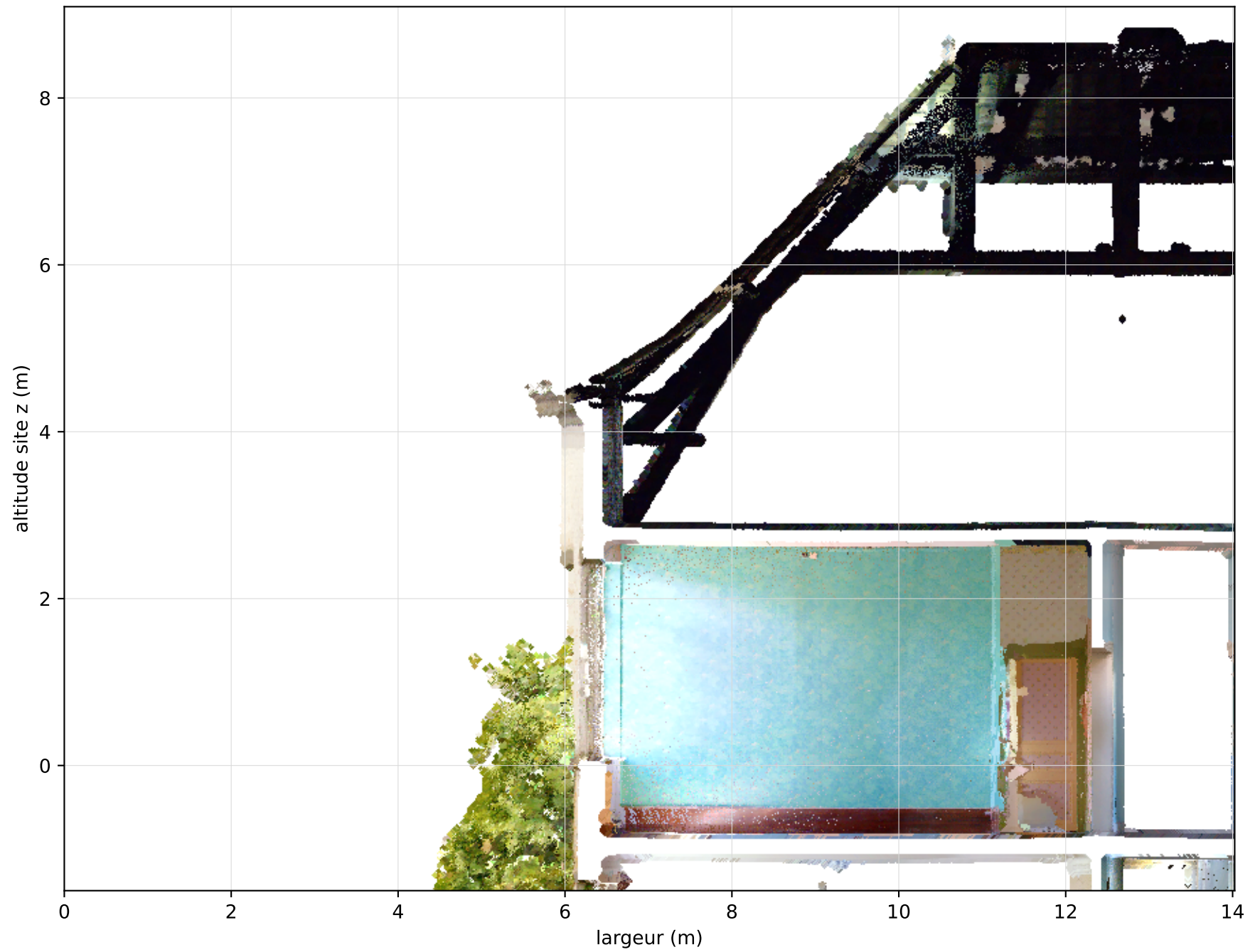
Aile Ouest — façade sud · 14.0 m · couverture 28 %
