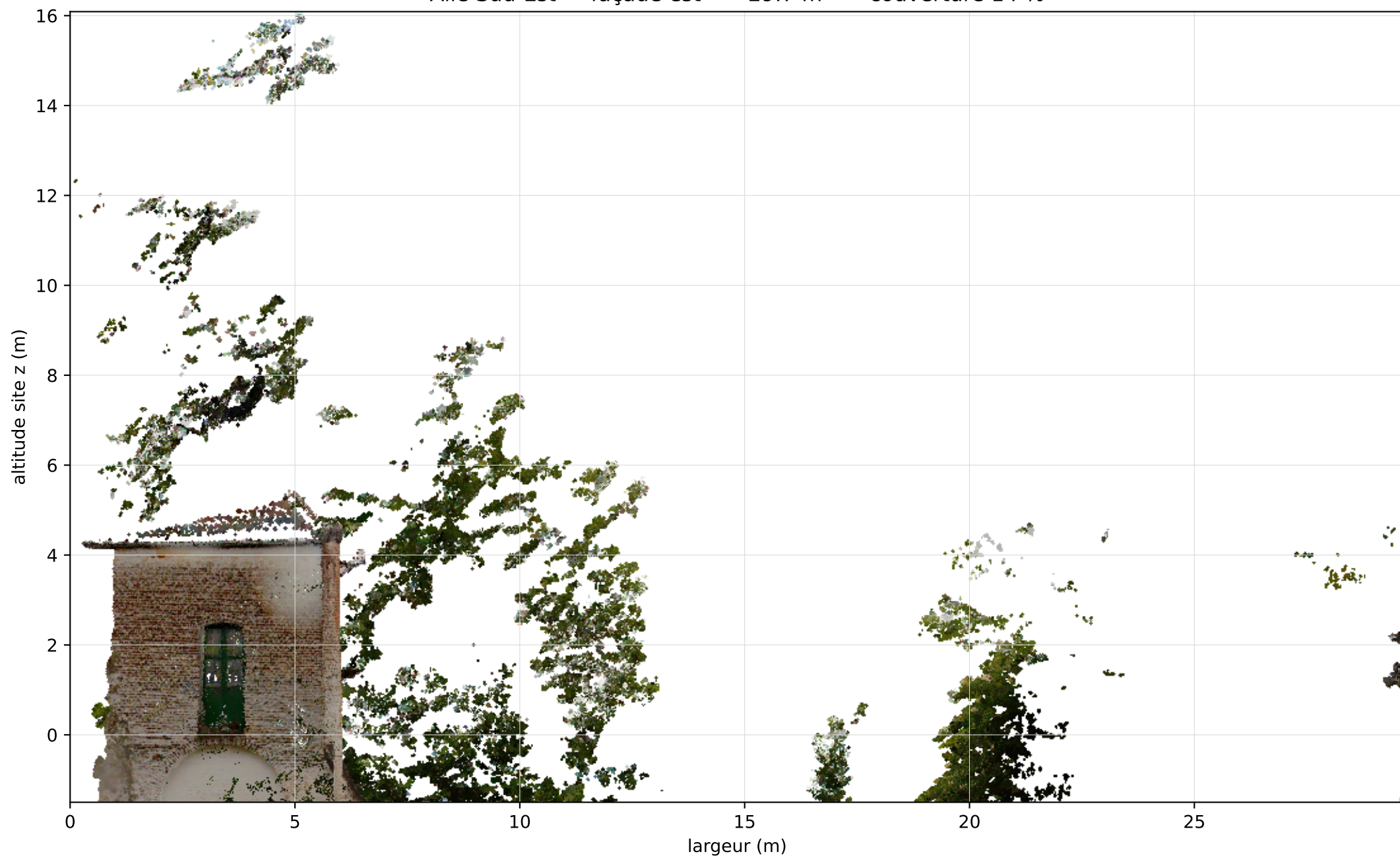
Aile Sud-Est — façade est · 29.7 m · couverture 14 %
