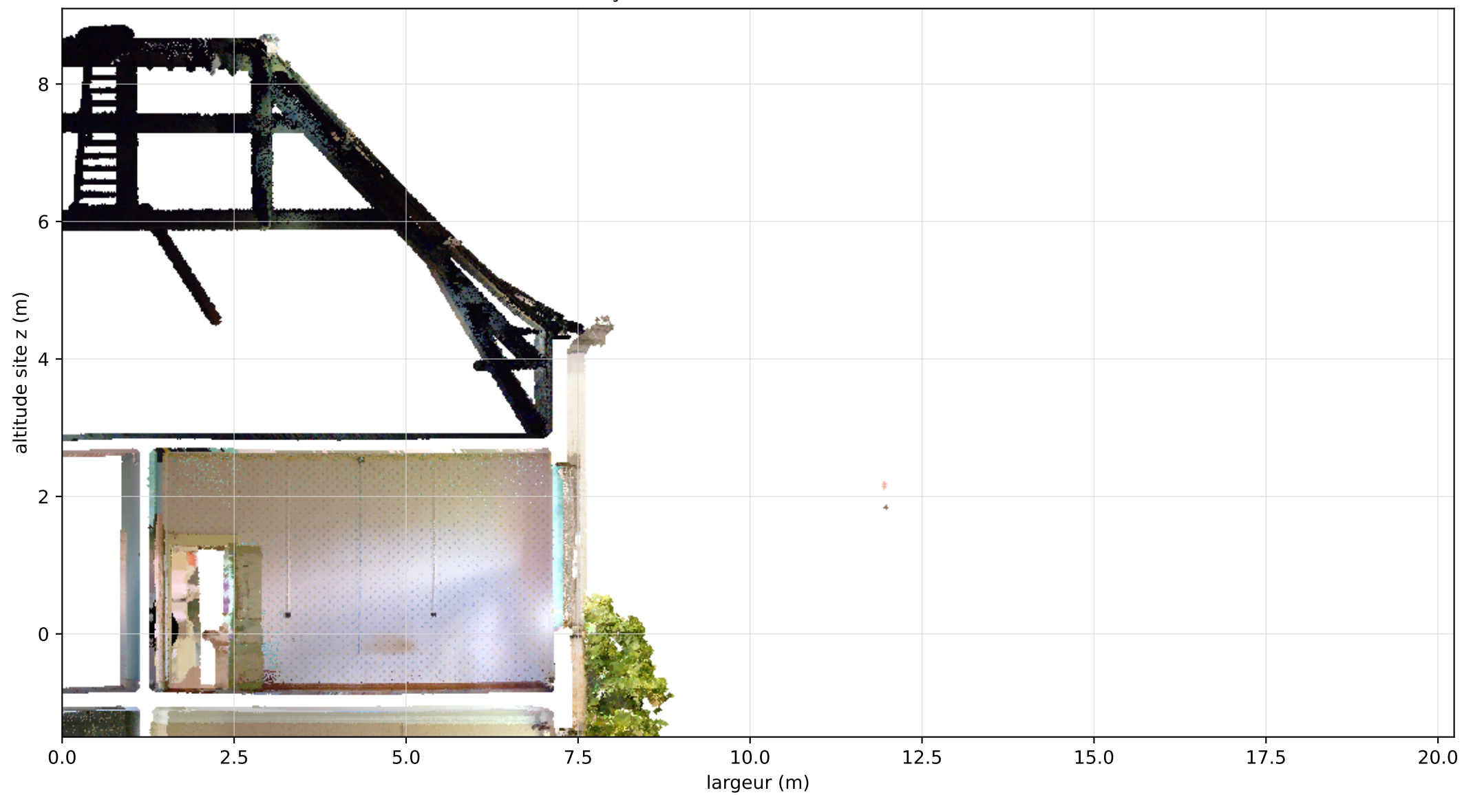
Aile Ouest — façade nord · 20.2 m · couverture 18 %
