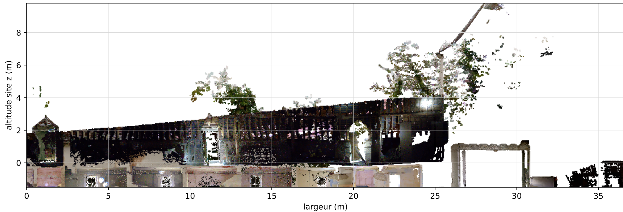
Aile Sud-Est — façade sud · 36.6 m · couverture 33 %
