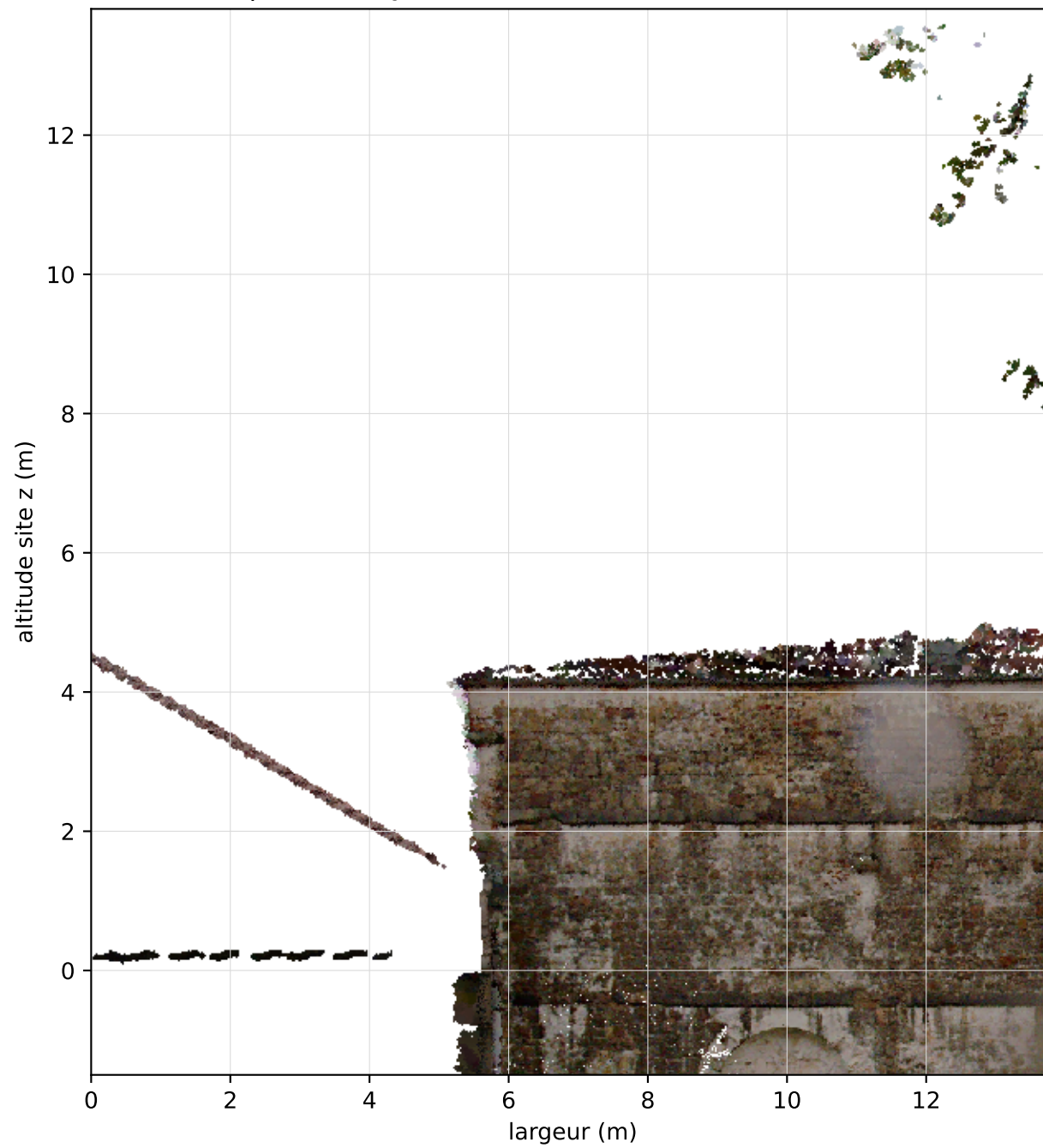
Chapelle — façade est · 13.8 m · couverture 25 %
