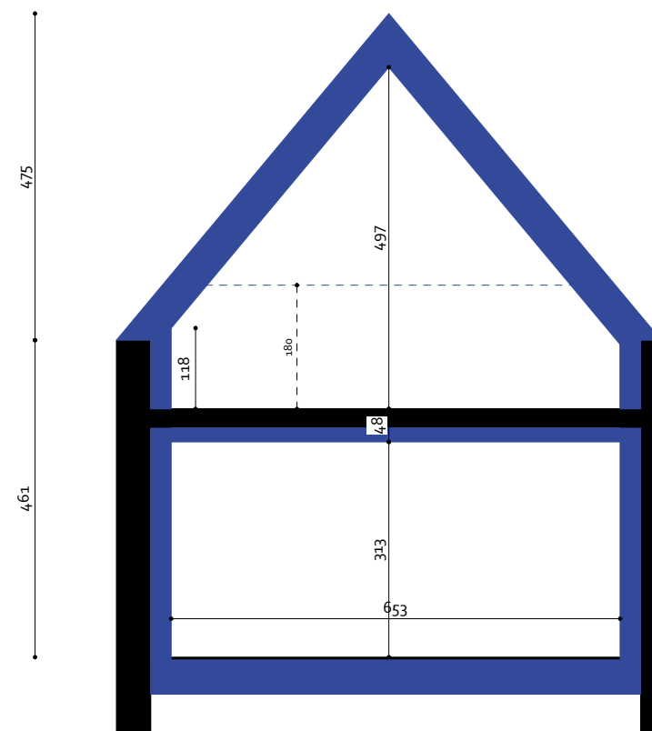
coupes grange est L7/L8
