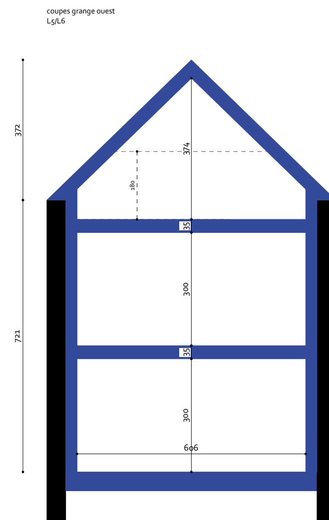
coupes granges ouest
