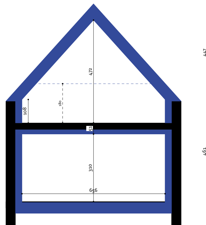
coupes grange sud L9/atelier construction
