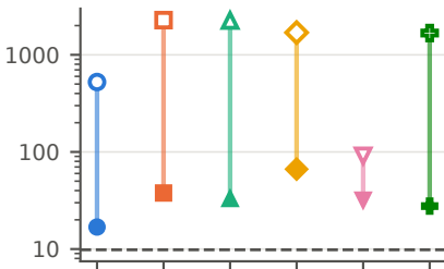
Llama-3.2-1B
