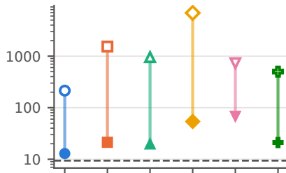
Qwen3-1.7B
