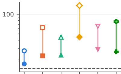
OPT-1.3B
