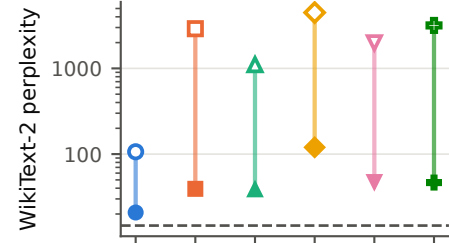
OPT-1.3B
