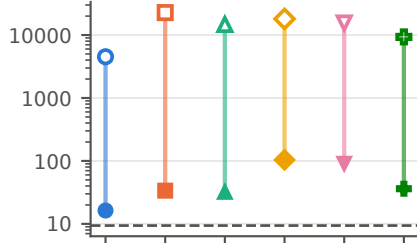
Qwen3-1.7B
