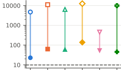
Llama-3.2-1B
