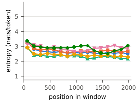
OPT-1.3B
