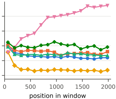
Llama-3.2-1B
