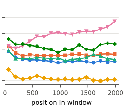
Qwen3-1.7B
