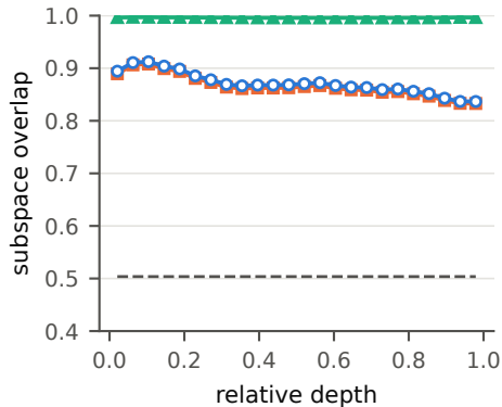
OPT-1.3B
