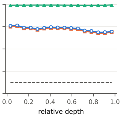
Llama-3.2-1B
