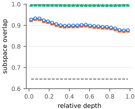
OPT-1.3B
