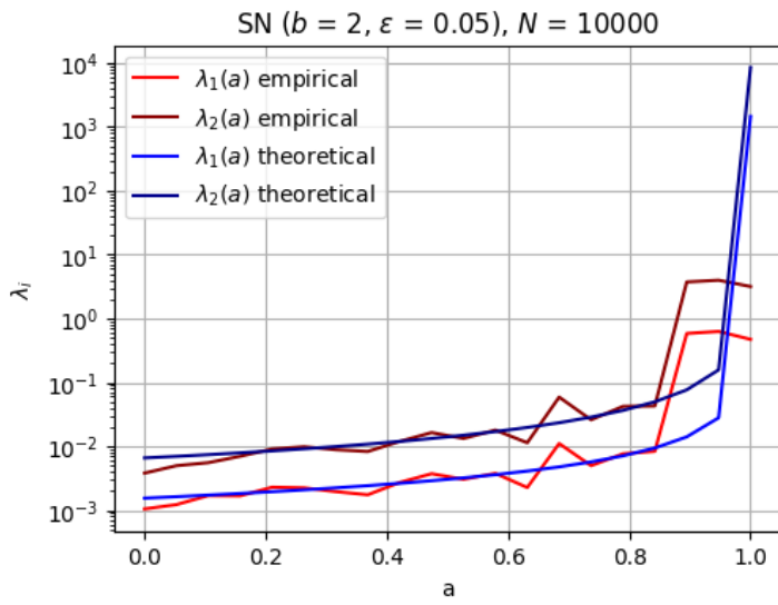
Рис. 31: Сравнение собственных значений матрицы ковариации и матрицы стохастической чувствительности для модели SN
