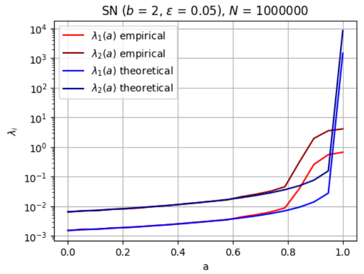
Рис. 31: Сравнение собственных значений матрицы ковариации и матрицы стохастической чувствительности для модели SN
