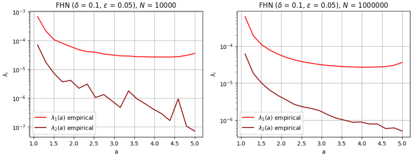
Рис. 26: Собственные значения матрицы ковариации для модели FHN
