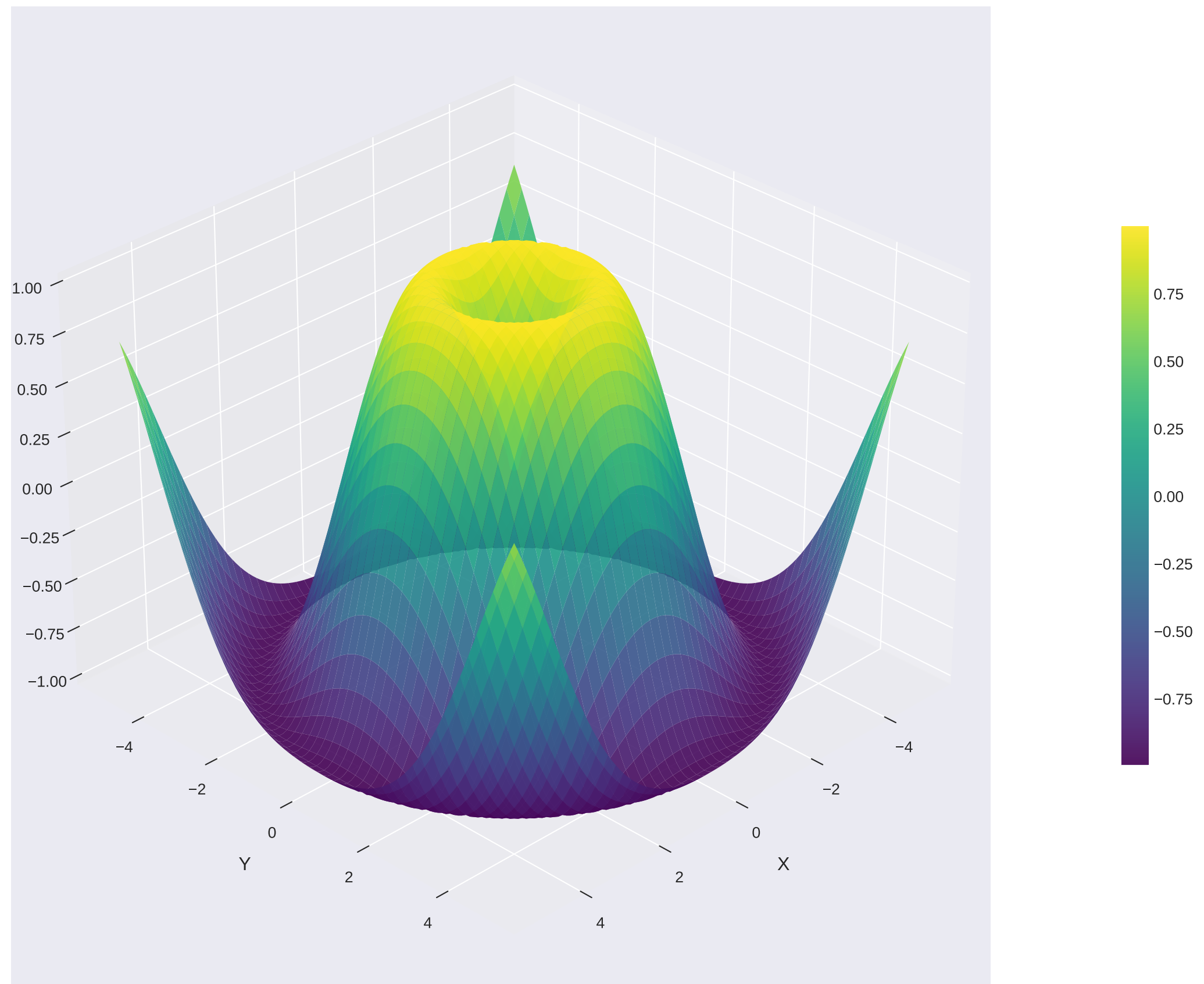
3D поверхность: z = \sin(\sqrt{x^2 + y^2})
