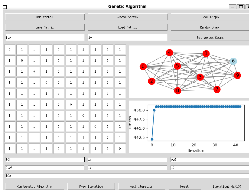
Рисунок 1 – Графический интерфейс программы
