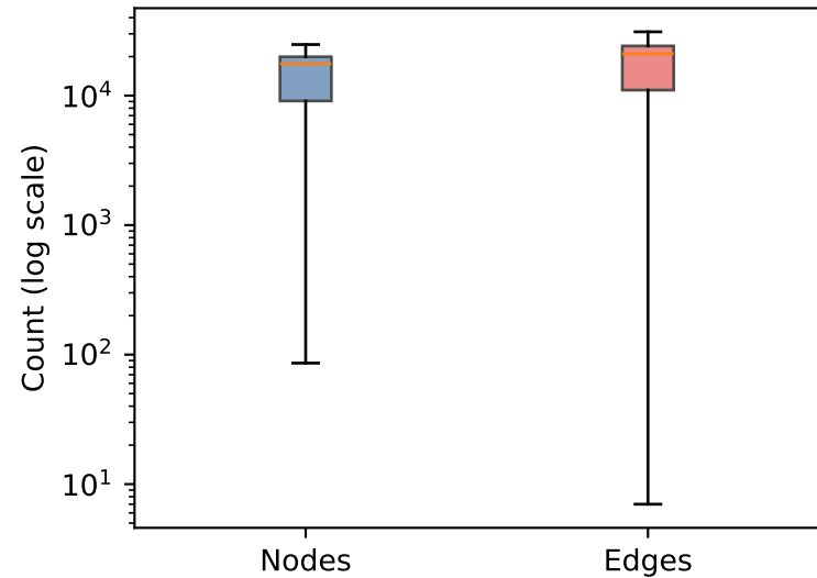
Benign
