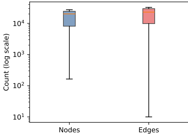
Malware
