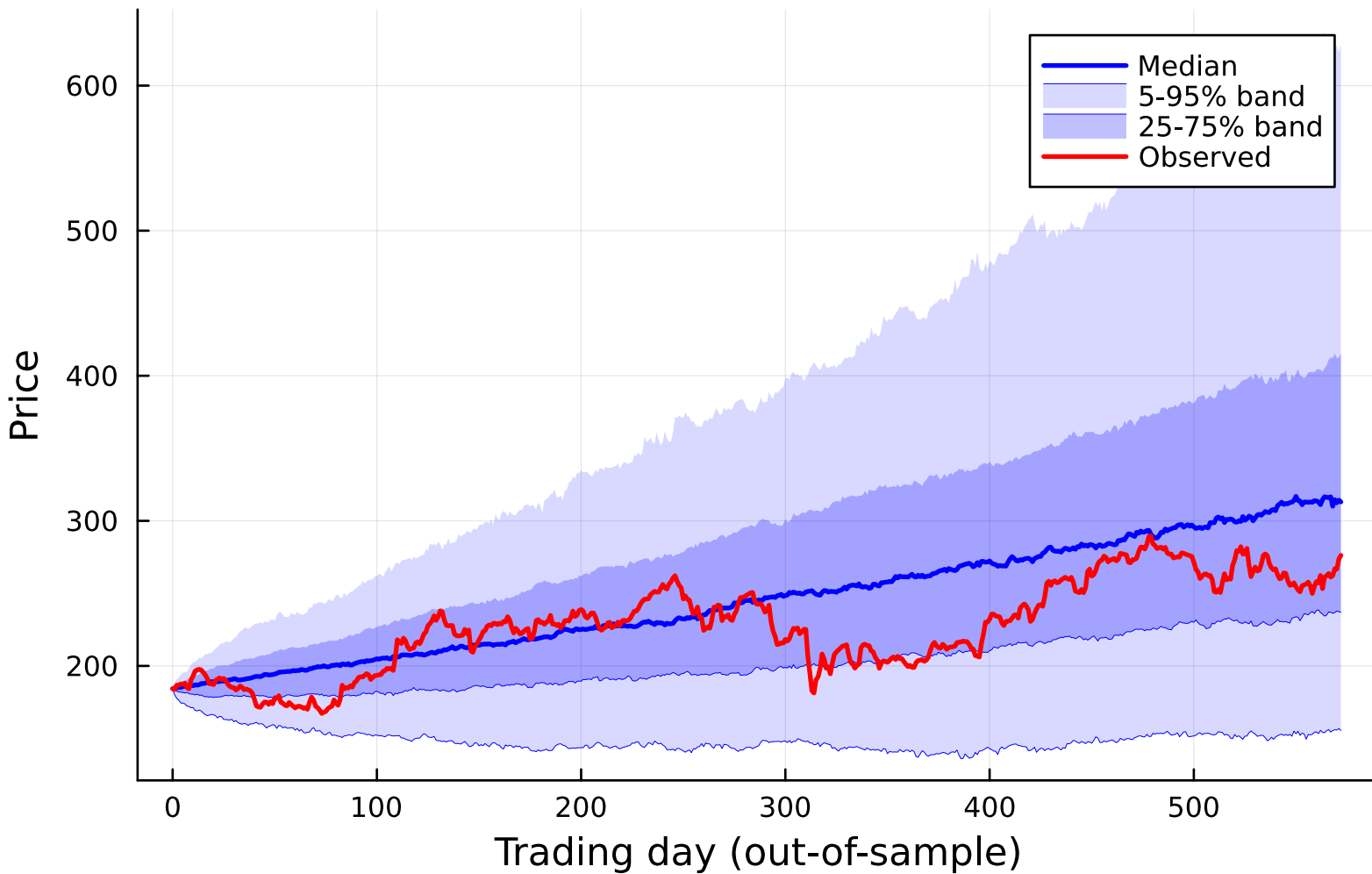
AAPL - CHMM-N price fan (K=18, 500 paths)
