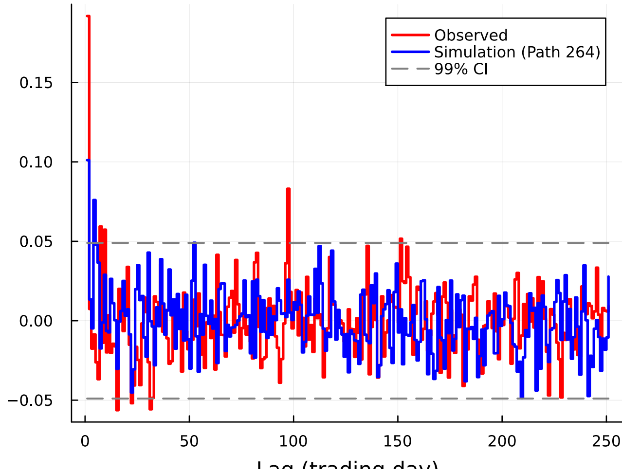
Returns ACF — K=18
