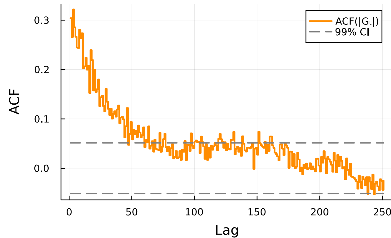
(d) Volatility Clustering
