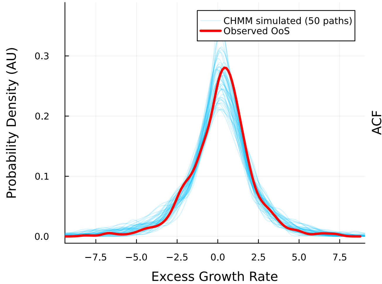
(b) OoS Density Fan
