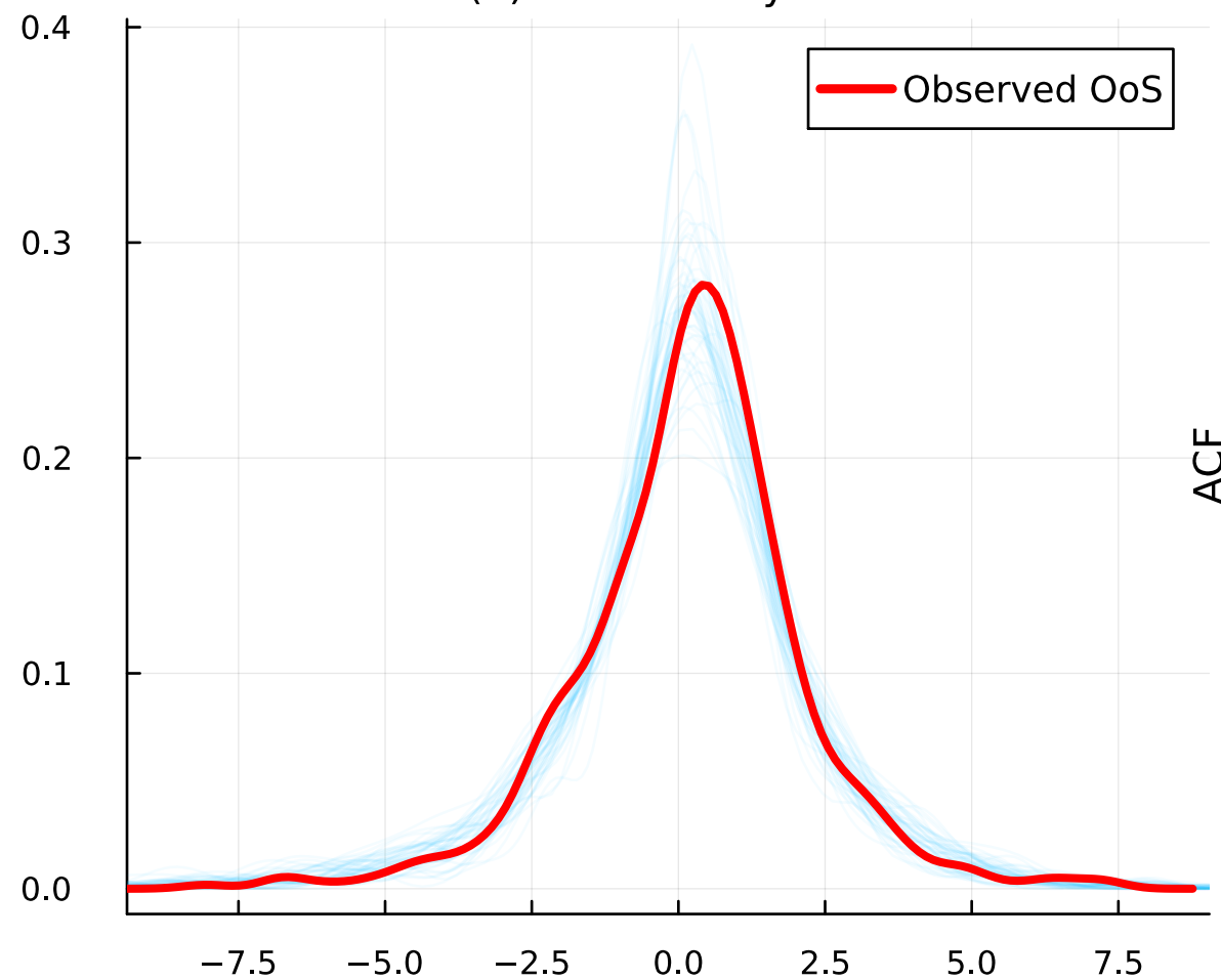
(b) OoS Density Fan
