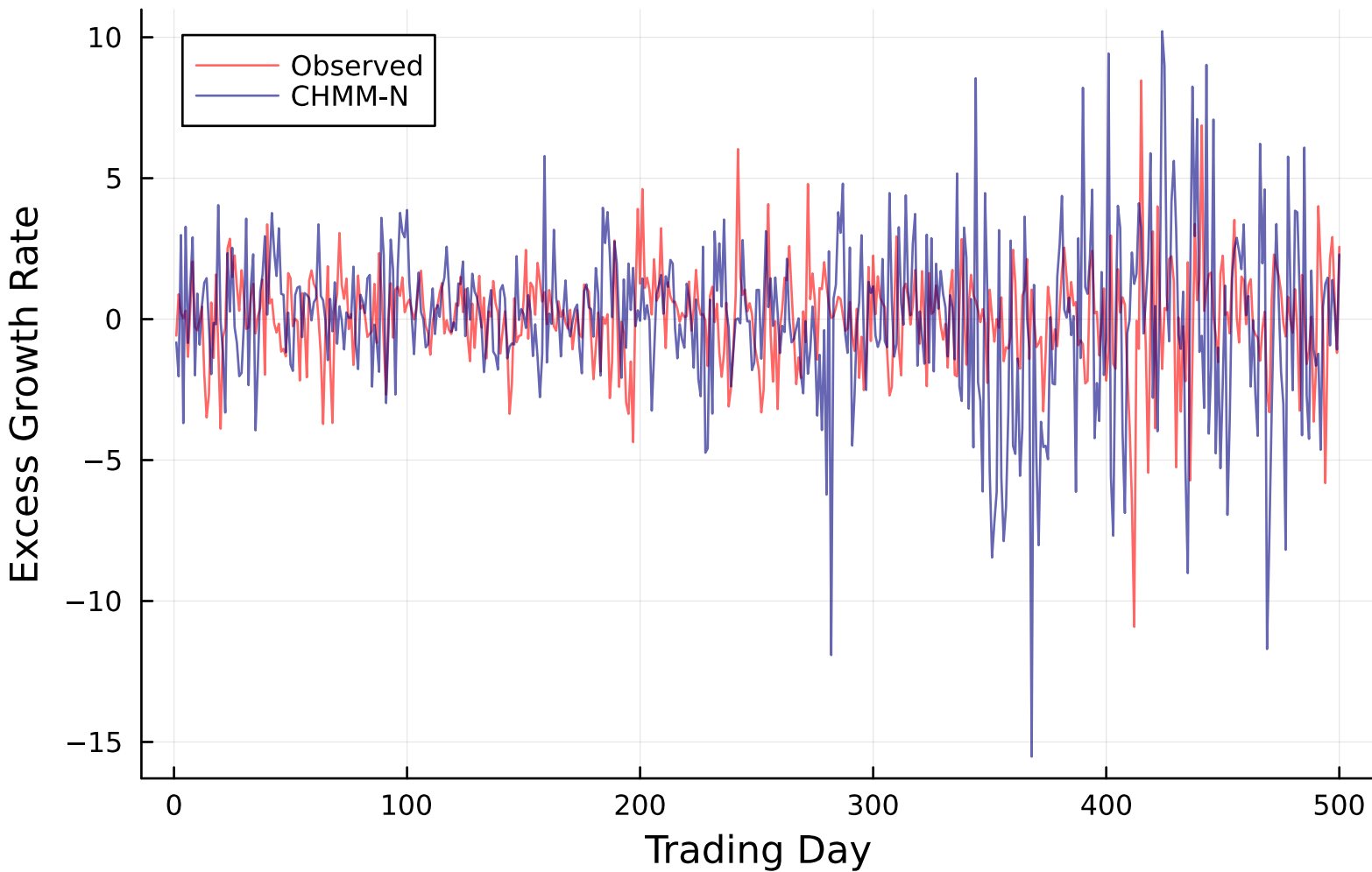
Return Trajectory (CHMM-N, K=18)
