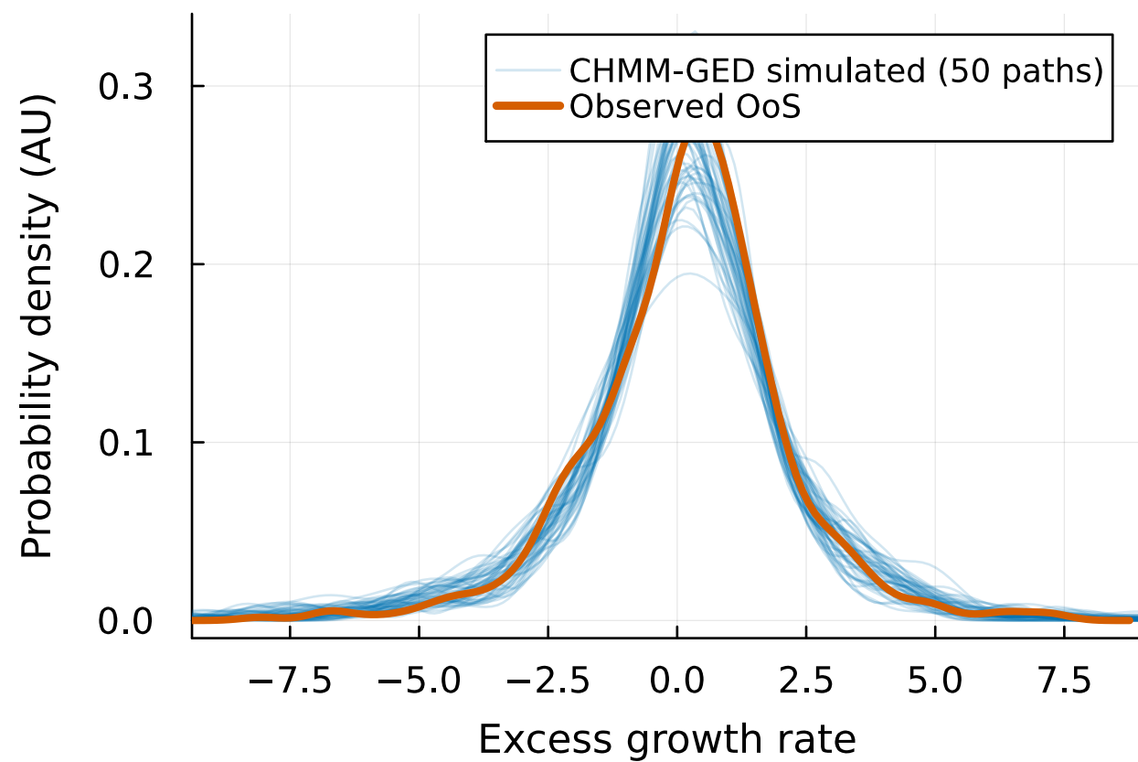
OoS density fan
