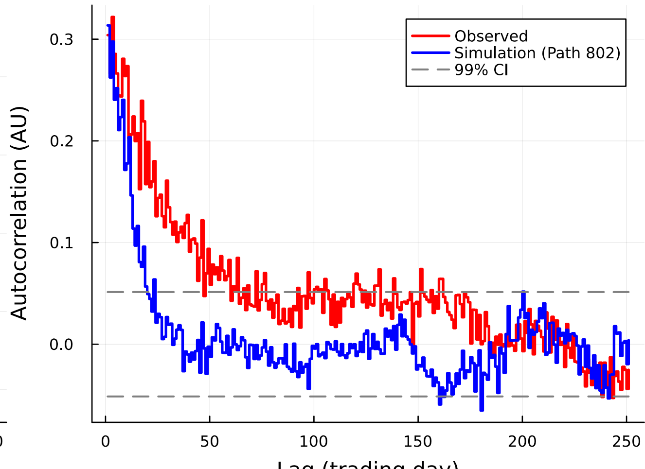
|Returns| ACF — K=18
