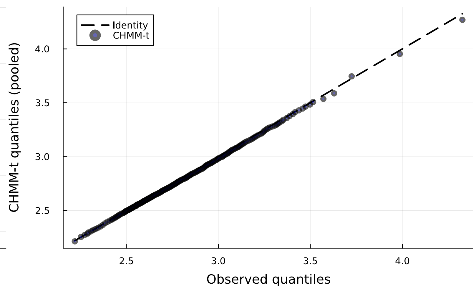
(d) Q-Q plot of log(VIX) levels
