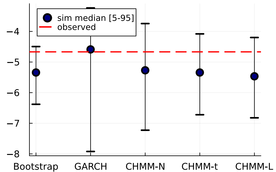
OoS ES (0.05)
