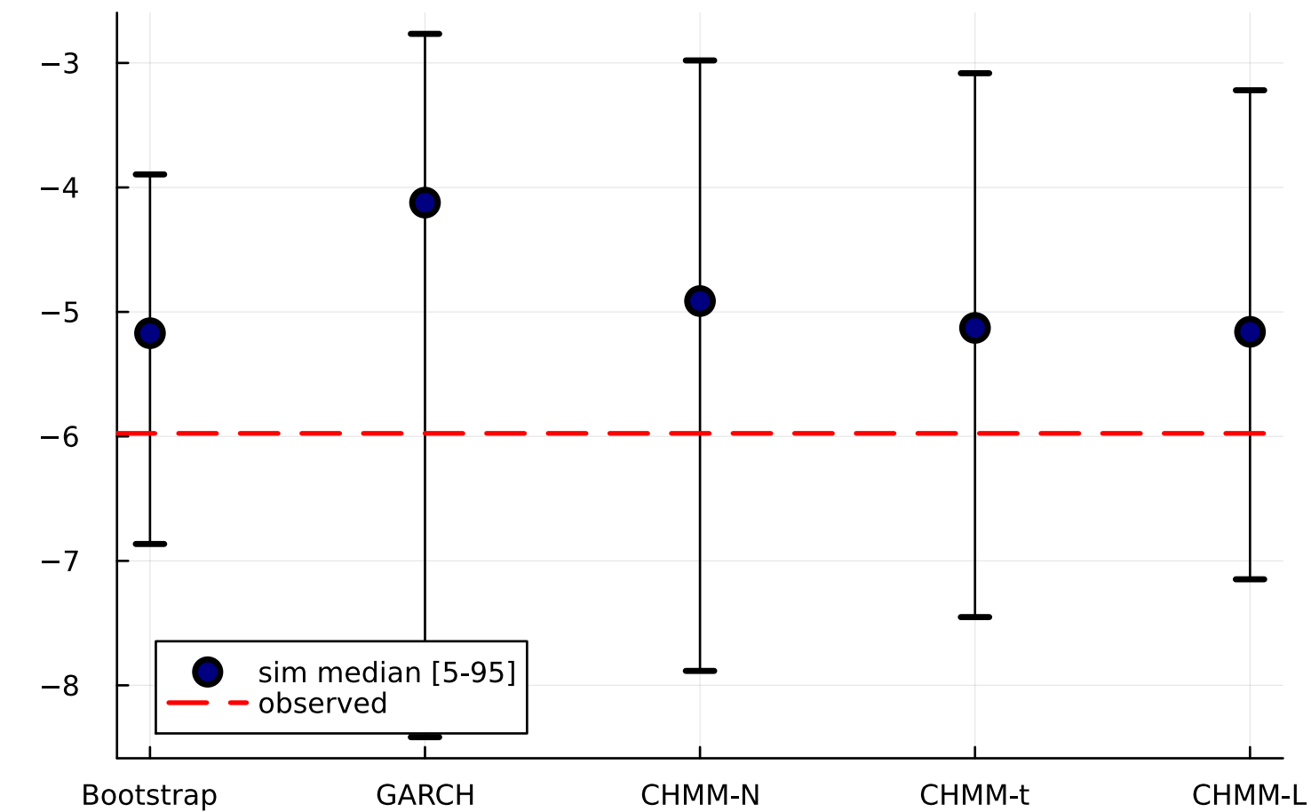
OoS ES (0.05)
