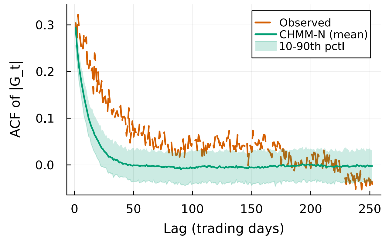
(d) ACF of |G_t|
