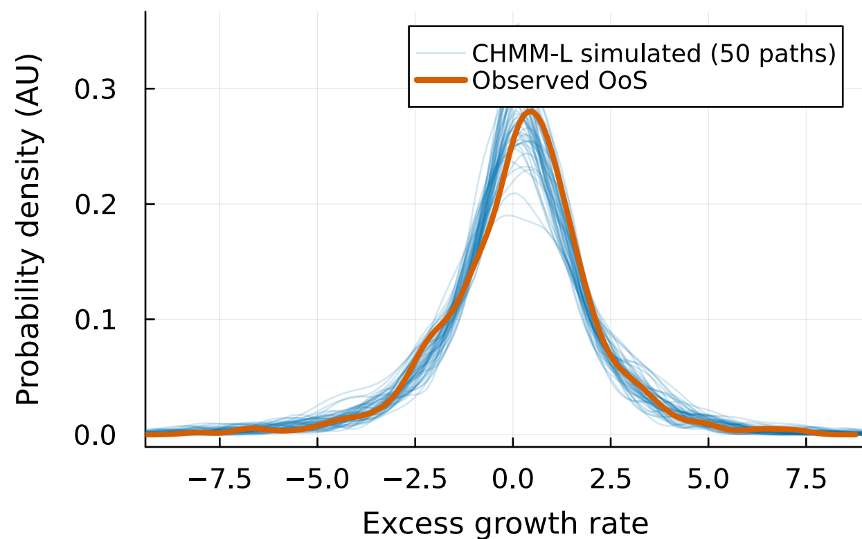
(a) OoS density fan
