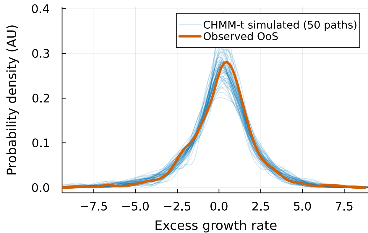
(a) OoS density fan
