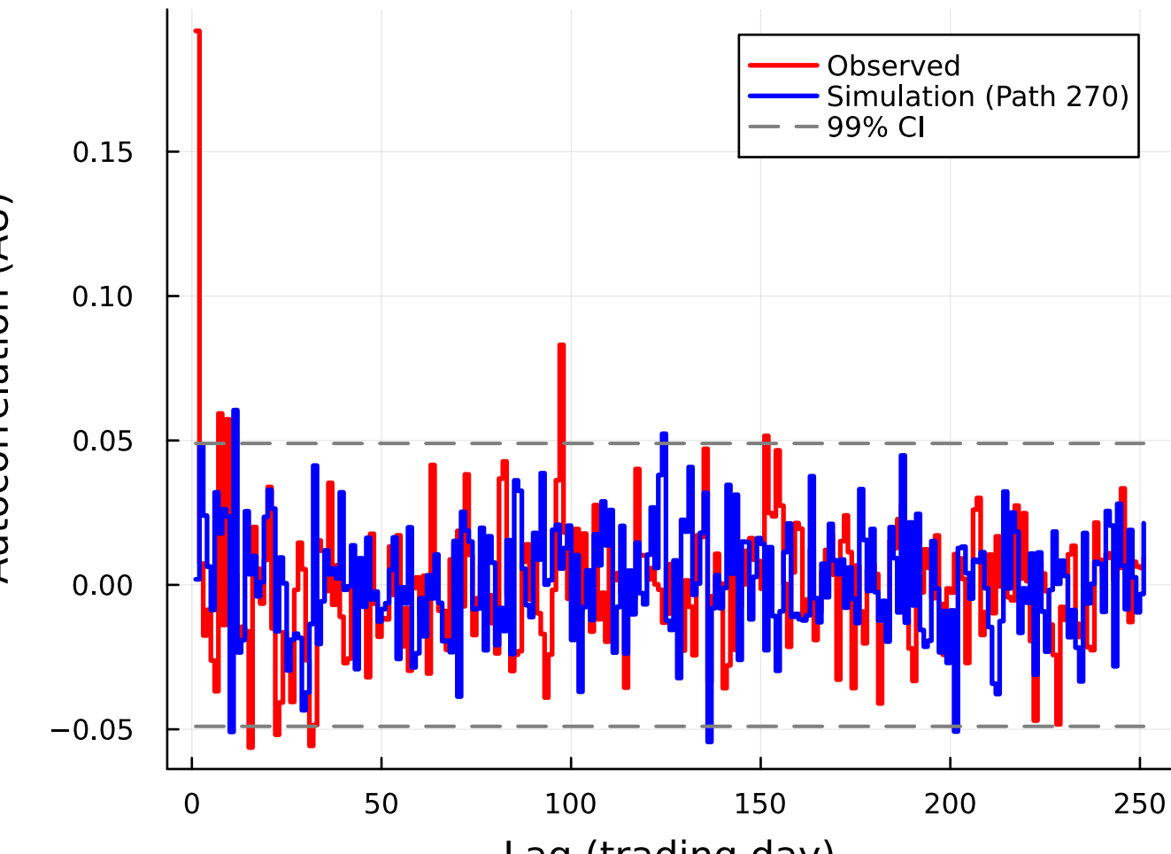
Returns ACF — K=3
