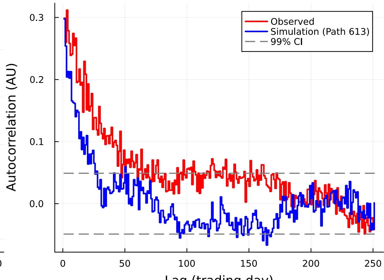
|Returns| ACF — K=6
