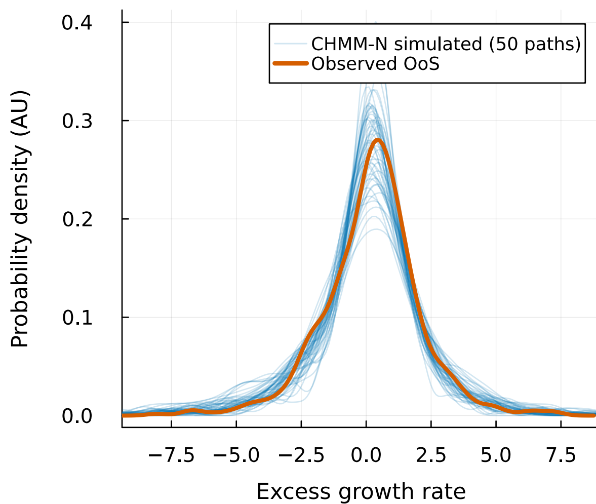
(b) OoS density fan
