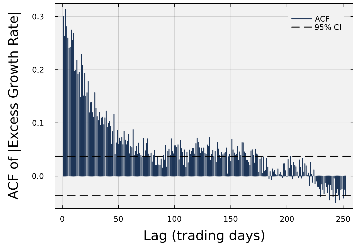
(d) ACF of |Excess Growth Rates|
