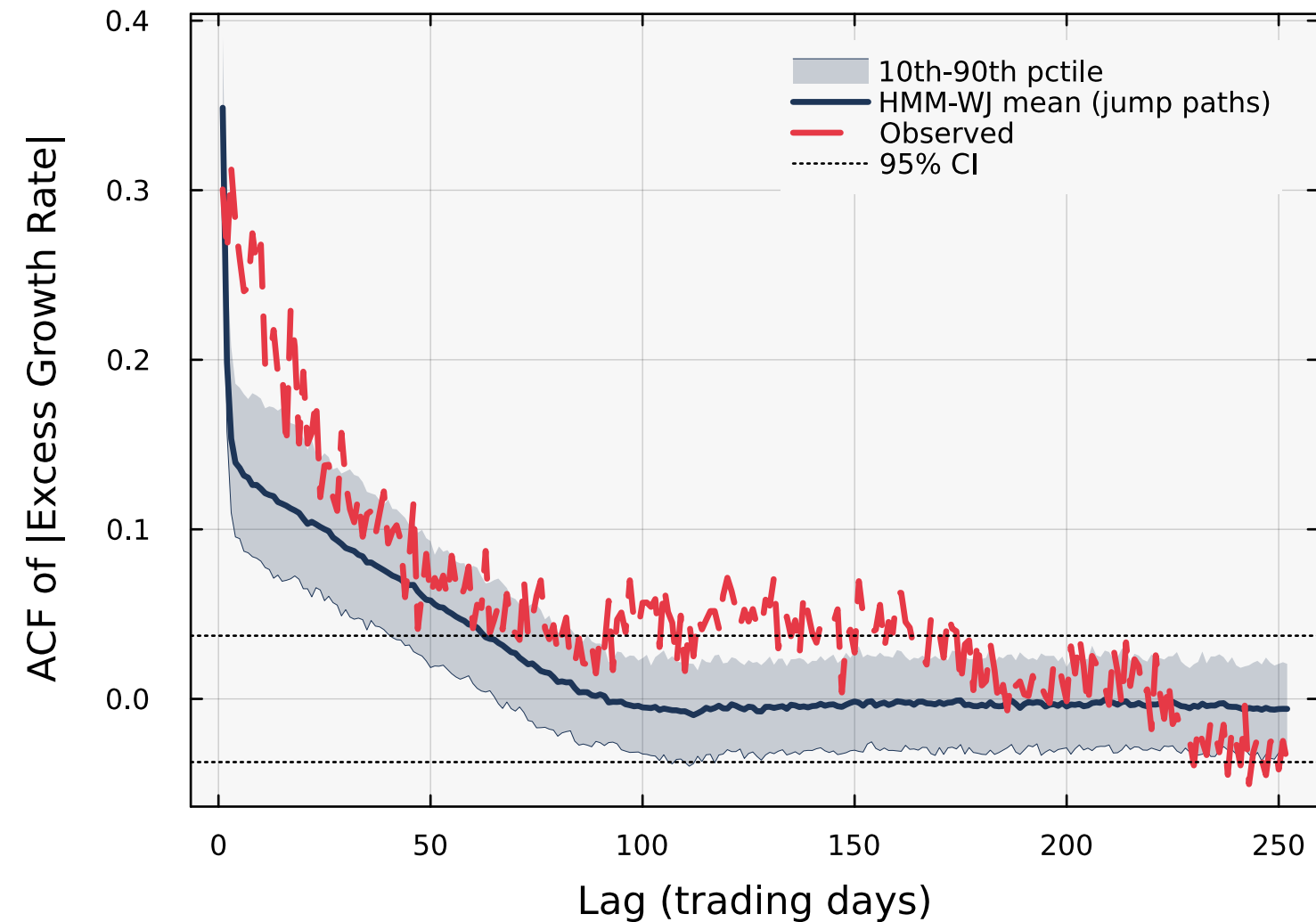
(d) IS Volatility Clustering (jump paths)
