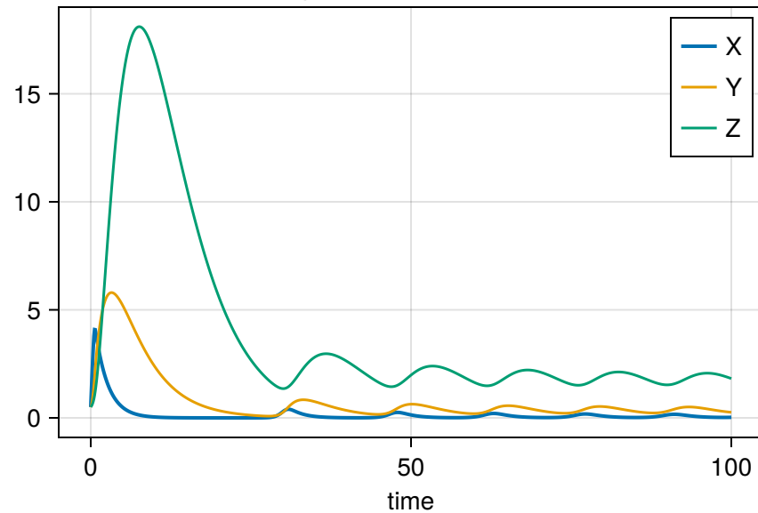
(D) Negative-feedback oscillator
