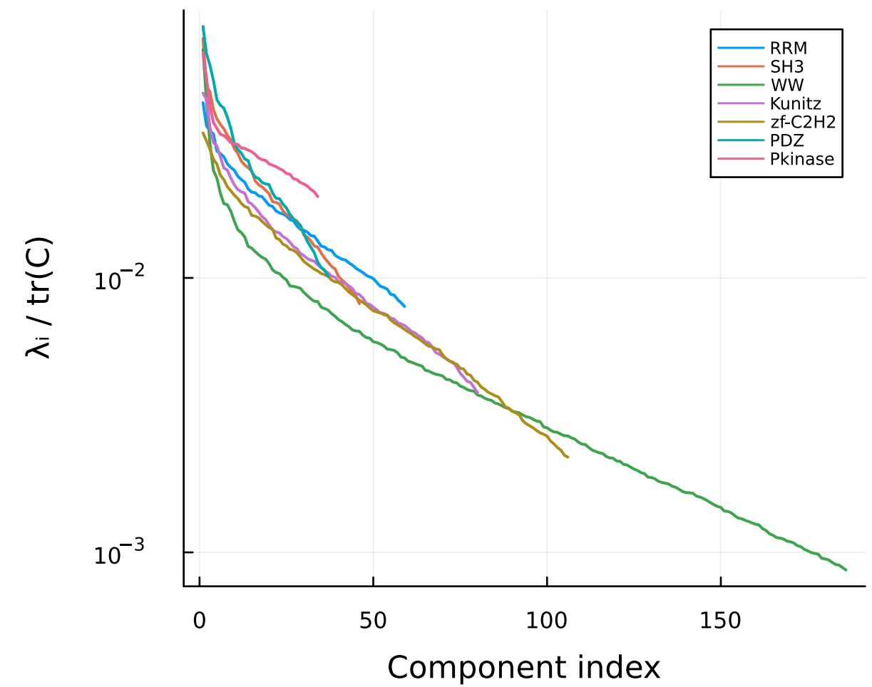
(F) Eigenvalue Spectra (Pfam)
