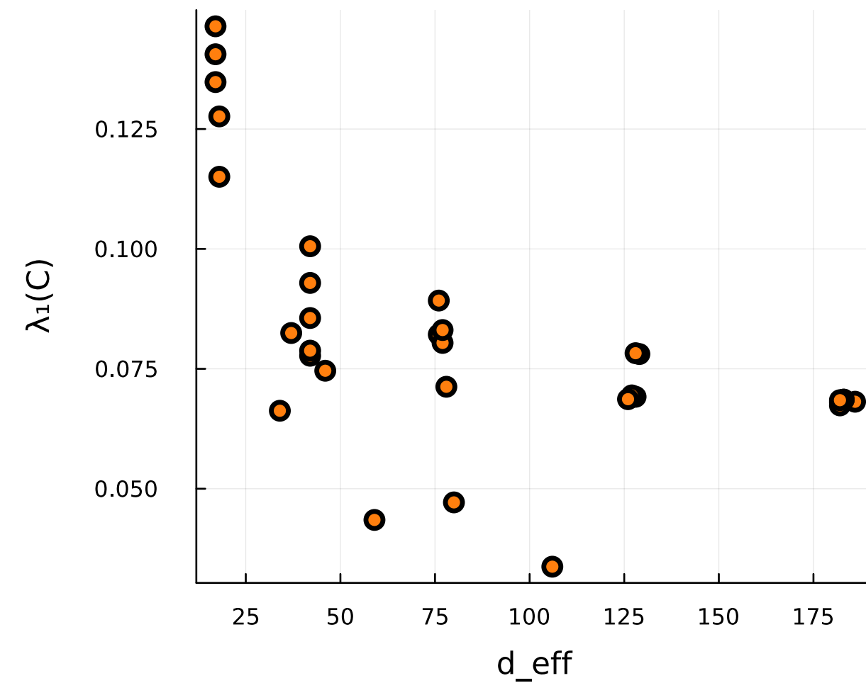
(D) Leading Eigenvalue vs d\_eff
