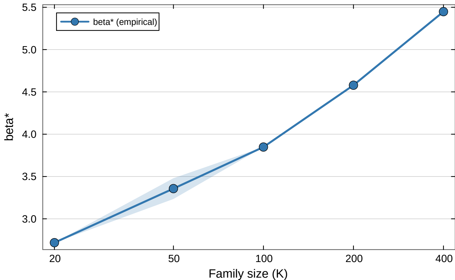
(D) Critical temperature
